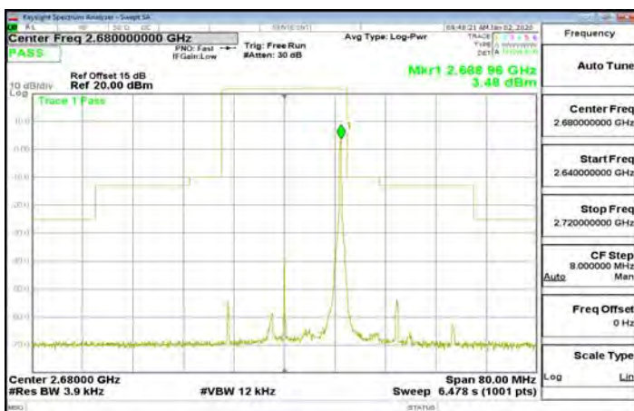
Band41_20MHz_QPSK_1_99_CH41490
