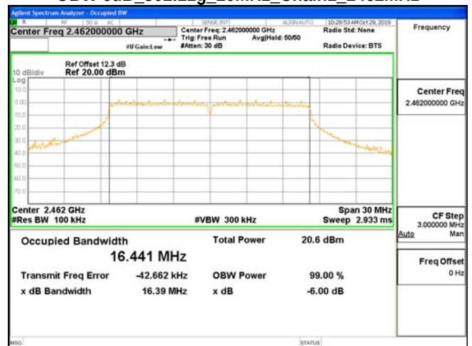
OBW 6dB_802.11g_20MHz_Chain1_2462MHz
