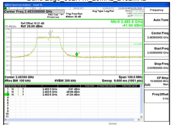
Band Edge 802.11n 20MHz 2462MHz
