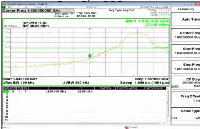
LTE\Band2 10MHz QPSK 1 0 LowCH18650-1855
