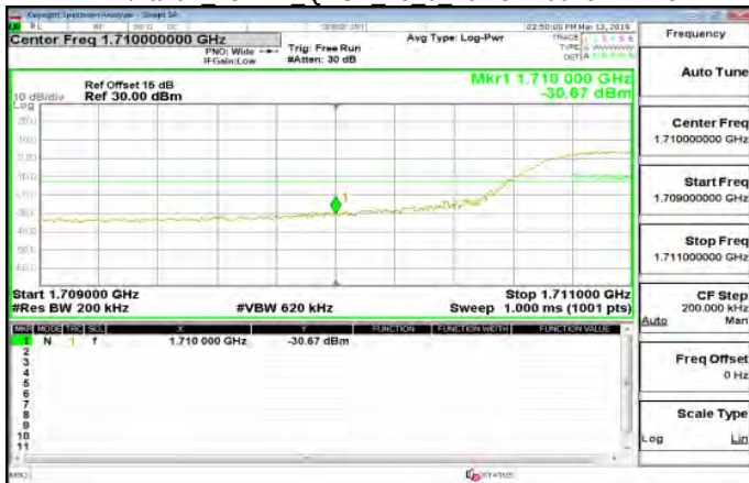
LTE\Band4 15MHz QPSK 75 0 LowCH20025-1717.5
