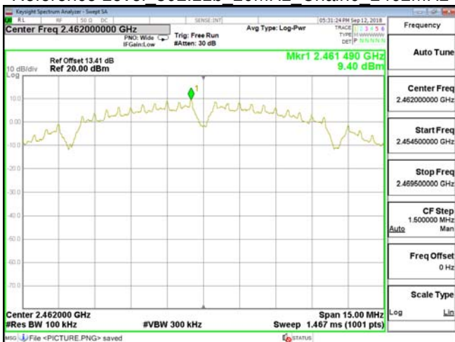
Reference Level 802.11b 20MHz Chain0 2462MHz
