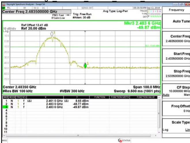
Band Edge 802.11b 20MHz Chain0 2462MHz
