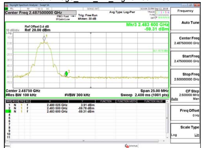
Band Edge BLE 2M HighCH39-2480
