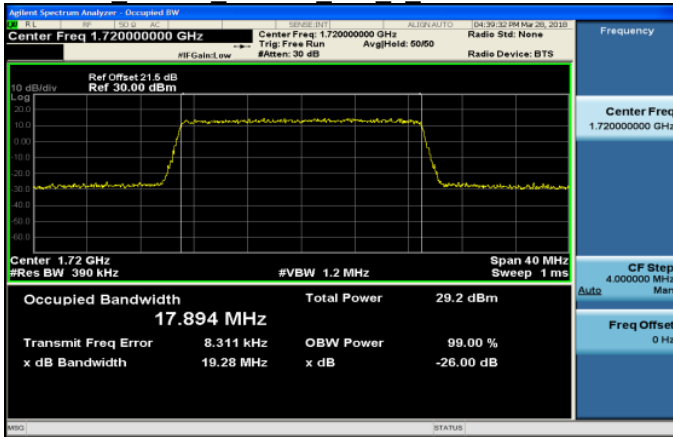
Band4 20MHz 16QAM 100 0 LowCH20050-1720
