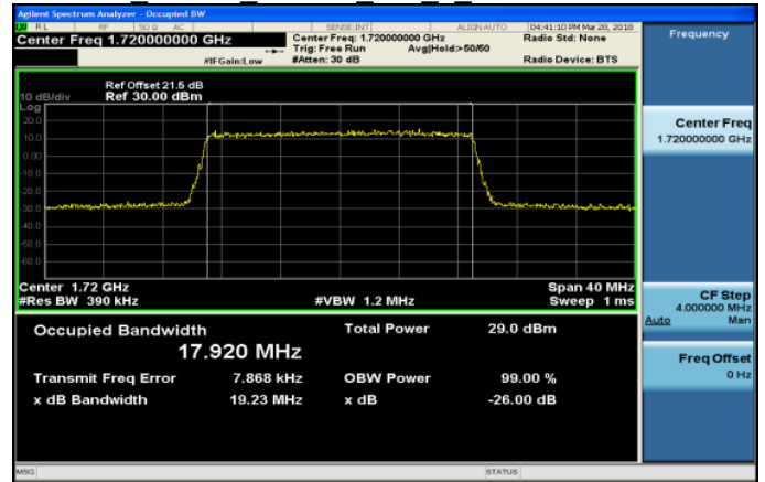
Band4 20MHz 64QAM 100 0 LowCH20050-1720
