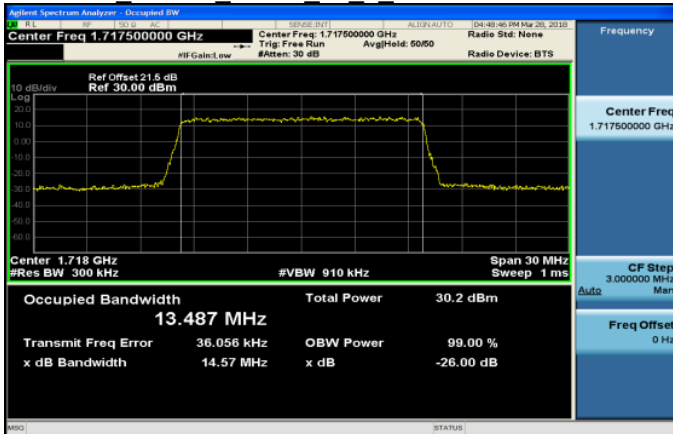
Band4 15MHz QPSK 75 0 LowCH20025-1717.5
