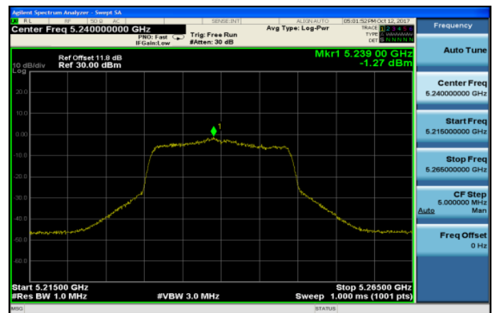
802.11n_20MHz_5240MHz
