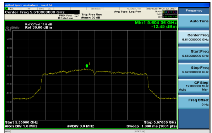
802.11ac_80MHz_5610MHz
