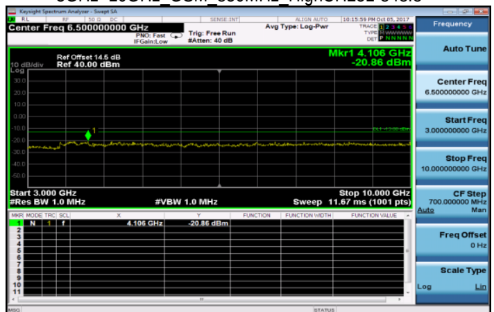
3GHz~10GHz GSM 850MHz HighCH251-848.8
