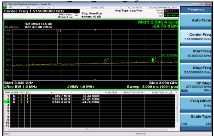
30MHz~3GHz GPRS 850MHz HighCH251-848.8
