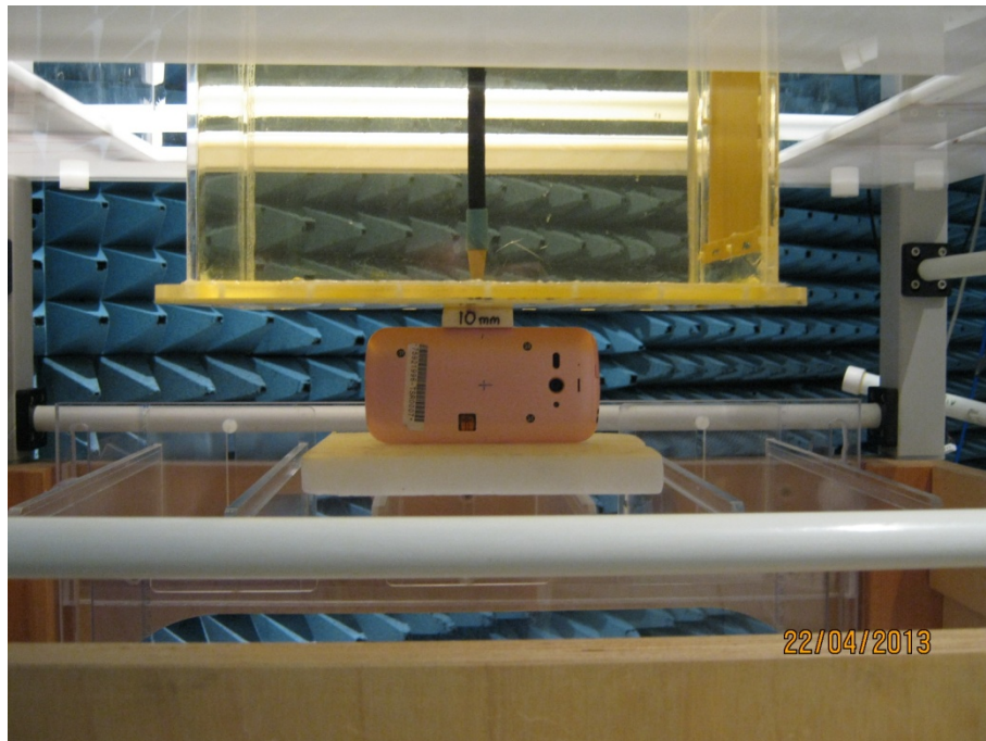
SAR - Body Left Edge
