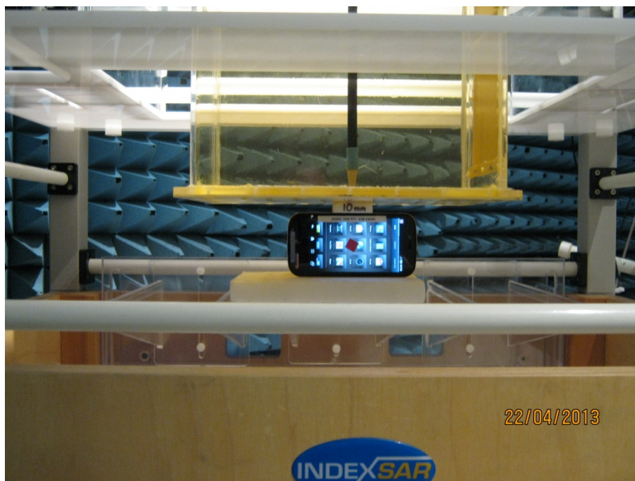
SAR - Body Right Edge
