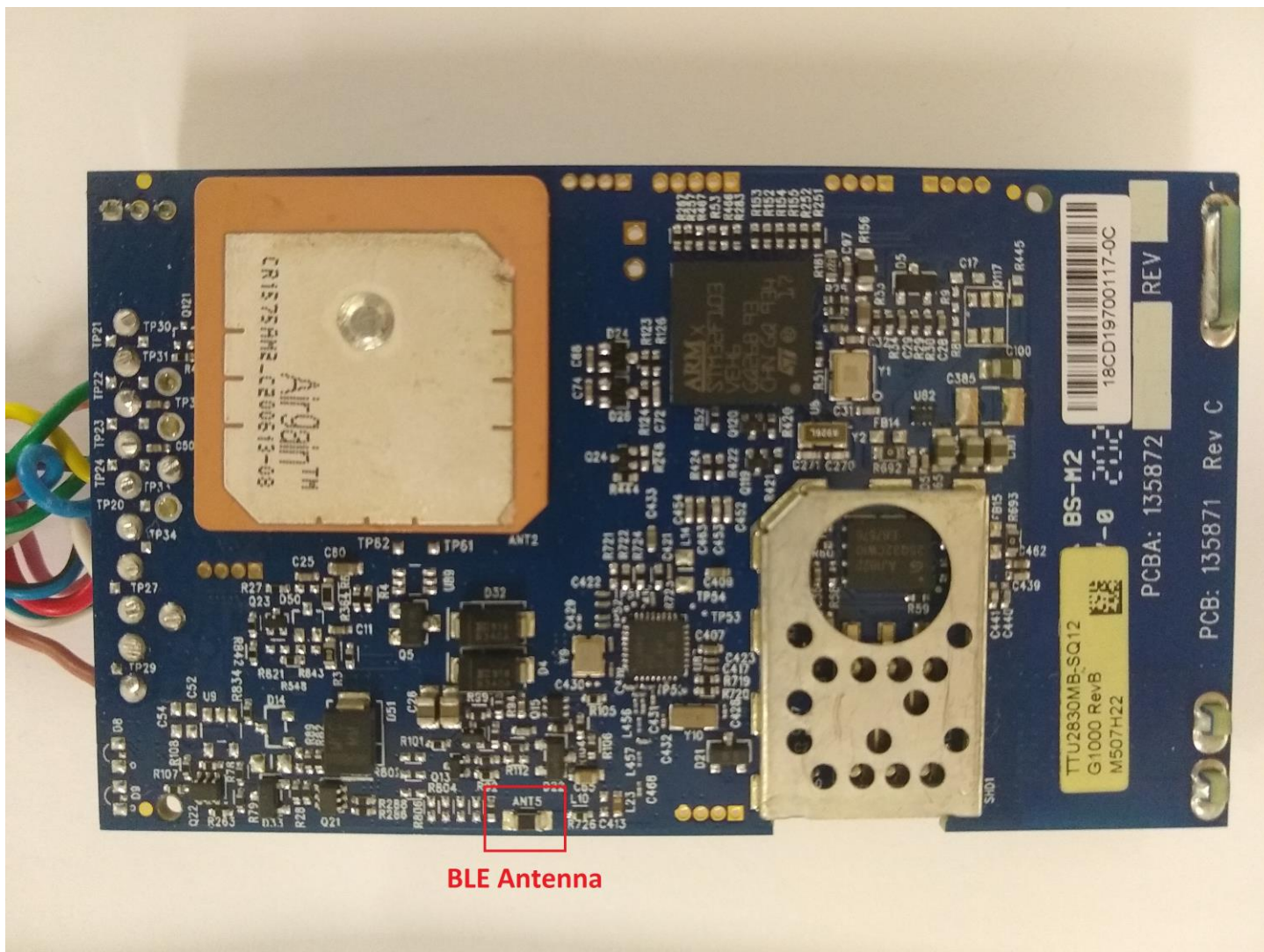
BLE Antenna Location
