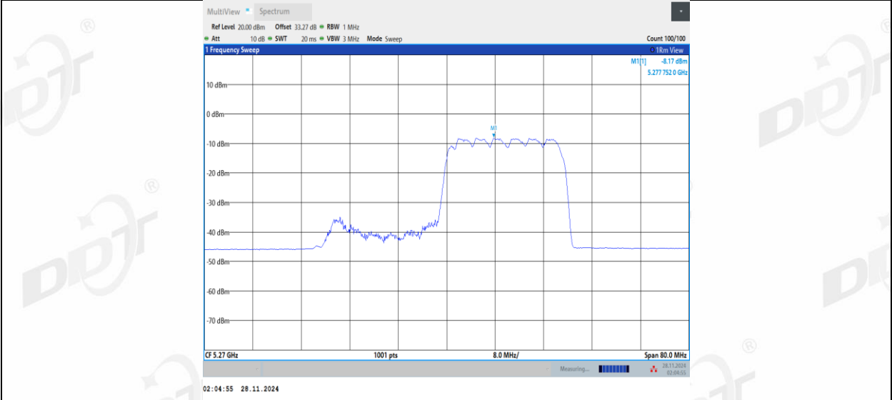
11AX40MIMO_Ant2_5270_106Tone_RU55
