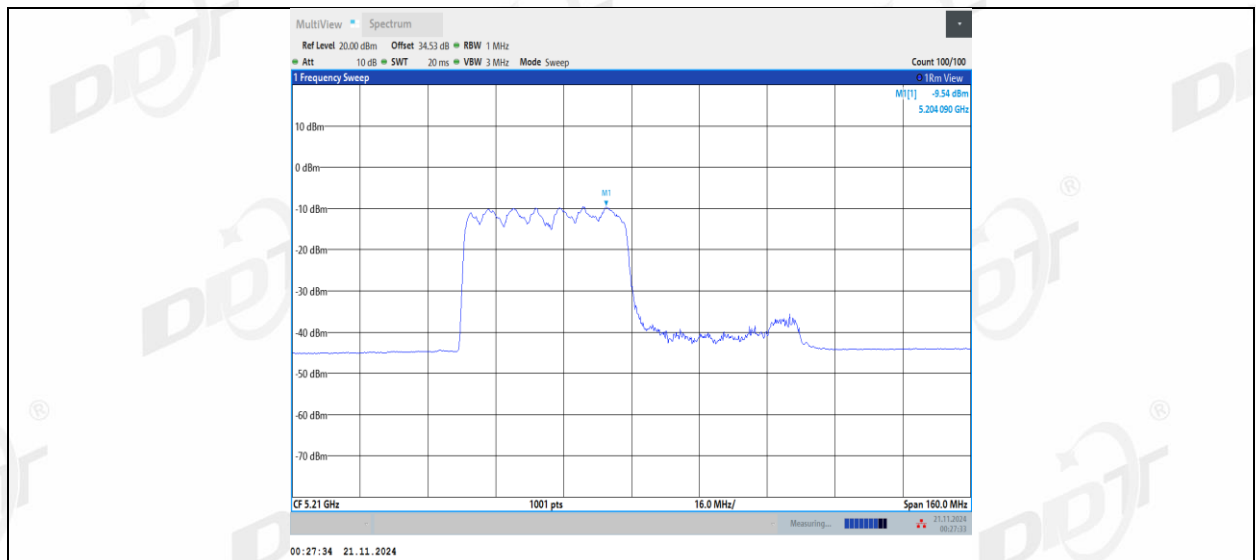
11AX80MIMO_Ant1_5210_484Tone_RU66
