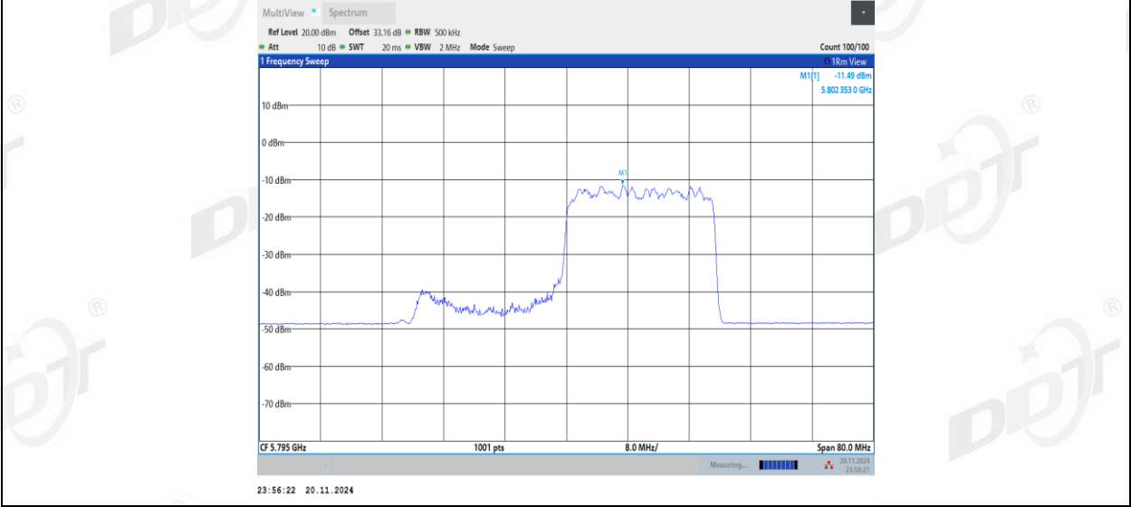
11AX40MIMO_Ant2_5795_106Tone_RU55
