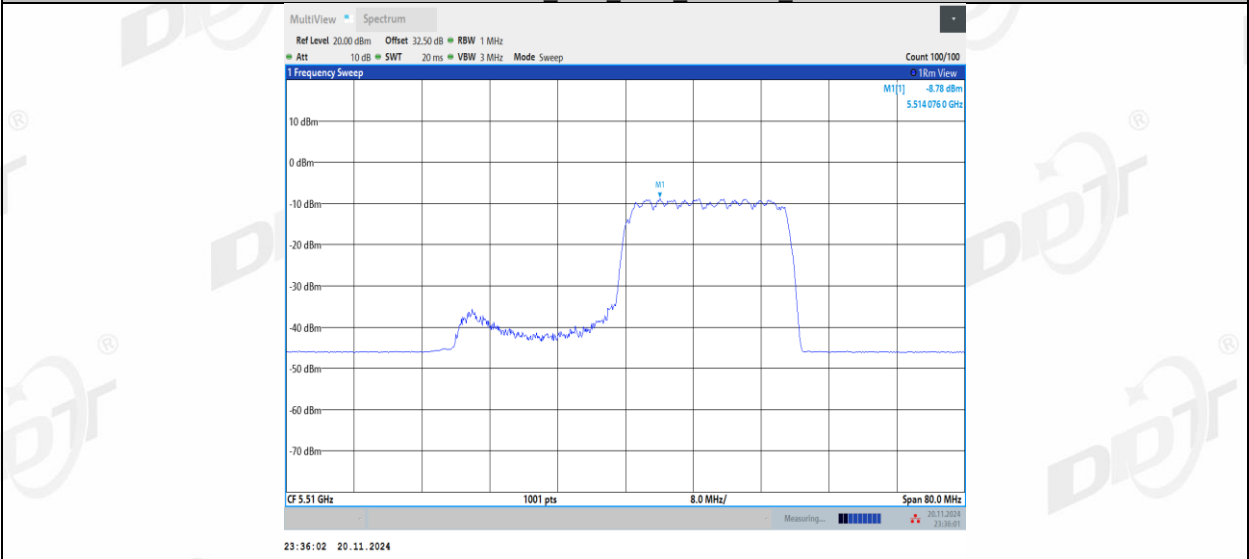
11AX40MIMO_Ant2_5510_106Tone_RU55
