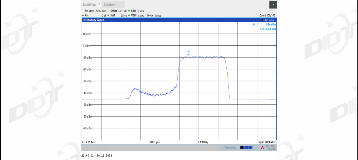
11AX40MIMO_Ant2_5550_106Tone_RU55
