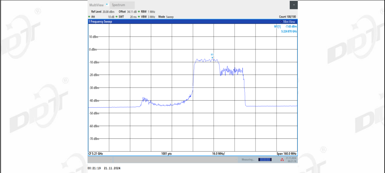
11AX80MIMO_Ant1_5210_242Tone_RU64
