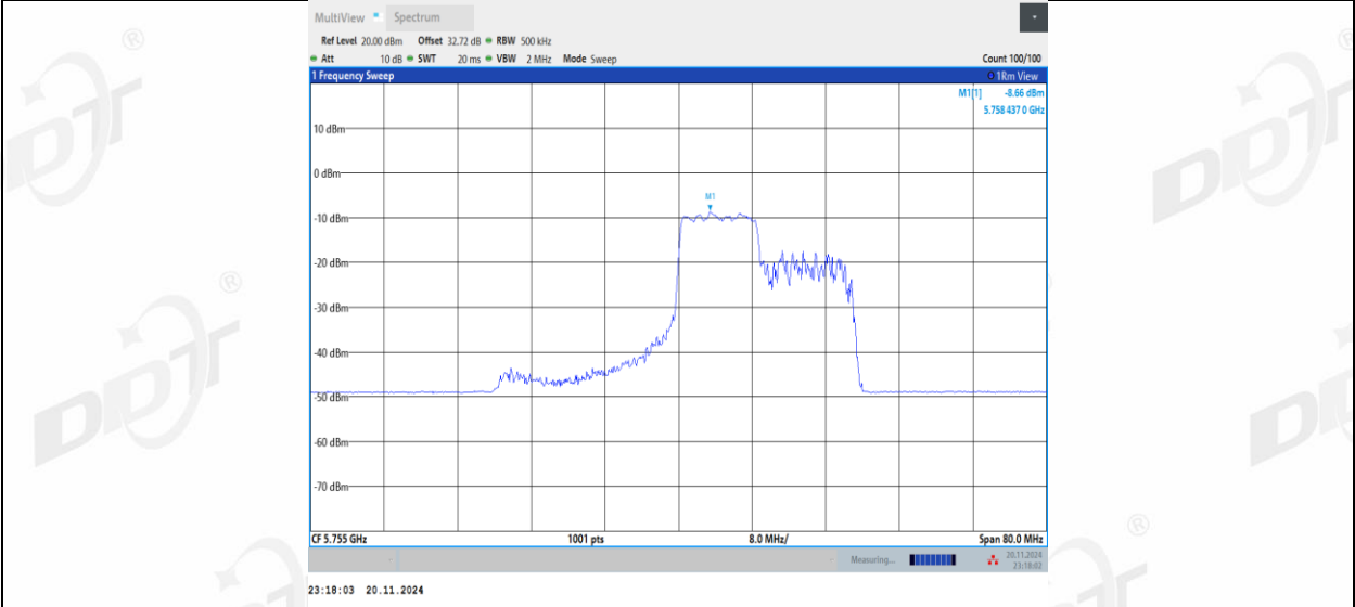
11AX40MIMO_Ant2_5755_106Tone_RU56
