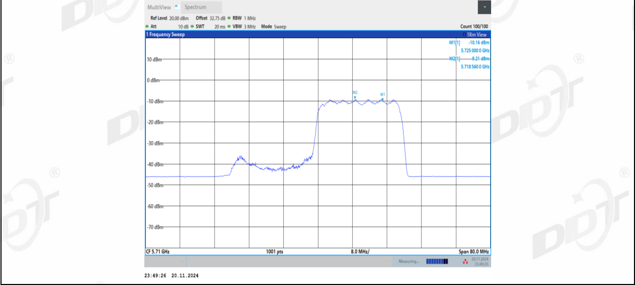
11AX40MIMO_Ant2_5710_UNII-2C_106Tone_RU55
