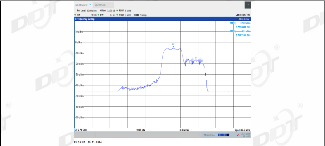
11AX40MIMO_Ant2_5710_UNII-2C_106Tone_RU56
