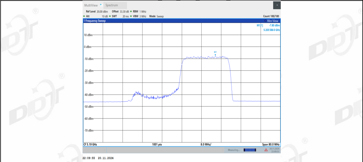
11AX40MIMO_Ant1_5230_106Tone_RU55
