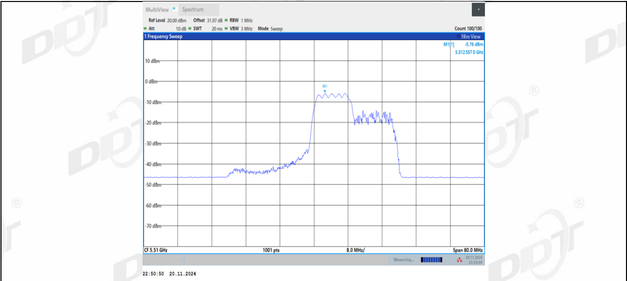
11AX40MIMO_Ant2_5510_106Tone_RU56
