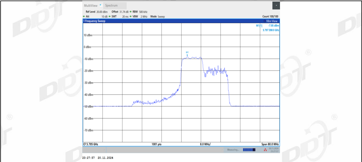
11AX40MIMO_Ant2_5795_106Tone_RU56
