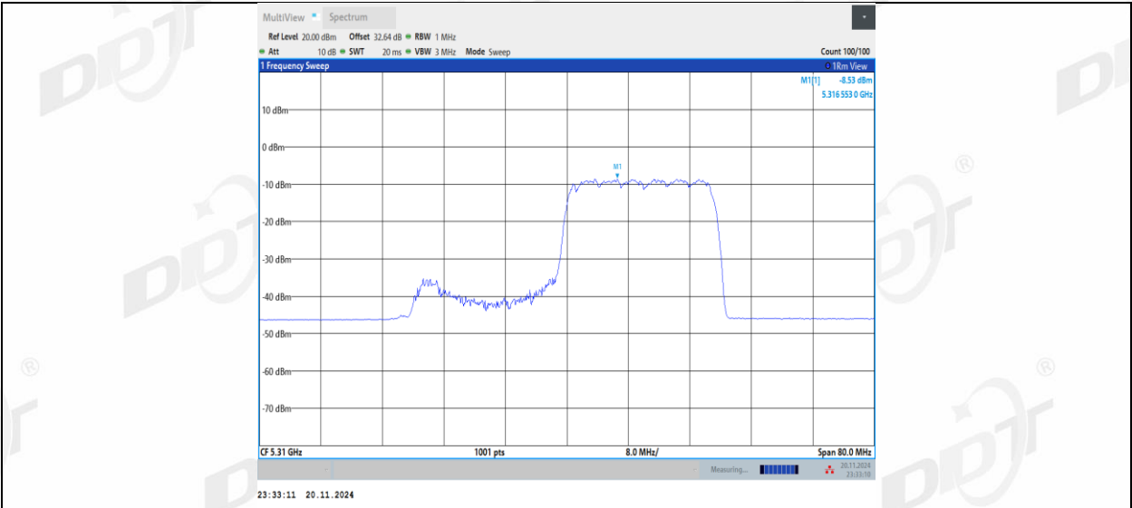
11AX40MIMO_Ant2_5310_106Tone_RU55
