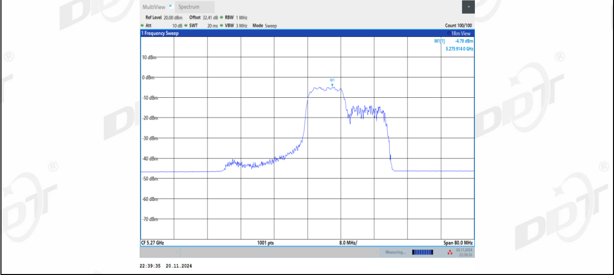
11AX40MIMO_Ant2_5270_106Tone_RU56
