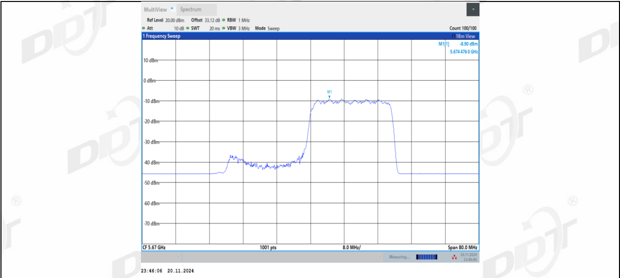
11AX40MIMO_Ant2_5670_106Tone_RU55
