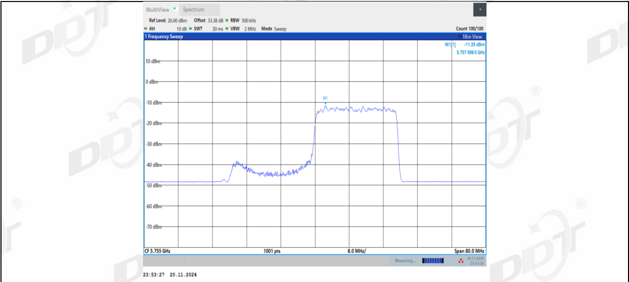
11AX40MIMO_Ant2_5755_106Tone_RU55
