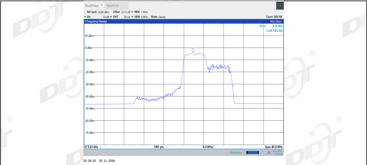
11AX40MIMO_Ant2_5230_106Tone_RU56
