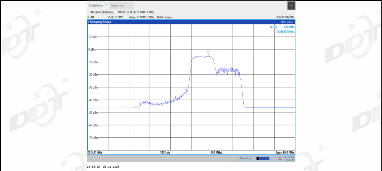
11AX40MIMO_Ant2_5310_106Tone_RU56
