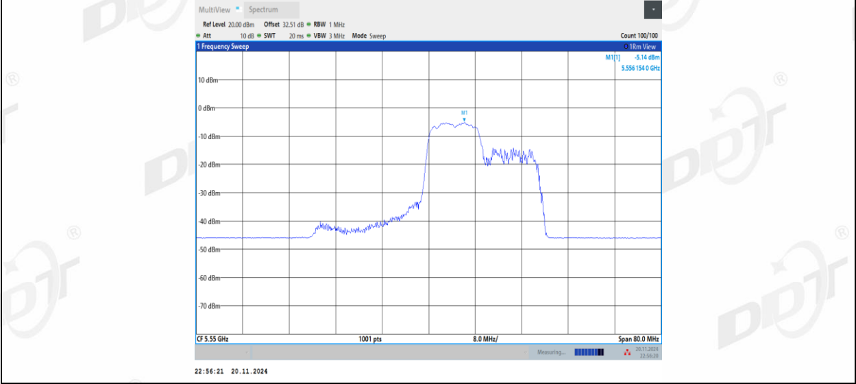
11AX40MIMO_Ant2_5550_106Tone_RU56
