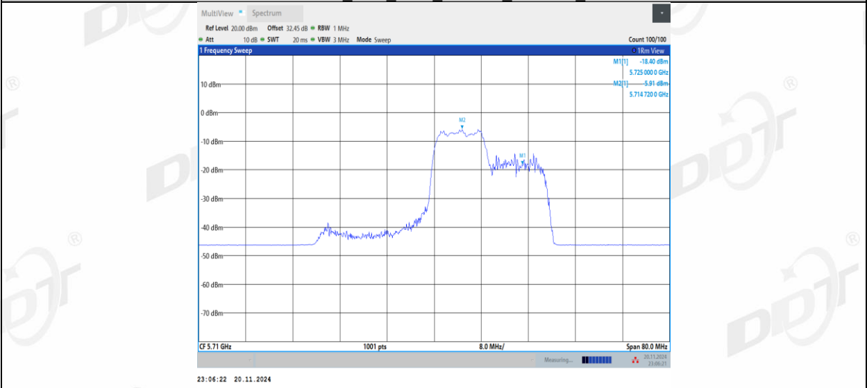
11AX40MIMO_Ant1_5710_UNII-2C_106Tone_RU56
