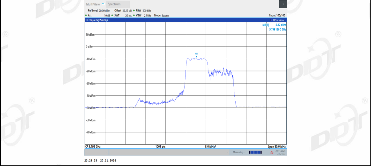
11AX40MIMO_Ant1_5795_106Tone_RU56
