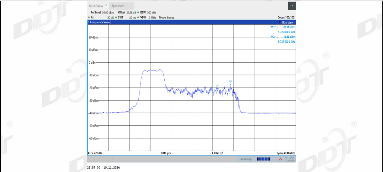
11AX20MIMO_Ant1_5720_UNII-3_52Tone_RU38
