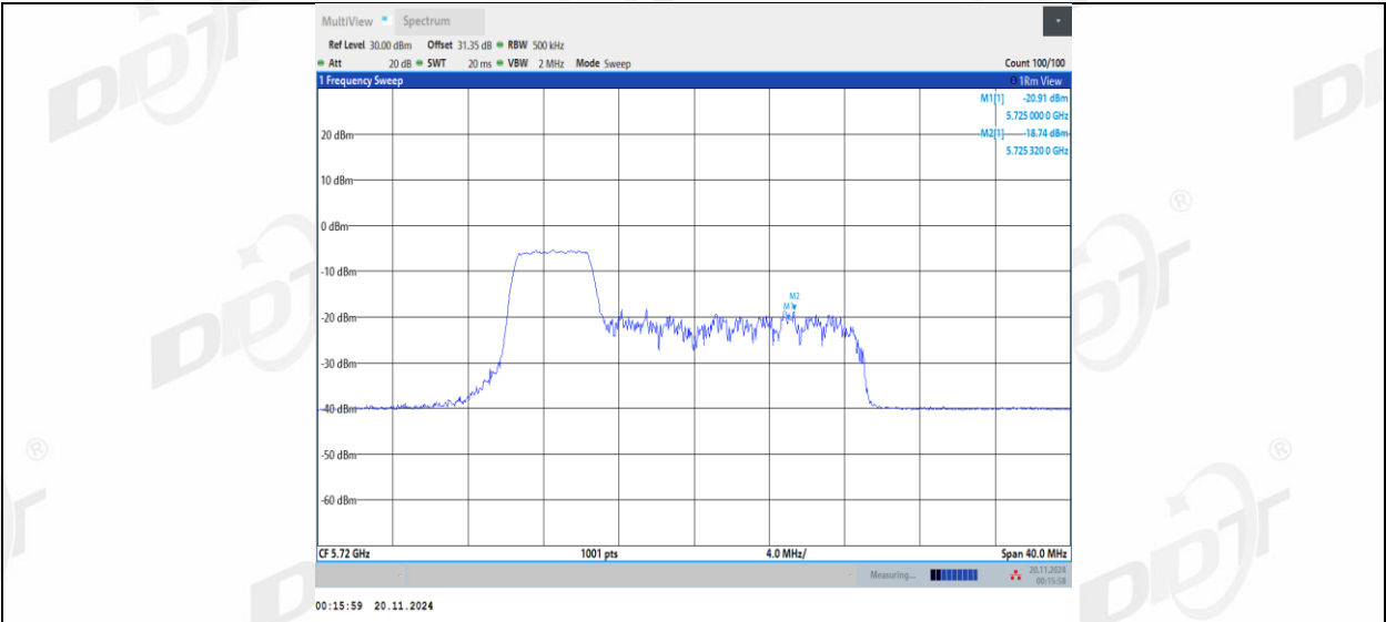
11AX20MIMO_Ant2_5720_UNII-3_52Tone_RU38
