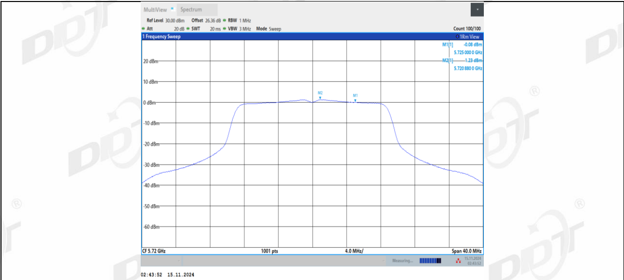
11AC20MIMO_Ant2_5720_UNII-2C
