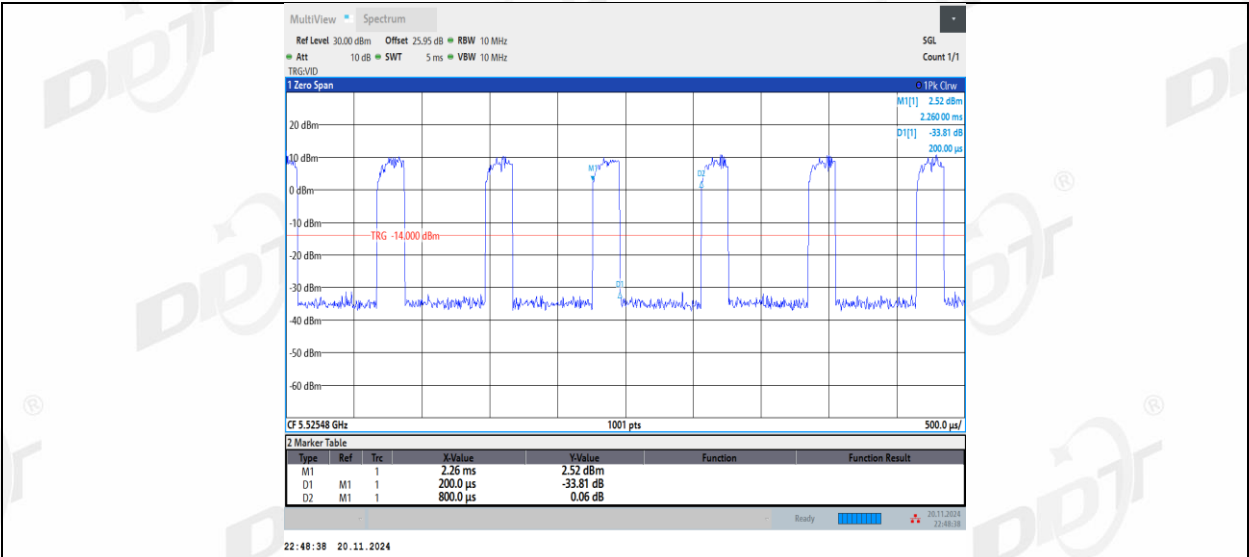
11AX40MIMO_Ant1_5510_242Tone_RU61
