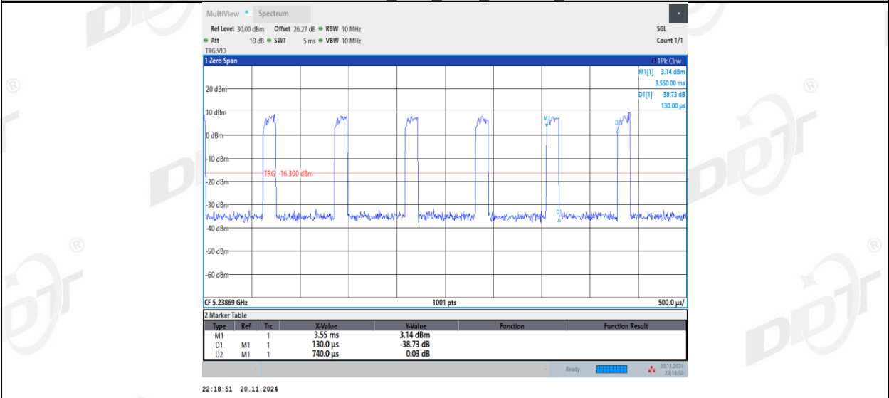
11AX40MIMO_Ant2_5230_106Tone_RU55
