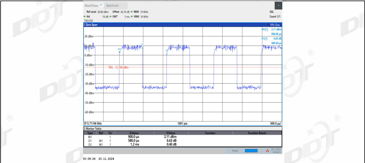
11AX20MIMO_Ant2_5720_26Tone_RU4
