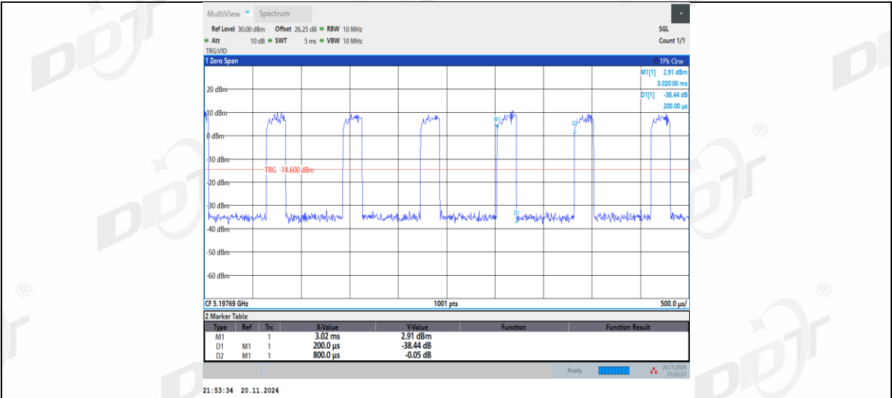
11AX40MIMO_Ant1_5190_106Tone_RU56
