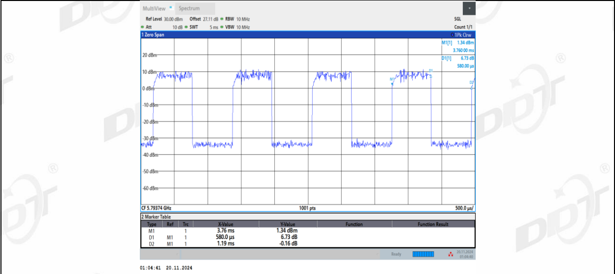
11AX20MIMO_Ant1_5785_52Tone_RU37
