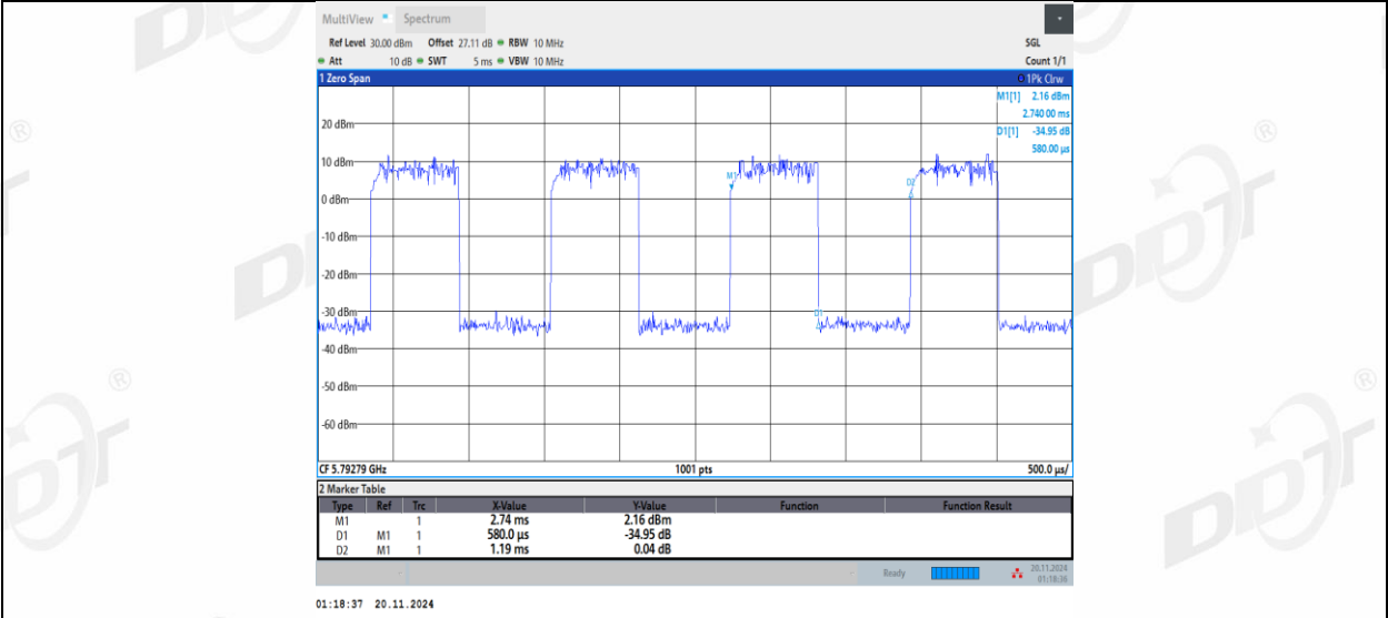
11AX20MIMO_Ant2_5785_52Tone_RU37
