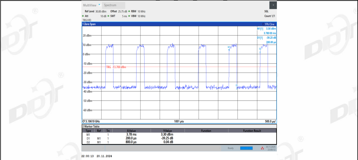
11AX40MIMO_Ant2_5190_106Tone_RU56
