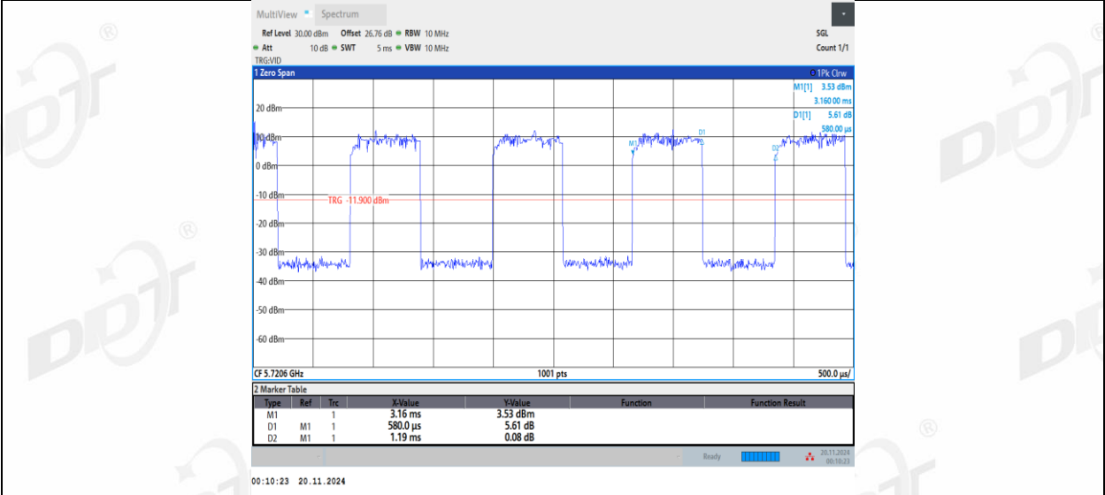
11AX20MIMO_Ant2_5720_26Tone_RU8
