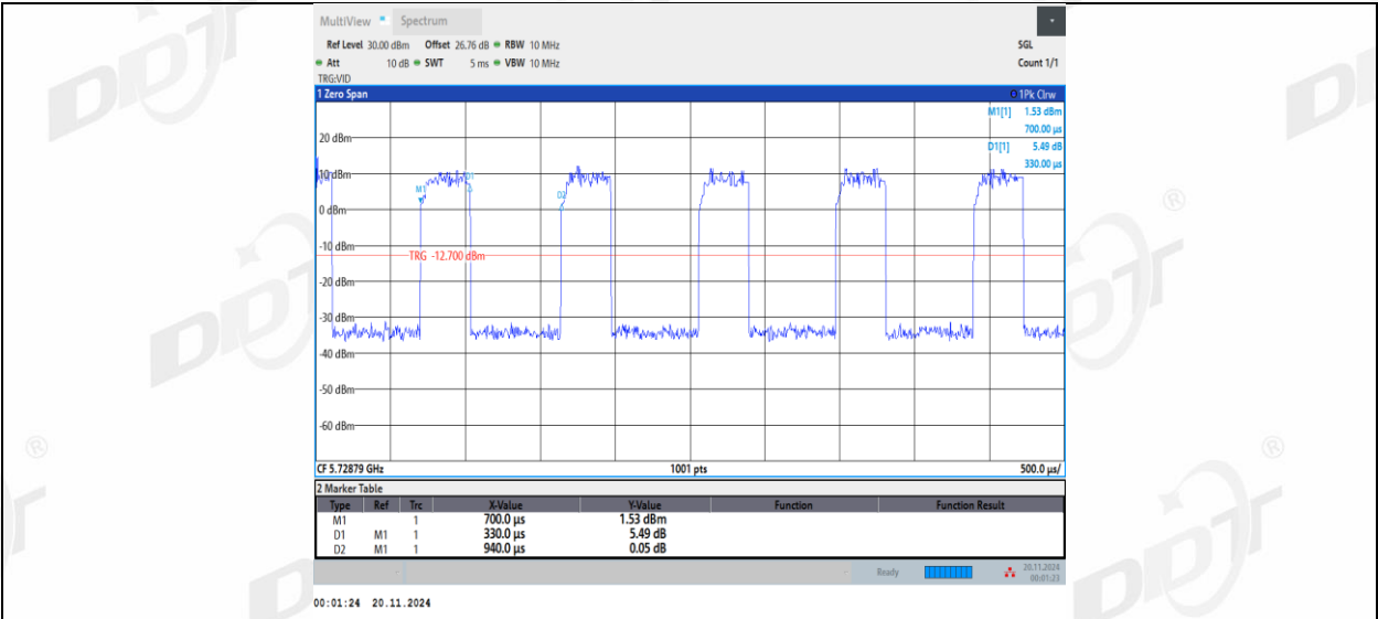
11AX20MIMO_Ant1_5720_106Tone_RU53
