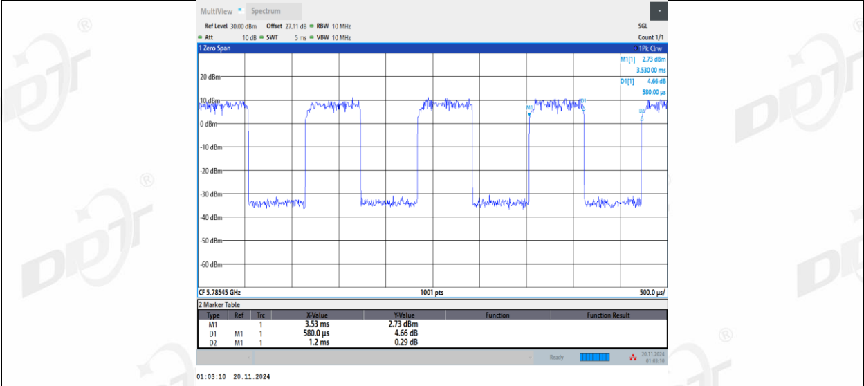
11AX20MIMO_Ant1_5785_26Tone_RU8
