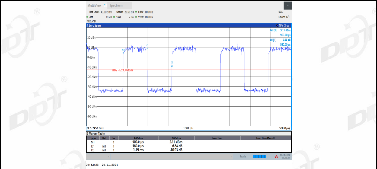
11AX20MIMO_Ant1_5745_26Tone_RU8
