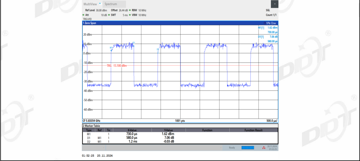
11AX20MIMO_Ant2_5825_52Tone_RU37
