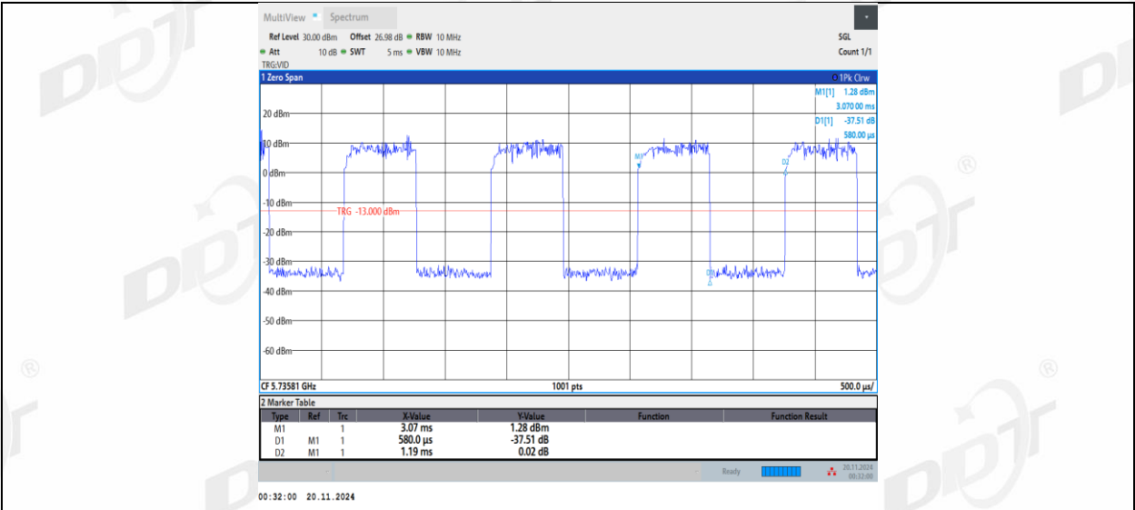
11AX20MIMO_Ant1_5745_26Tone_RU4
