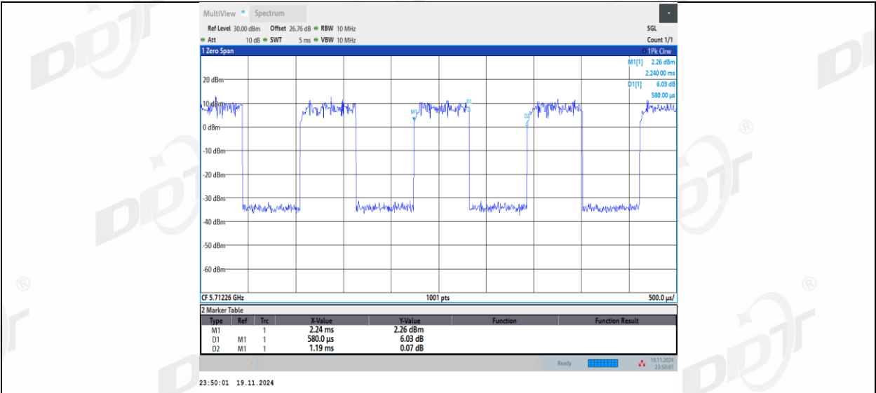
11AX20MIMO_Ant1_5720_26Tone_RU4
