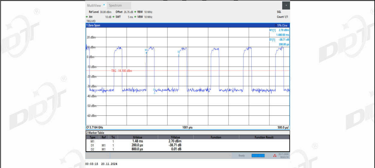
11AX20MIMO_Ant1_5720_106Tone_RU54
