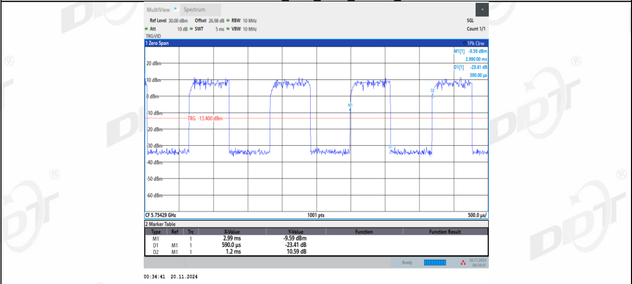
11AX20MIMO_Ant1_5745_52Tone_RU37
