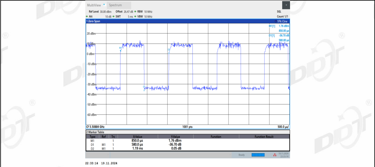
11AX20MIMO_Ant1_5500_52Tone_RU37
