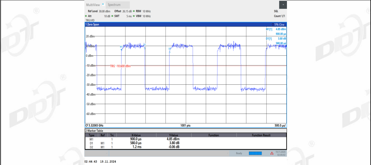
11AX20MIMO_Ant2_5320_26Tone_RU8
