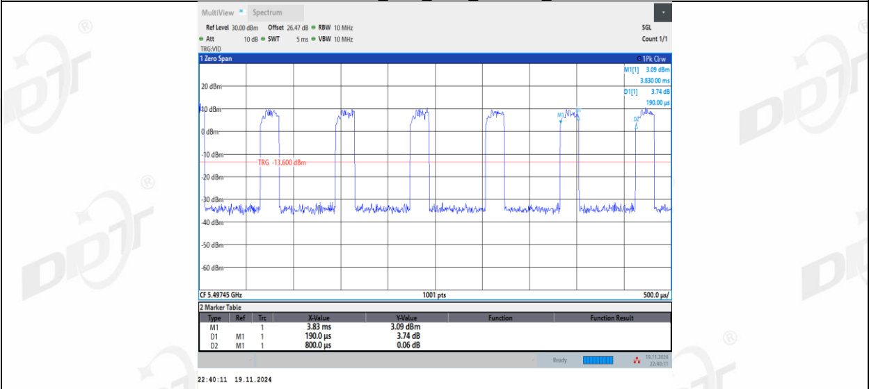
11AX20MIMO_Ant1_5500_106Tone_RU54
