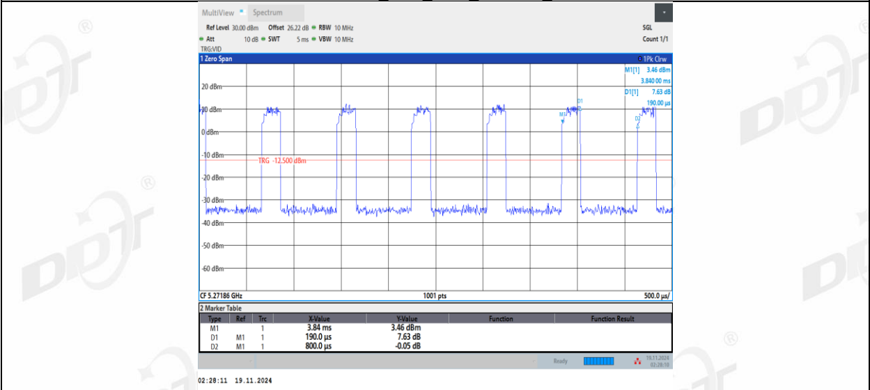
11AX20MIMO_Ant2_5280_106Tone_RU54
