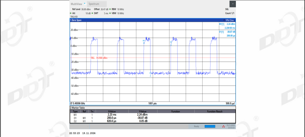
11AX20MIMO_Ant2_5500_106Tone_RU54
