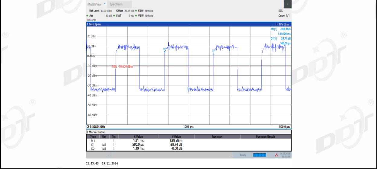
11AX20MIMO_Ant1_5320_52Tone_RU37
