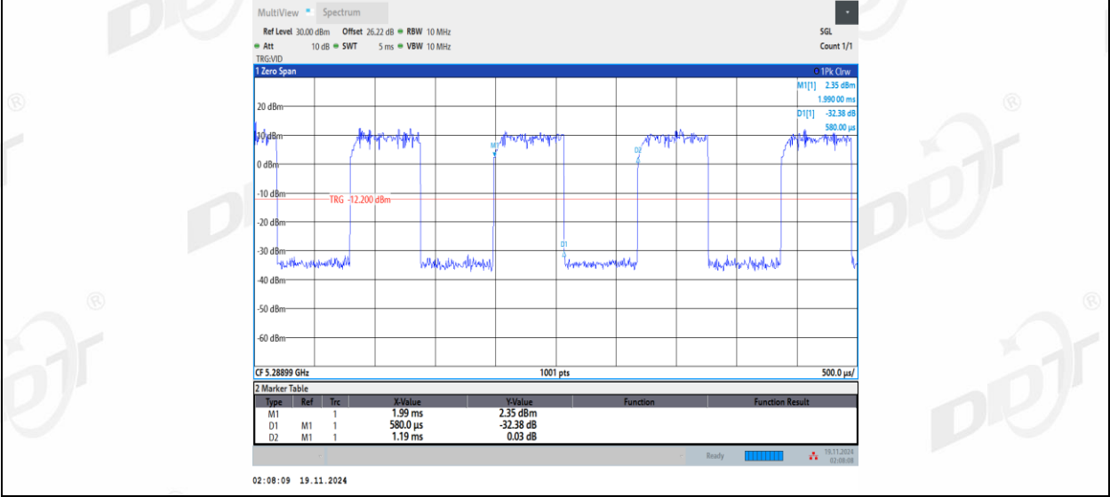
11AX20MIMO_Ant1_5280_52Tone_RU37
