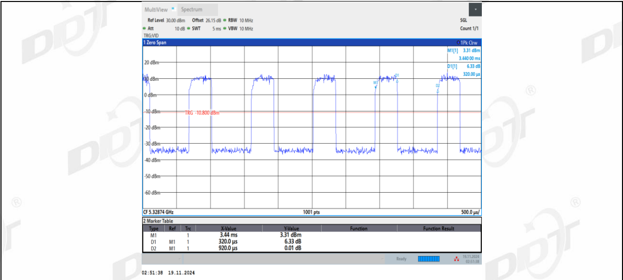
11AX20MIMO_Ant2_5320_106Tone_RU53
