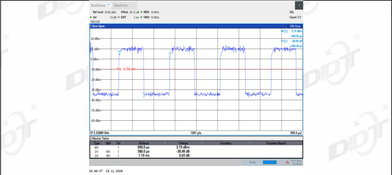
11AX20MIMO_Ant2_5320_52Tone_RU37
