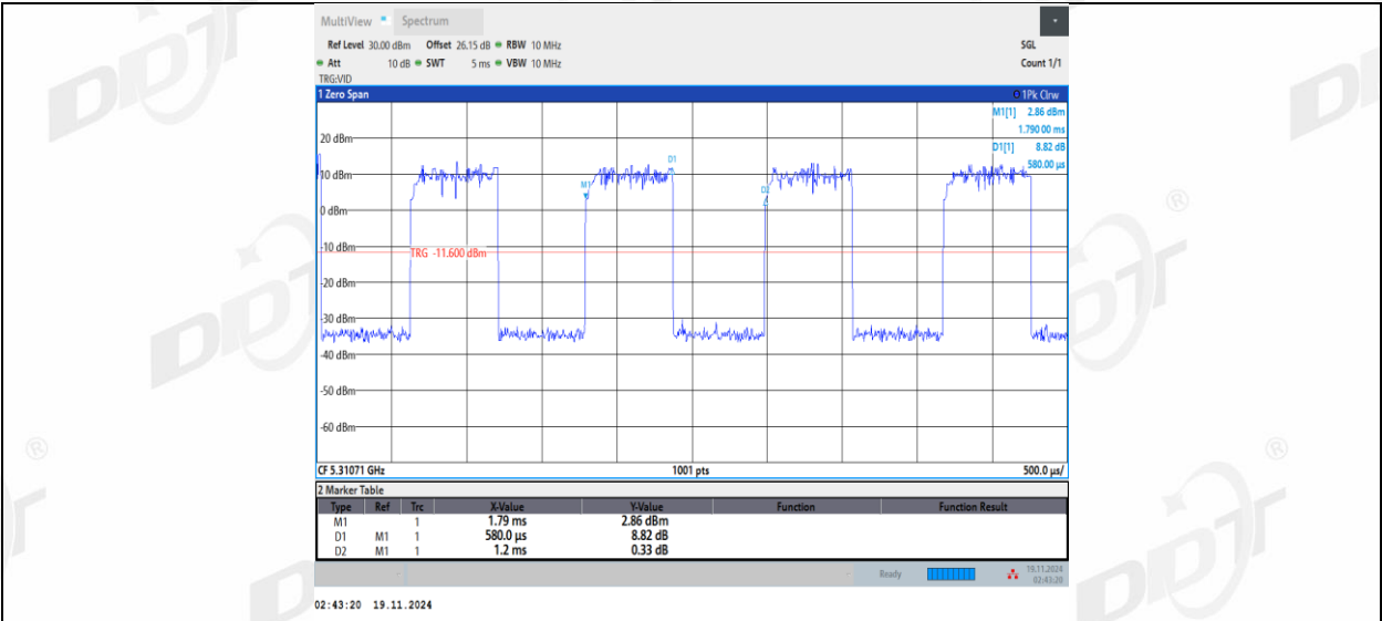
11AX20MIMO_Ant2_5320_26Tone_RU4
