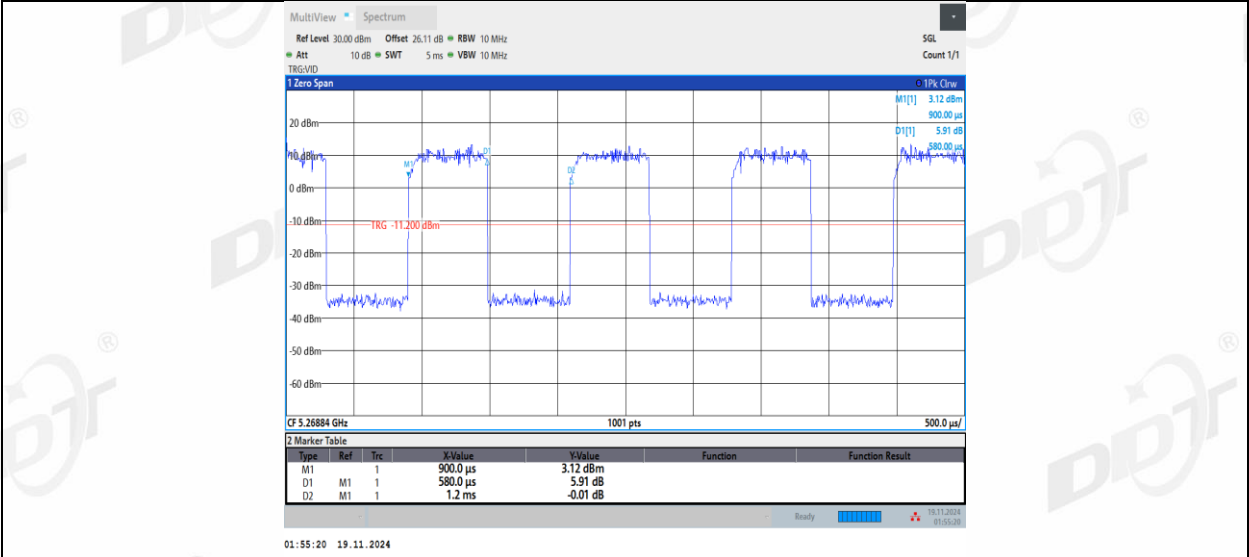
11AX20MIMO_Ant2_5260_52Tone_RU7
