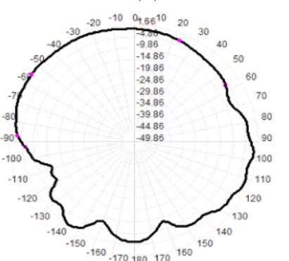
2460.0MHz Total(E2), Max= 1.66dBi
