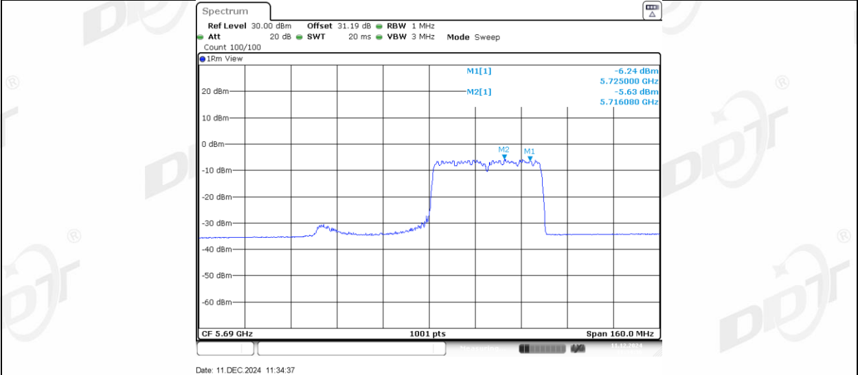
11AX80MIMO_Ant2_5690_UNII-2C_484Tone_RU65
