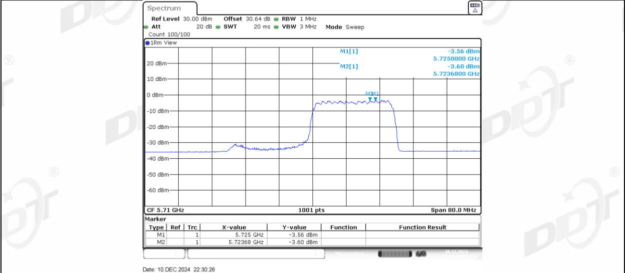
11AX40MIMO_Ant1_5710_UNII-3_242Tone_RU61
