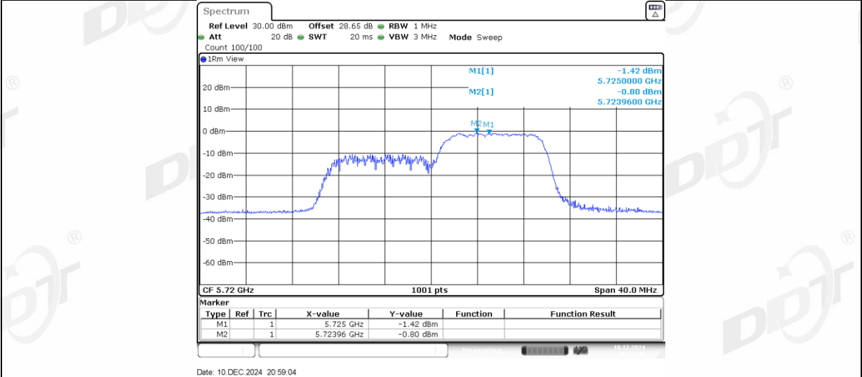
11AX20MIMO_Ant1_5720_UNII-3_26Tone_RU0
