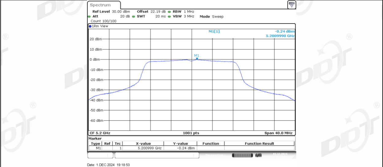
11AC20MIMO_Ant2_5200
