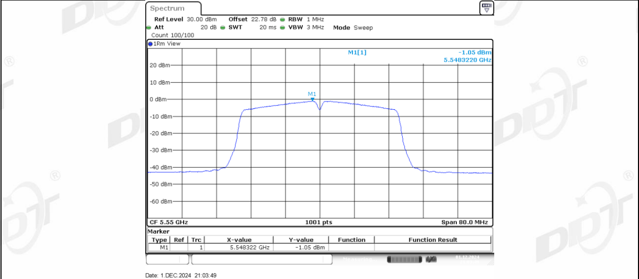
11AC40MIMO_Ant2_5550
