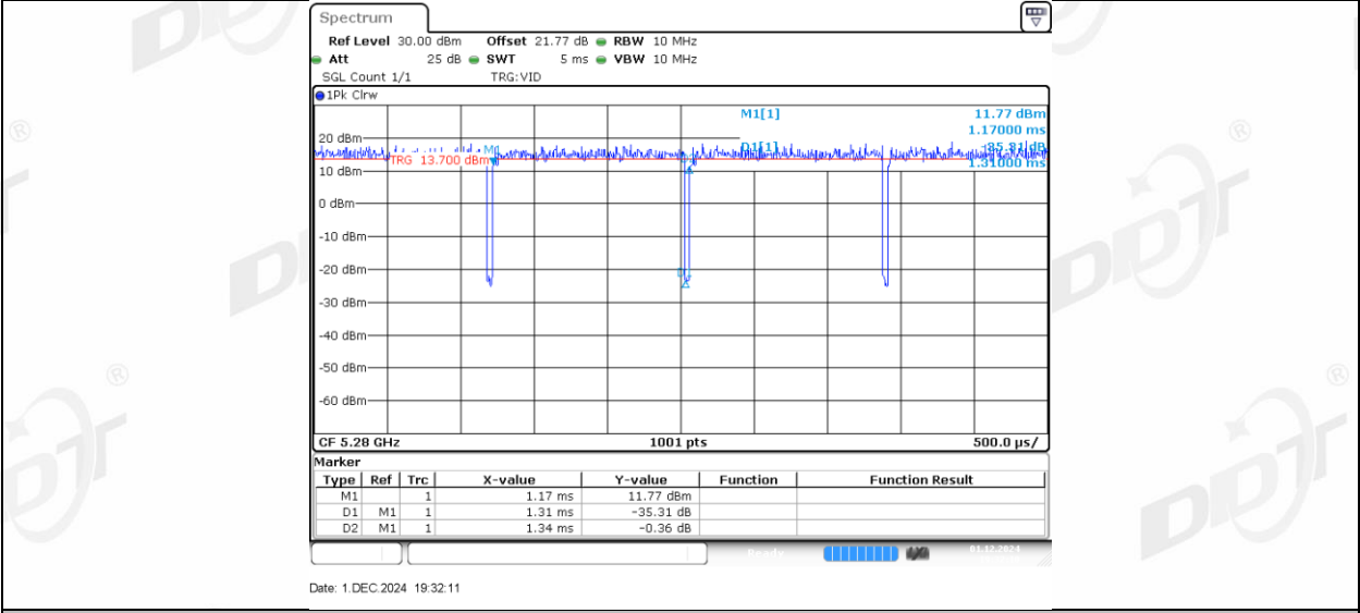
11AC20MIMO_Ant2_5280
