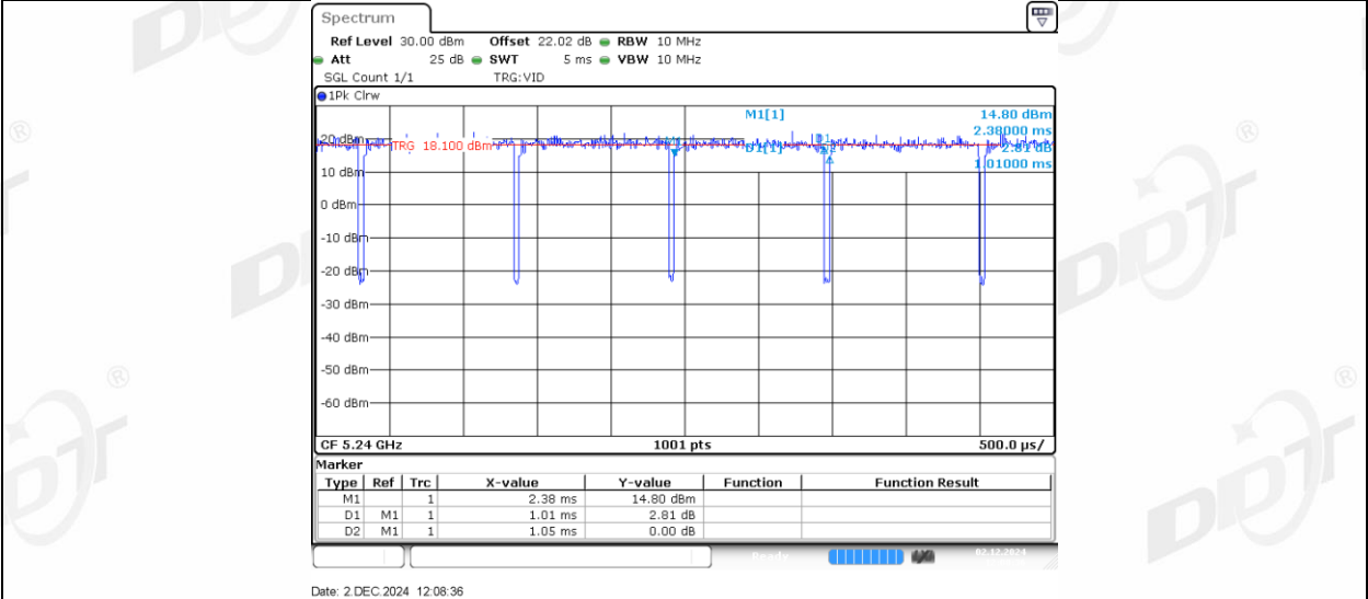
11AX20MIMO_Ant2_5240
