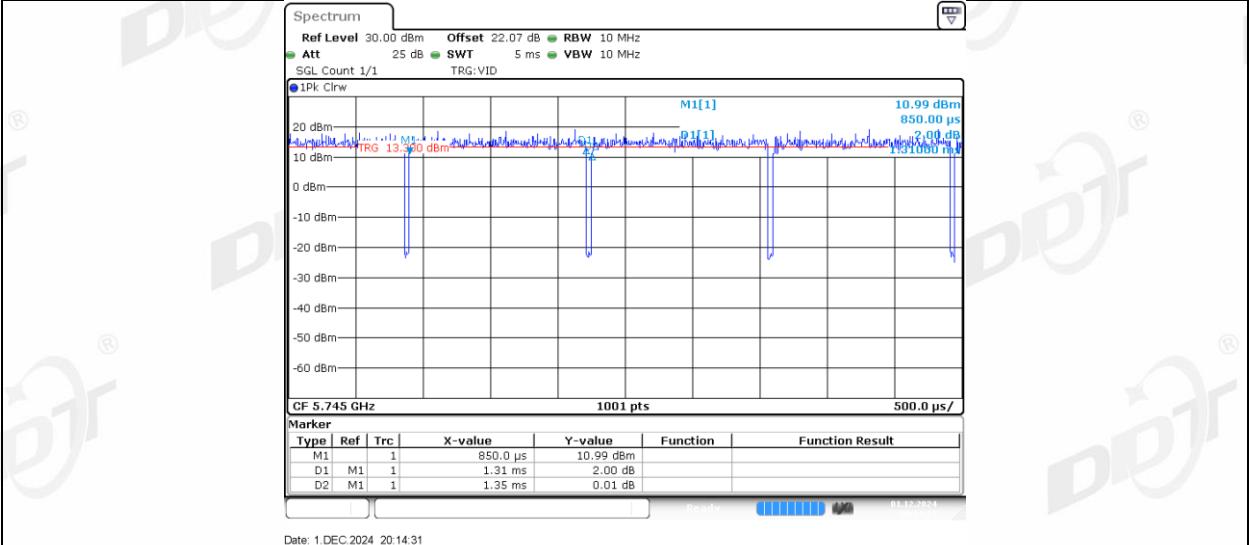
11AC20MIMO_Ant2_5745
