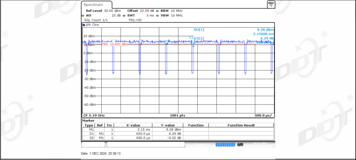
11AC40MIMO_Ant2_5190
