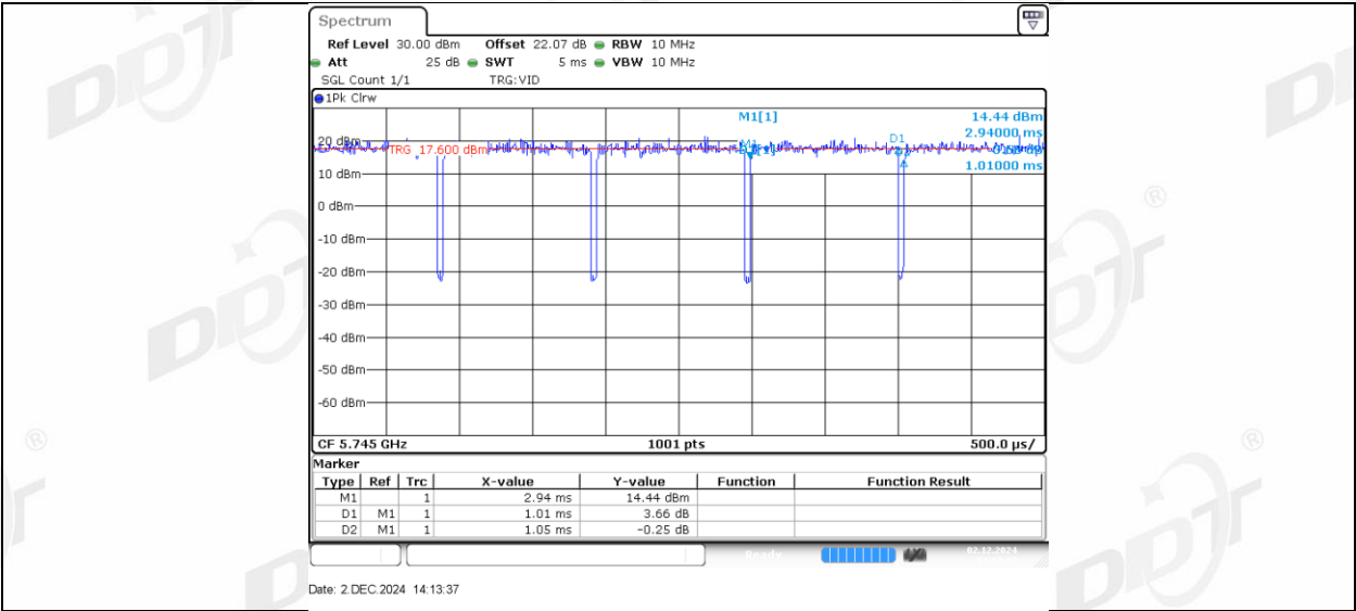
11AX20MIMO_Ant2_5745
