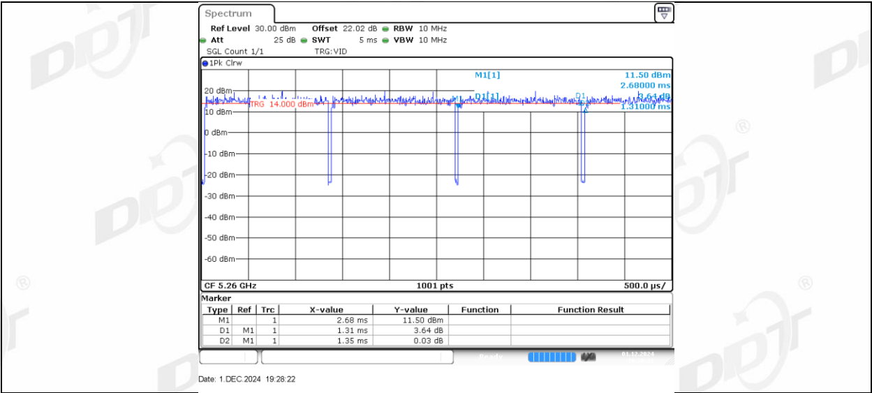
11AC20MIMO_Ant2_5260
