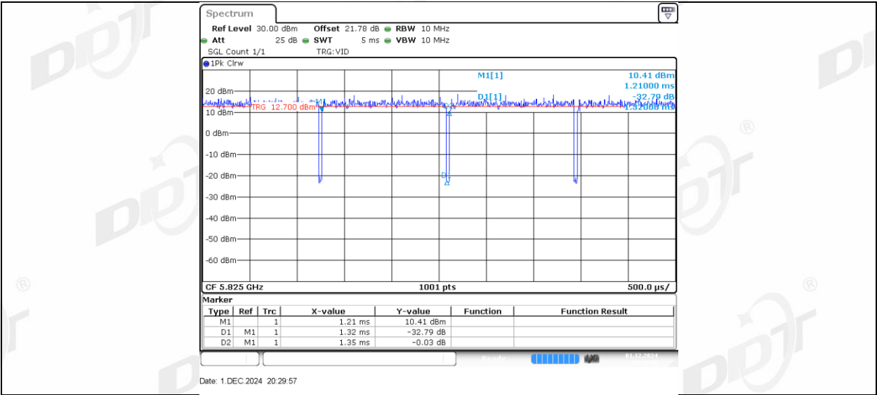
11AC20MIMO_Ant2_5825
