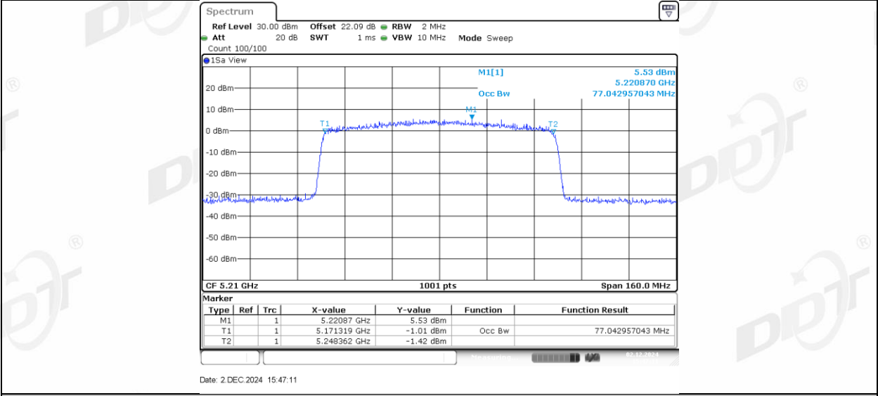
11AX80MIMO_Ant2_5210
