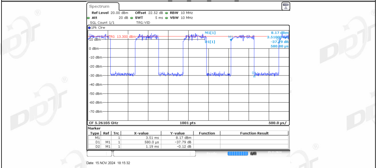
11AX20MIMO_Ant1_5260_26Tone_RU8
