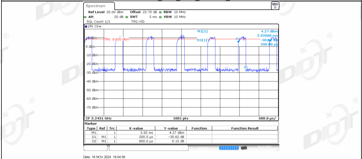
11AX20MIMO_Ant1_5260_26Tone_RU0
