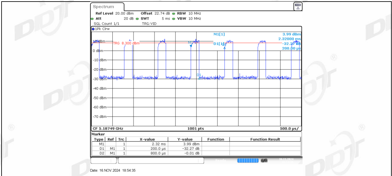
11AX20MIMO_Ant1_5200_26Tone_RU0
