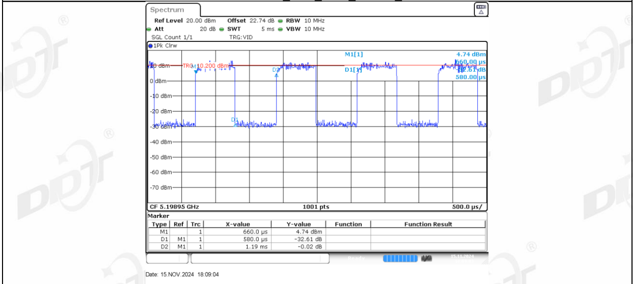
11AX20MIMO_Ant2_5200_26Tone_RU8
