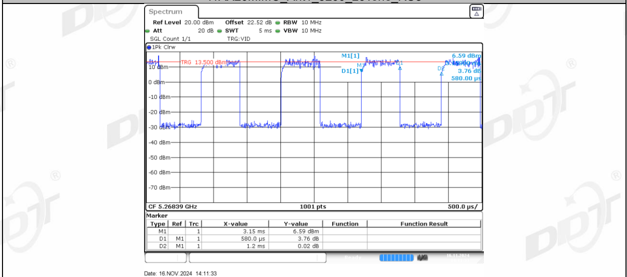
11AX20MIMO_Ant1_5260_52Tone_RU37
