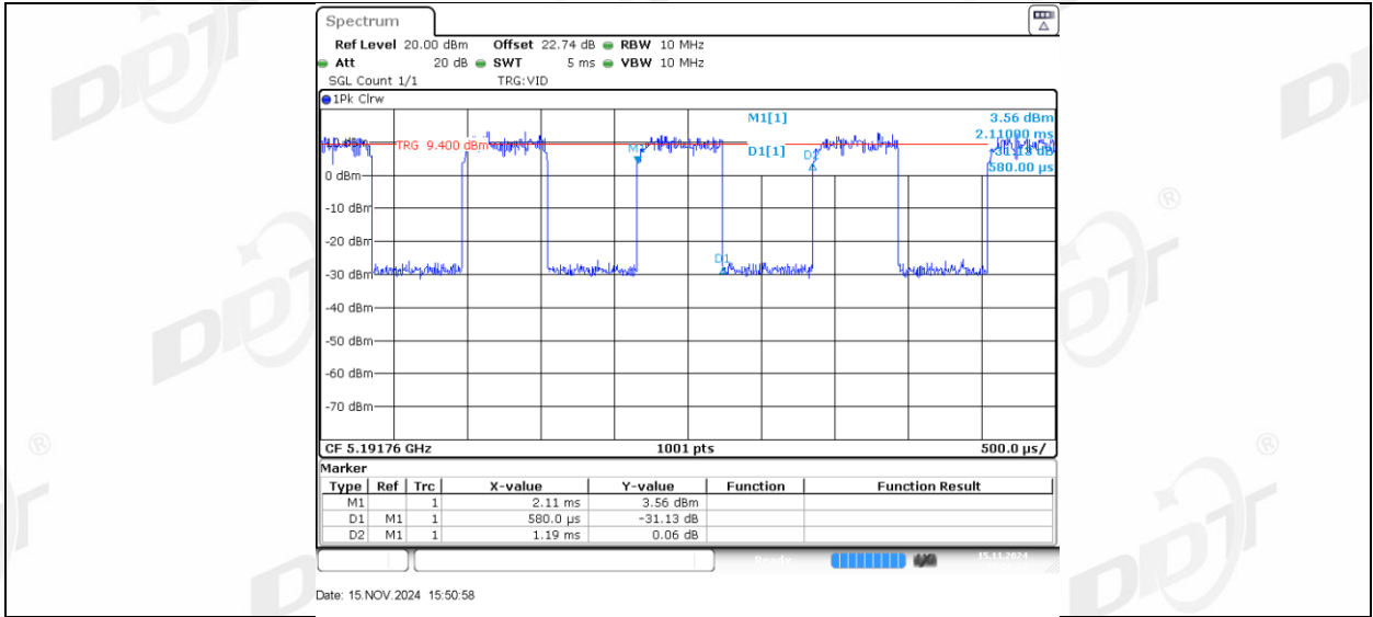
11AX20MIMO_Ant2_5200_26Tone_RU4
