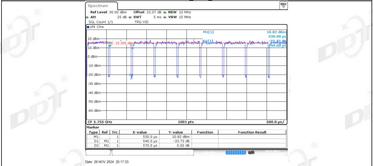
11AX40MIMO_Ant2_5755
