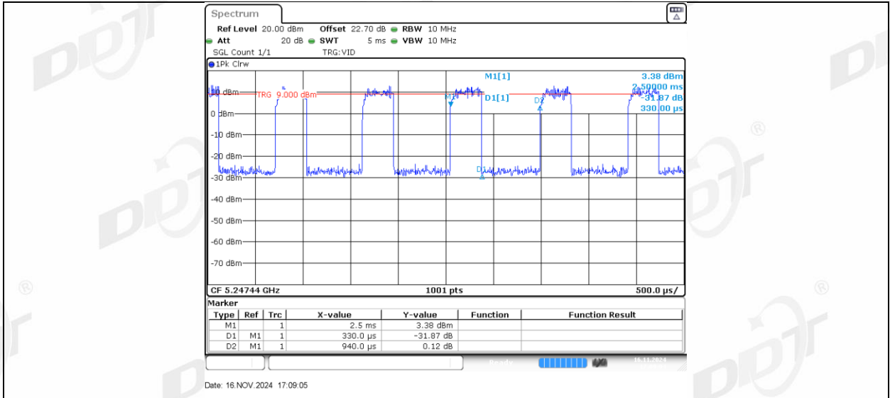
11AX20MIMO_Ant2_5240_106Tone_RU53
