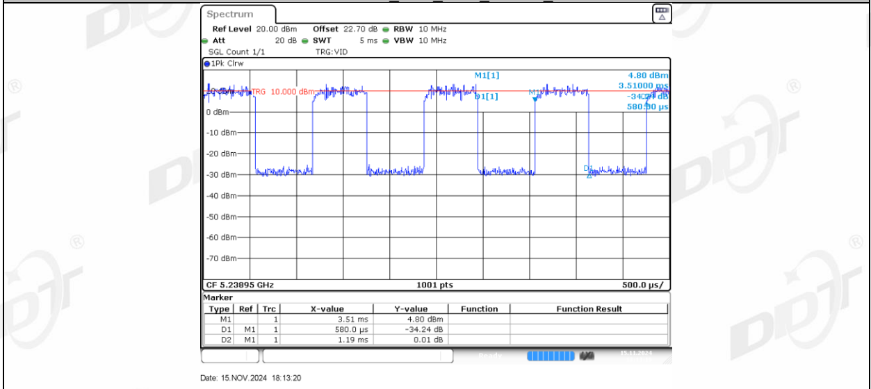
11AX20MIMO_Ant2_5240_26Tone_RU8
