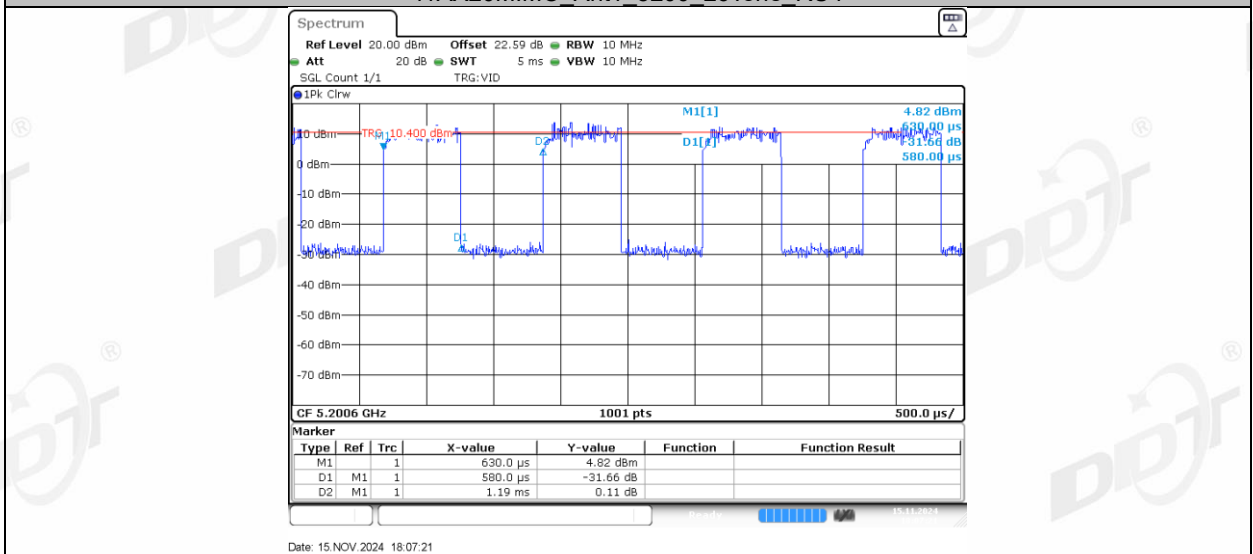
11AX20MIMO_Ant1_5200_26Tone_RU8
