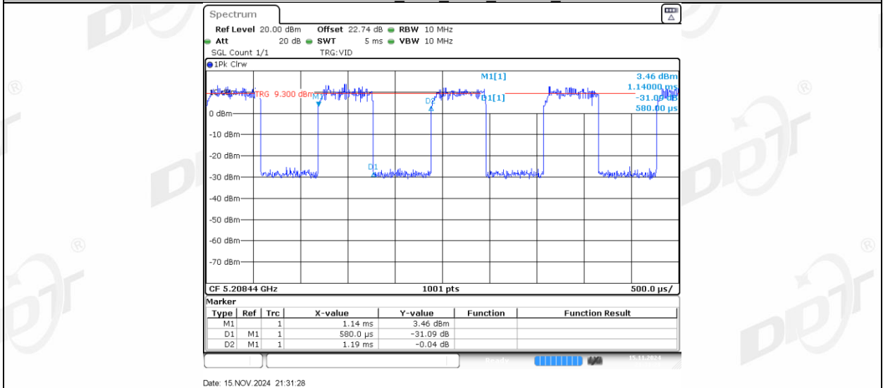
11AX20MIMO_Ant2_5200_52Tone_RU37
