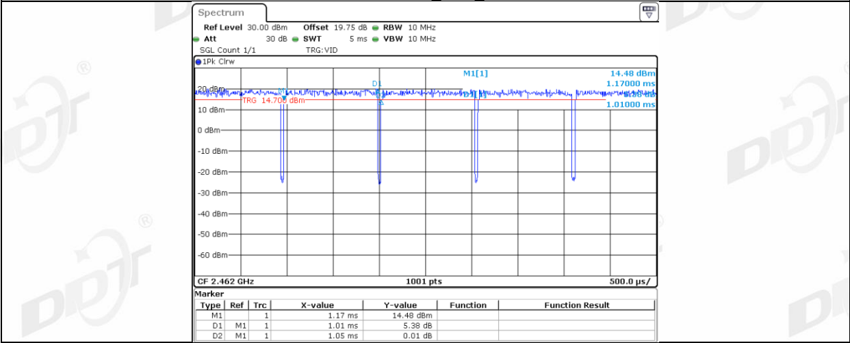
11AX20MIMO_Ant2_2462
