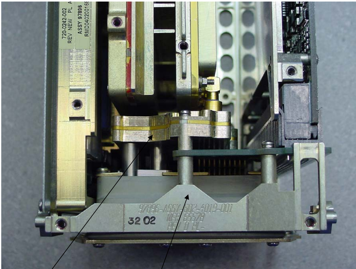
Antenna Coupler Module
