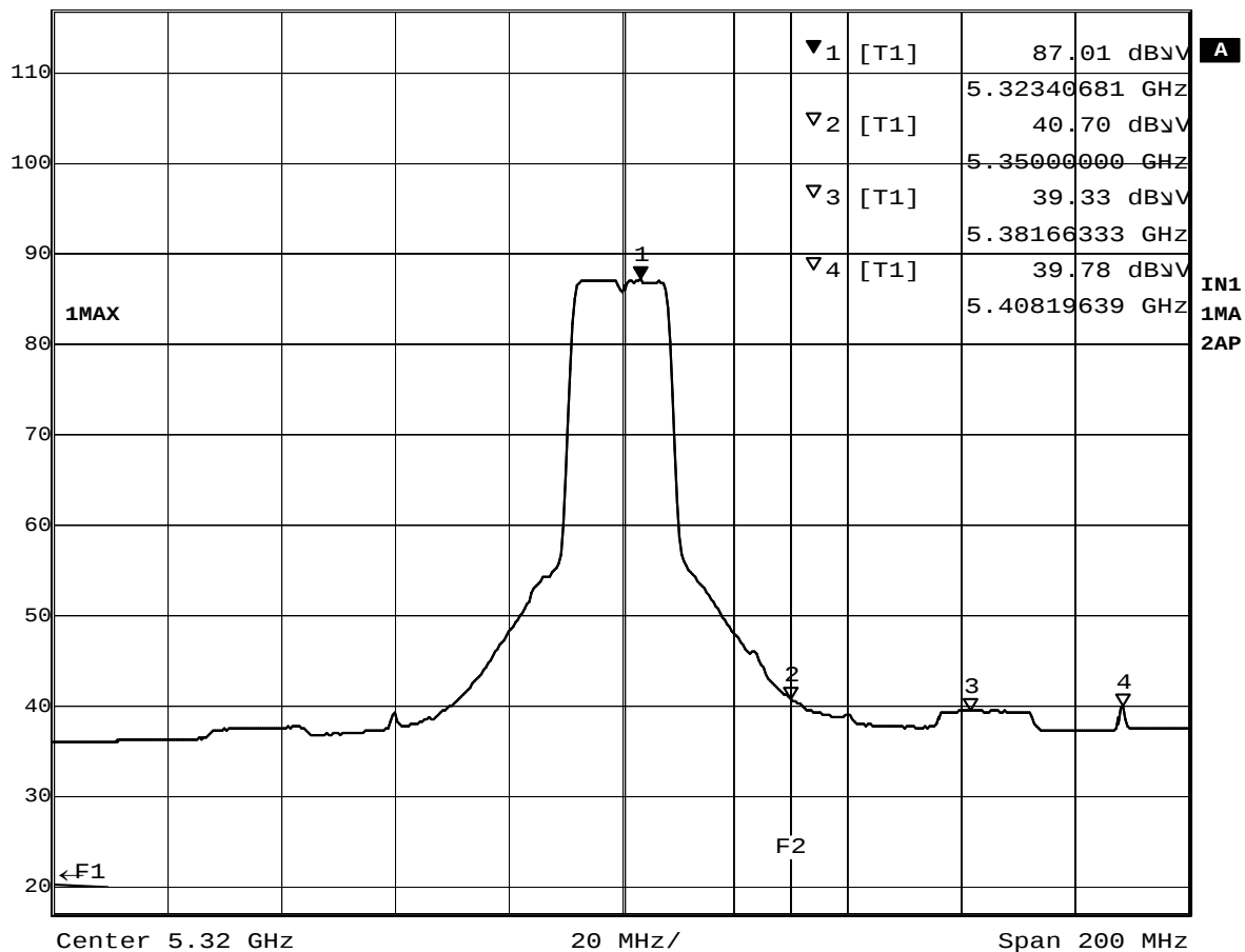
Plot 7-3-2 5320MHz TX mode (Average)
