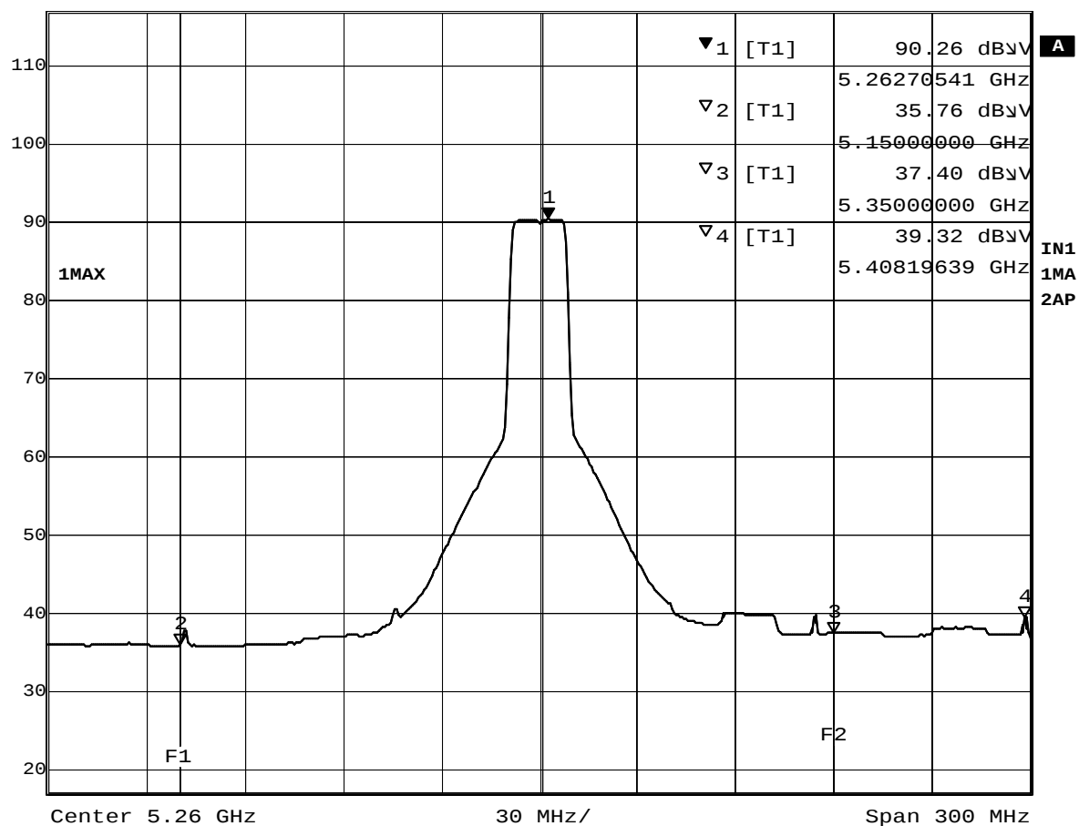
Plot 7-2-2 5260MHz TX mode (Average)
