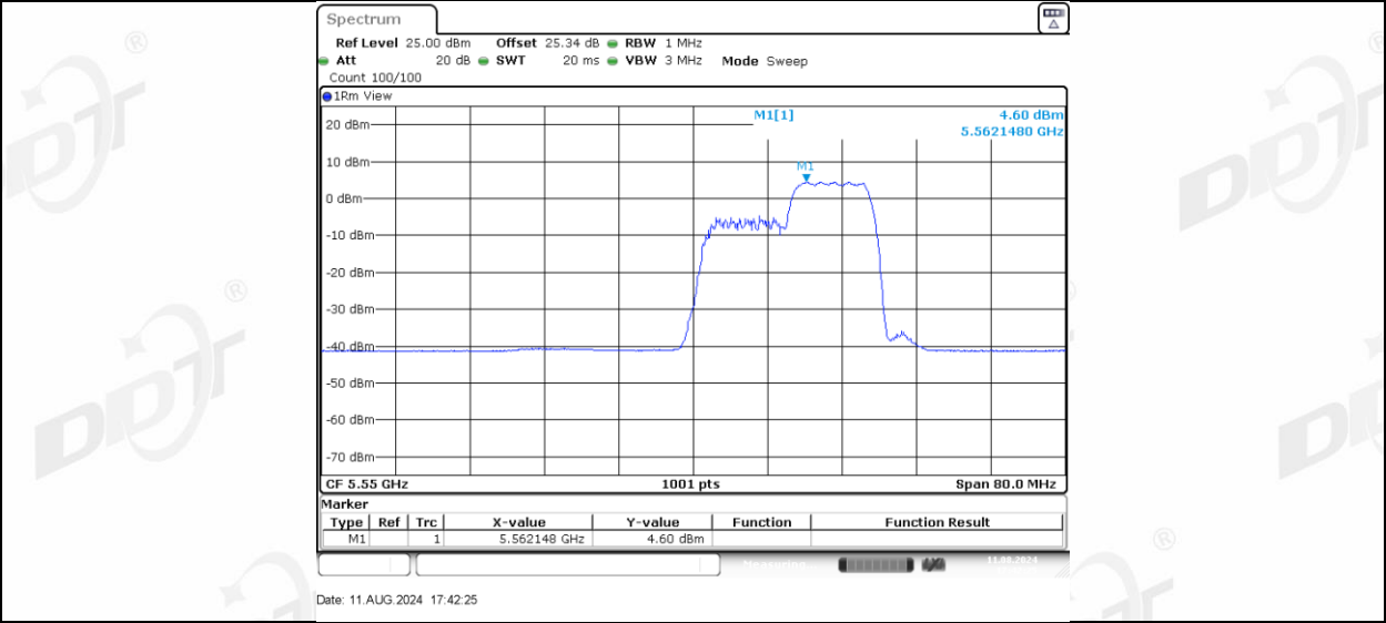
11AX40MIMO_Ant-1_5550_242Tone_RU61
