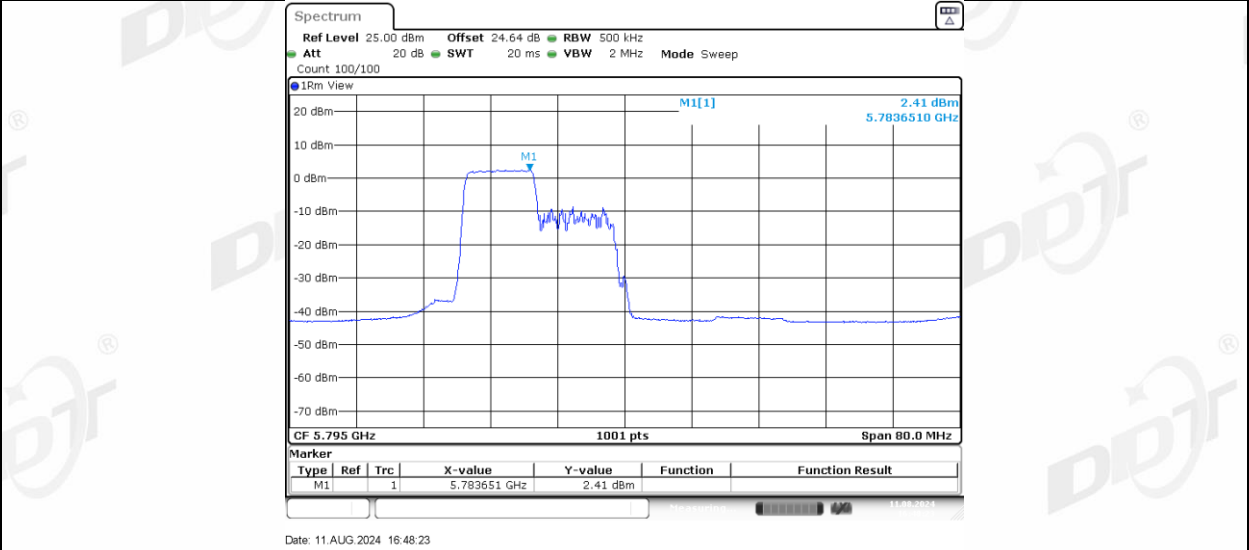
11AX40MIMO_Ant-3_5795_106Tone_RU56
