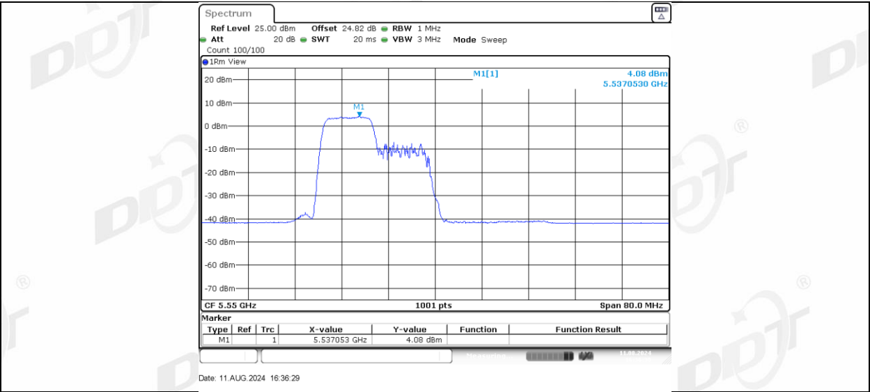
11AX40MIMO_Ant-1_5550_106Tone_RU56
