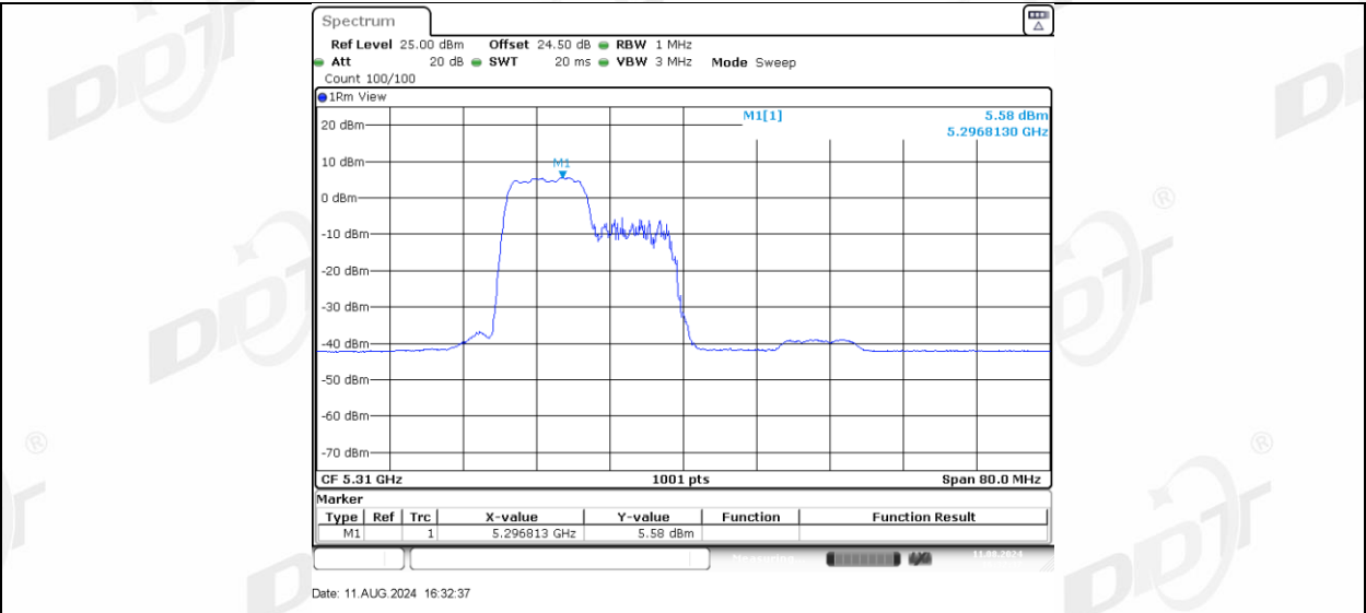
11AX40MIMO_Ant-3_5310_106Tone_RU56
