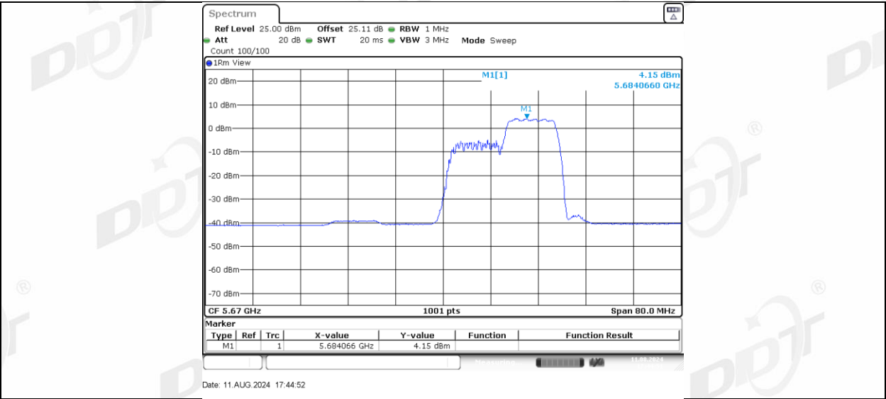
11AX40MIMO_Ant-1_5670_242Tone_RU61
