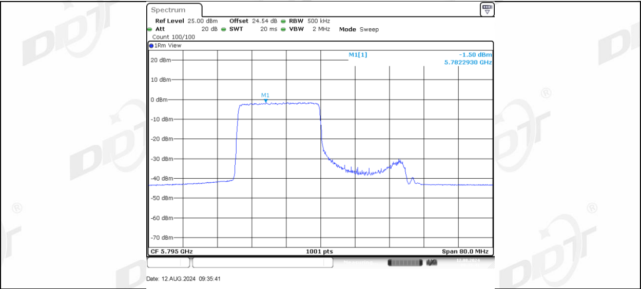
11AX40MIMO_Ant-1_5795_242Tone_RU62
