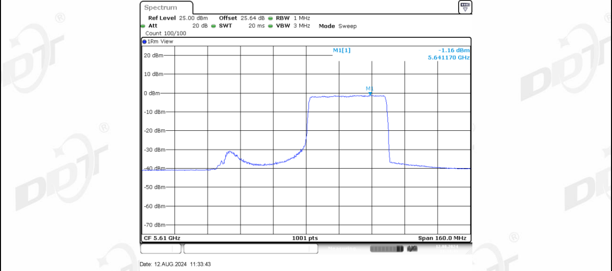
11AX80MIMO_Ant-1_5690_UNII-2C_242Tone_RU61
