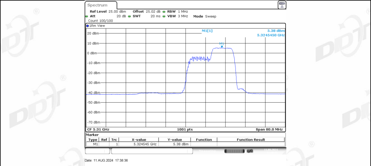
11AX40MIMO_Ant-3_5310_242Tone_RU61
