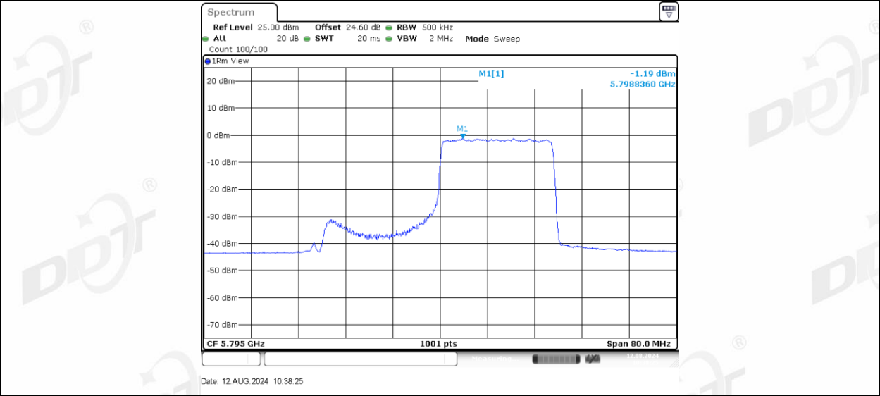
11AX40MIMO_Ant-3_5795_106Tone_RU53
