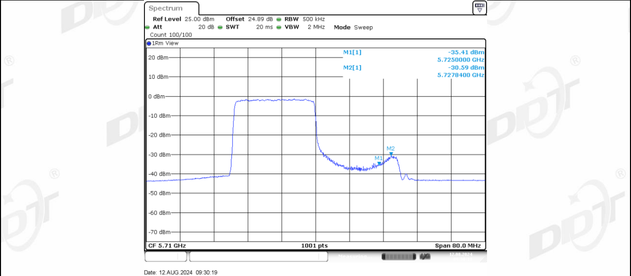
11AX40MIMO_Ant-1_5710_UNII-3_242Tone_RU62
