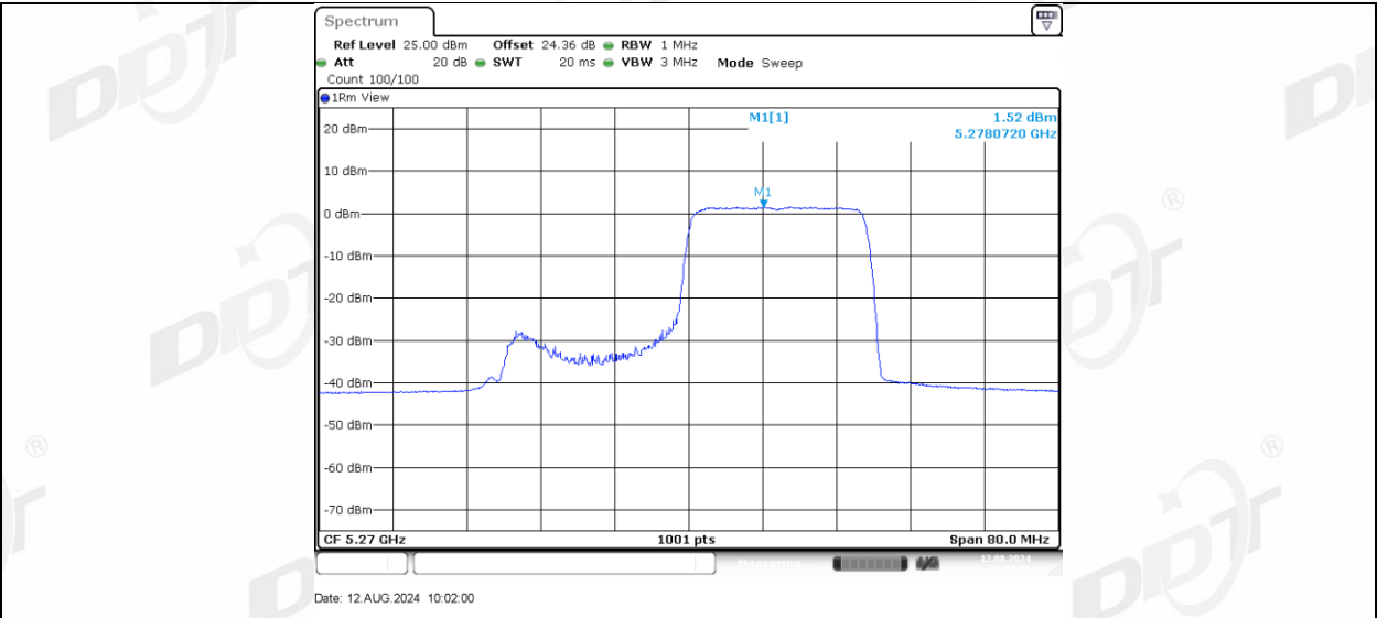
11AX40MIMO_Ant-3_5270_106Tone_RU53
