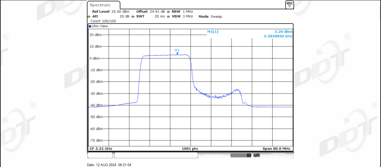
11AX40MIMO_Ant-3_5310_242Tone_RU62
