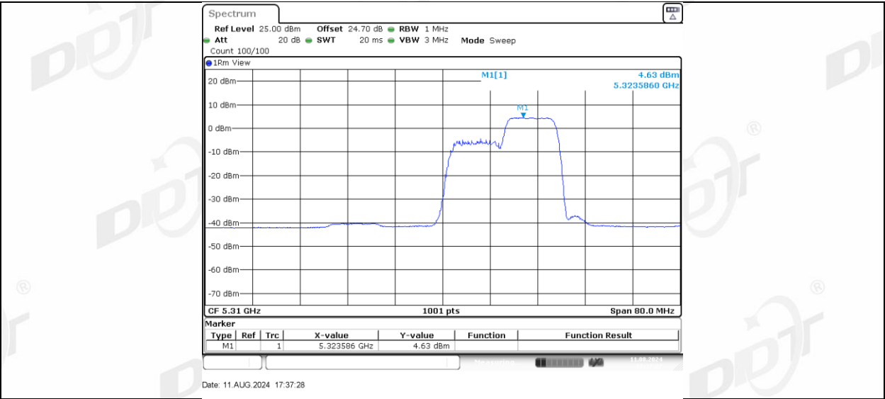
11AX40MIMO_Ant-1_5310_242Tone_RU61
