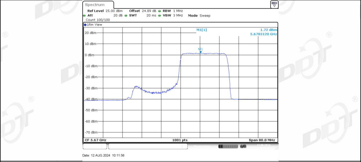
11AX40MIMO_Ant-3_5670_106Tone_RU53
