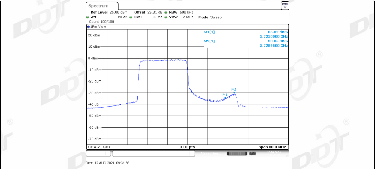
11AX40MIMO_Ant-3_5710_UNII-3_242Tone_RU62
