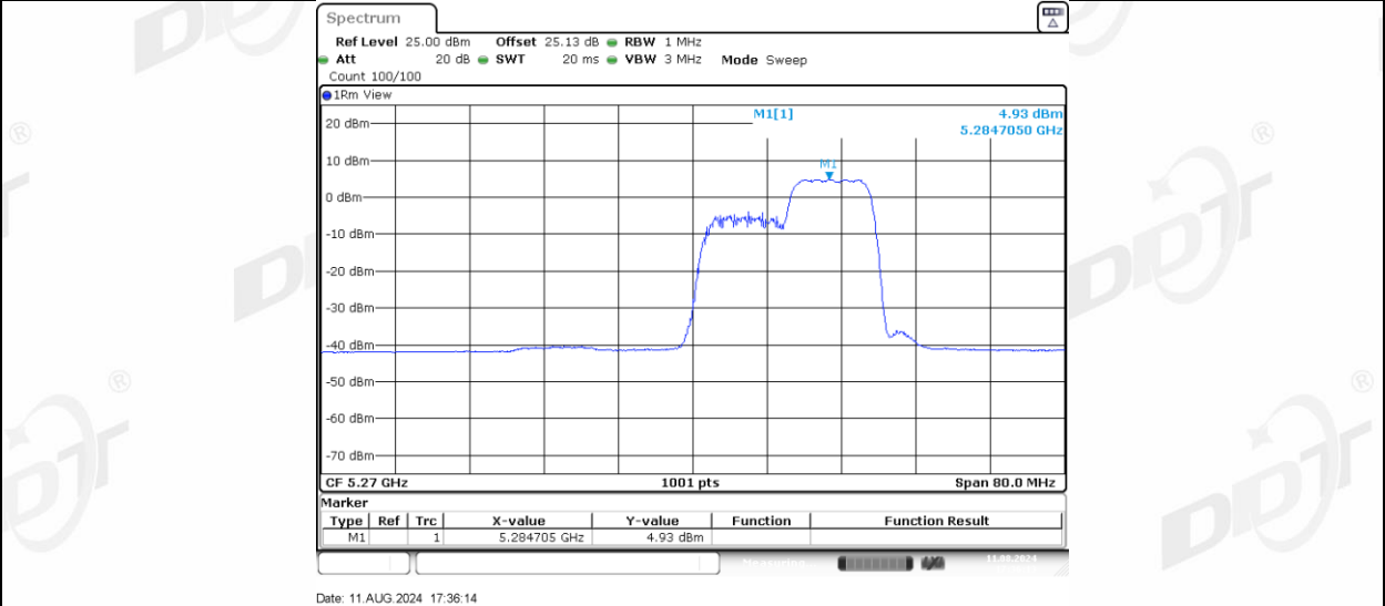
11AX40MIMO_Ant-3_5270_242Tone_RU61
