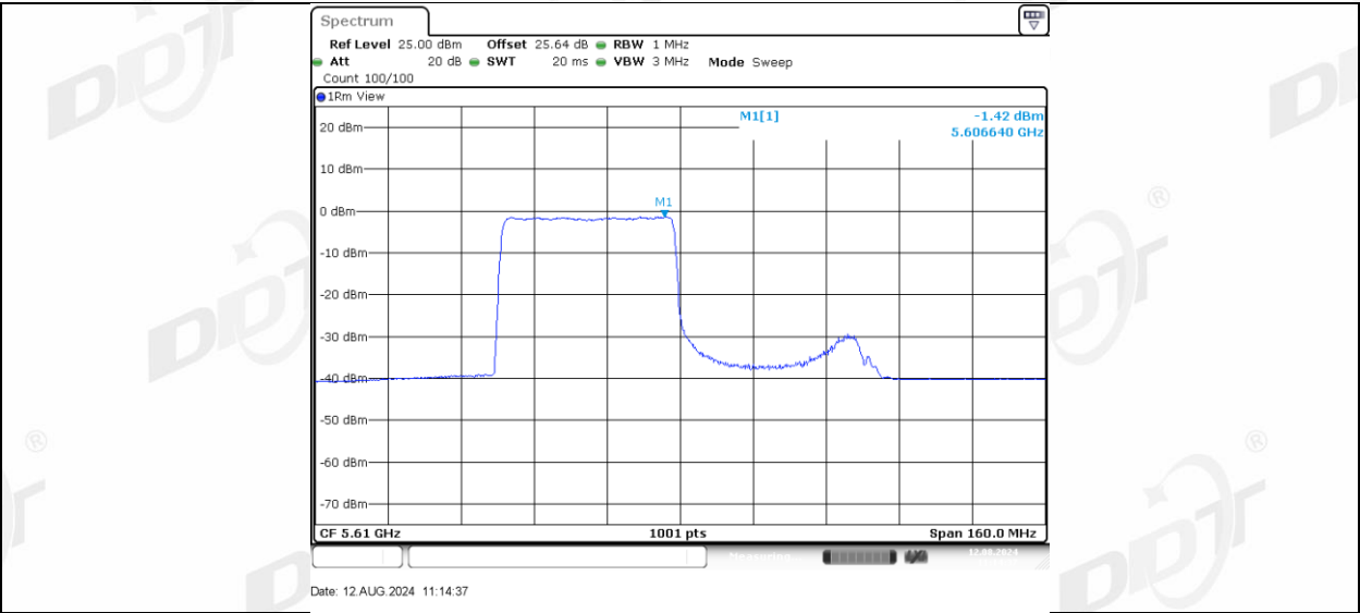
11AX80MIMO_Ant-3_5610_484Tone_RU66
