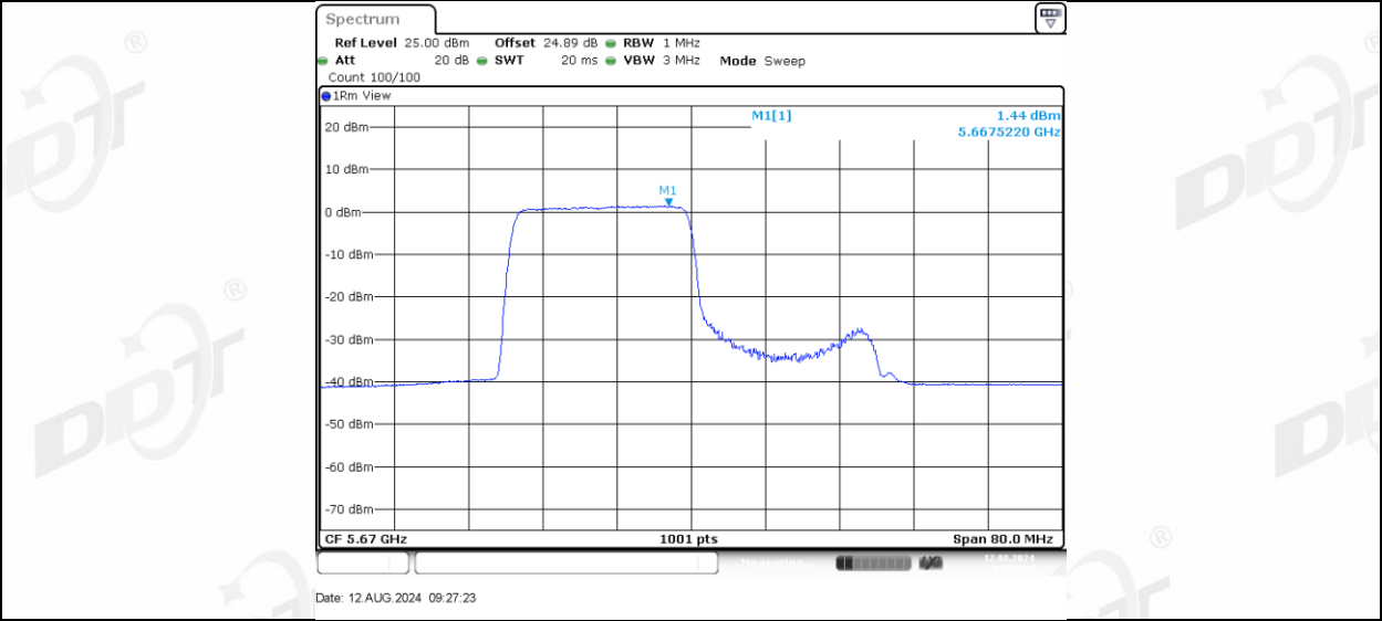
11AX40MIMO_Ant-1_5670_242Tone_RU62
