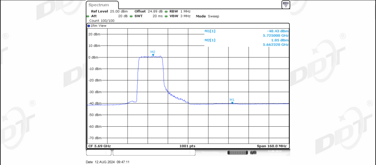
11AX80MIMO_Ant-1_5690_UNII-2C_242Tone_RU64
