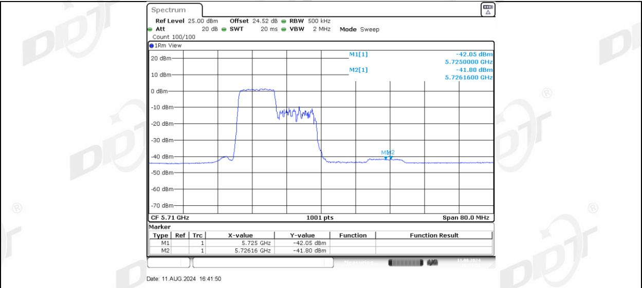
11AX40MIMO_Ant-1_5710_UNII-3_106Tone_RU56
