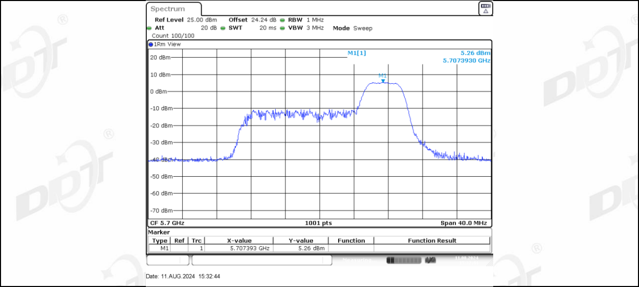
11AX20MIMO_Ant-1_5700_106Tone_RU53
