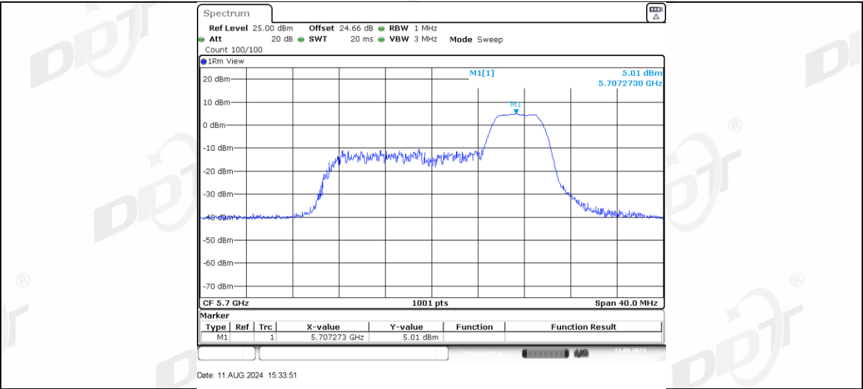
11AX20MIMO_Ant-3_5700_106Tone_RU53
