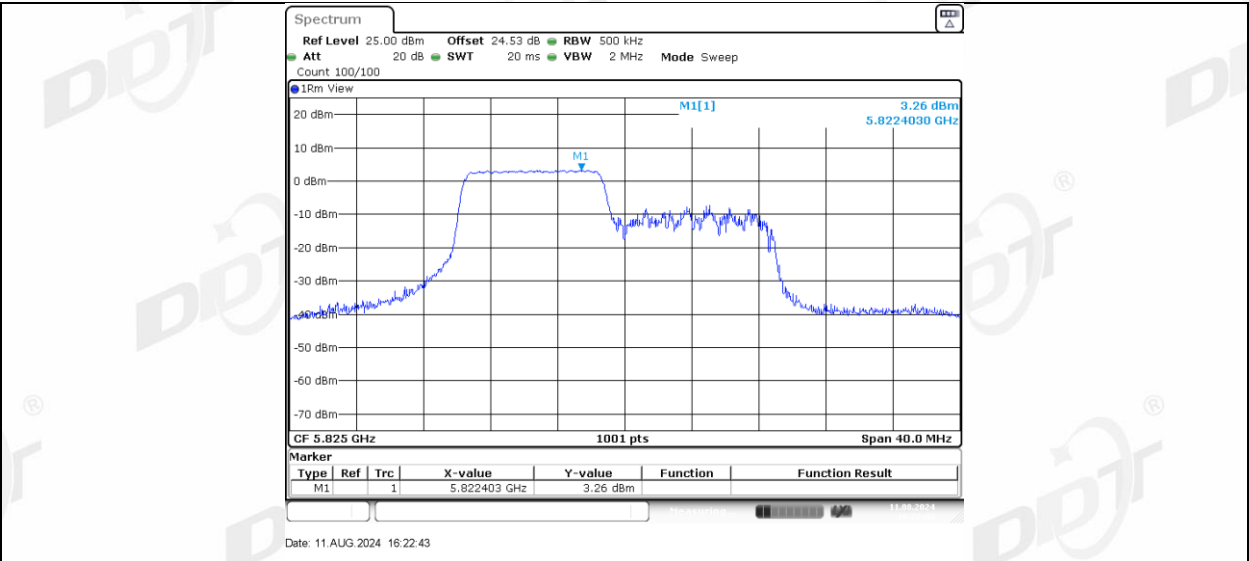
11AX20MIMO_Ant-3_5825_106Tone_RU54
