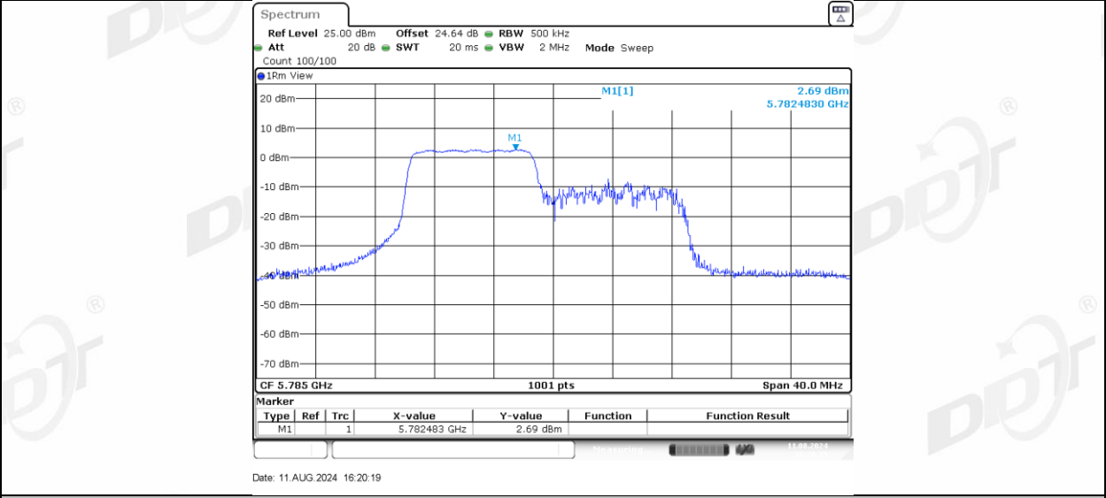
11AX20MIMO_Ant-3_5785_106Tone_RU54
