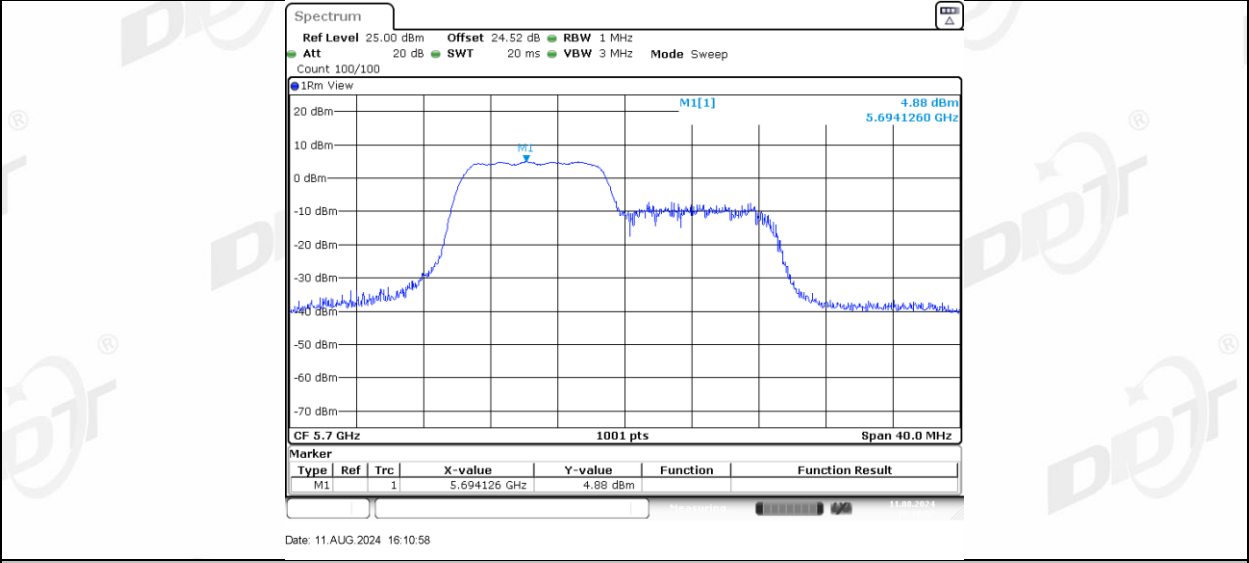
11AX20MIMO_Ant-1_5700_106Tone_RU54
