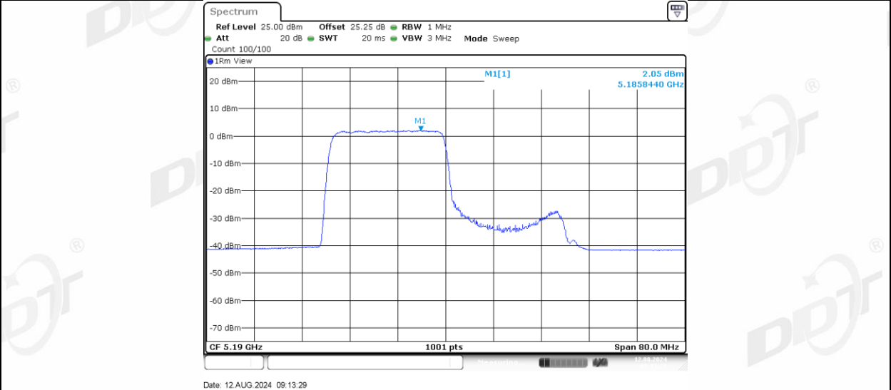
11AX40MIMO_Ant-3_5190_242Tone_RU62
