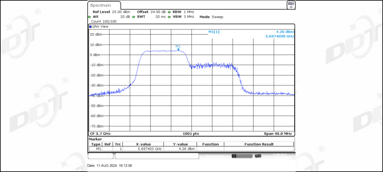
11AX20MIMO_Ant-3_5700_106Tone_RU54
