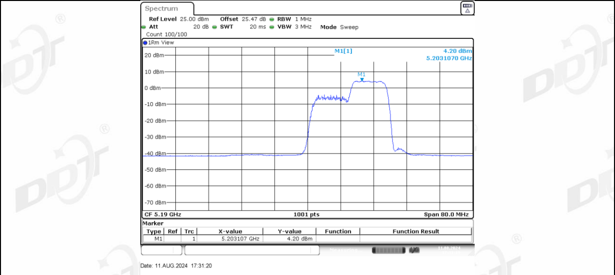
11AX40MIMO_Ant-3_5190_242Tone_RU61
