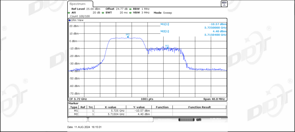
11AX20MIMO_Ant-3_5720_UNII-2C_106Tone_RU54
