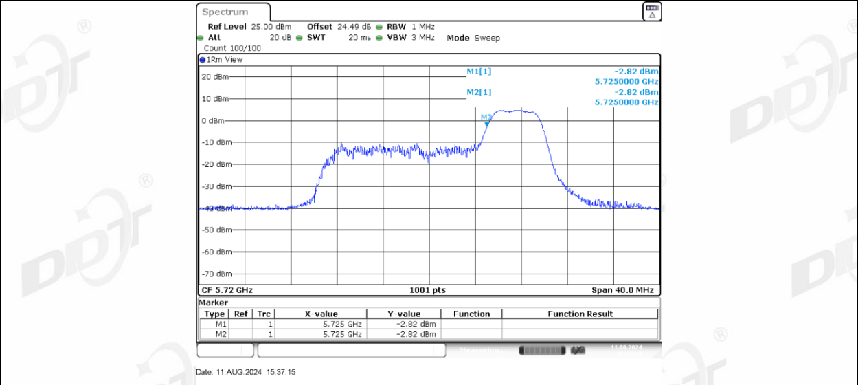
11AX20MIMO_Ant-3_5720_UNII-2C_106Tone_RU53
