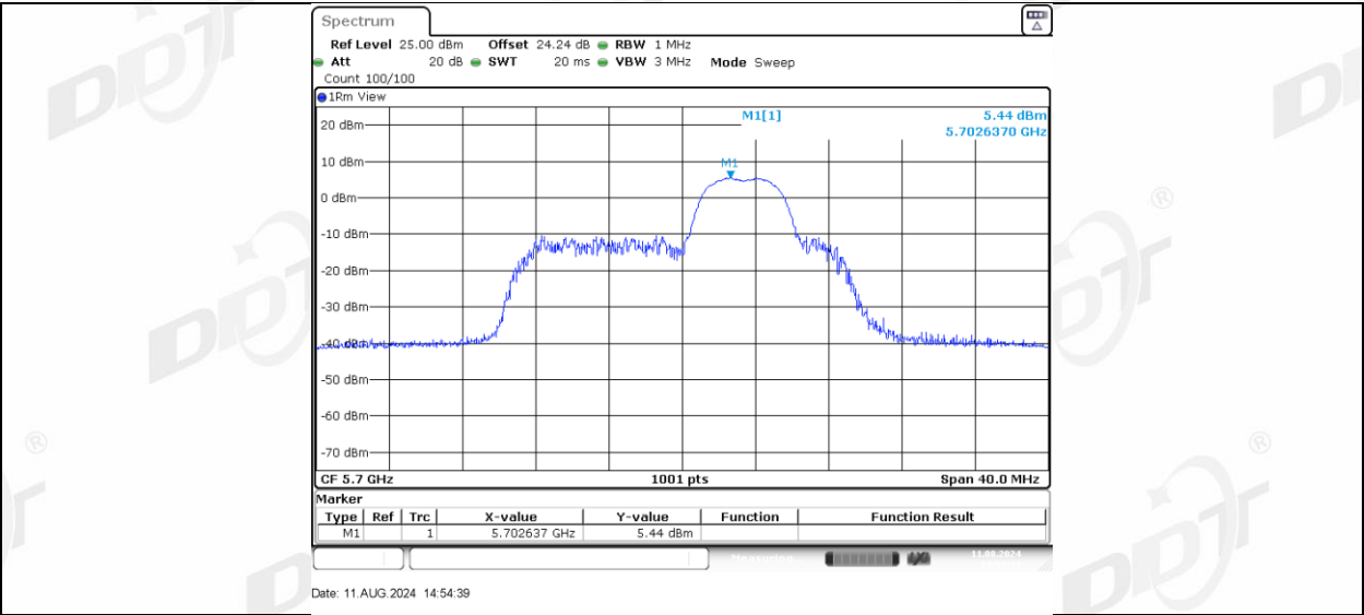
11AX20MIMO_Ant-1_5700_52Tone_RU40
