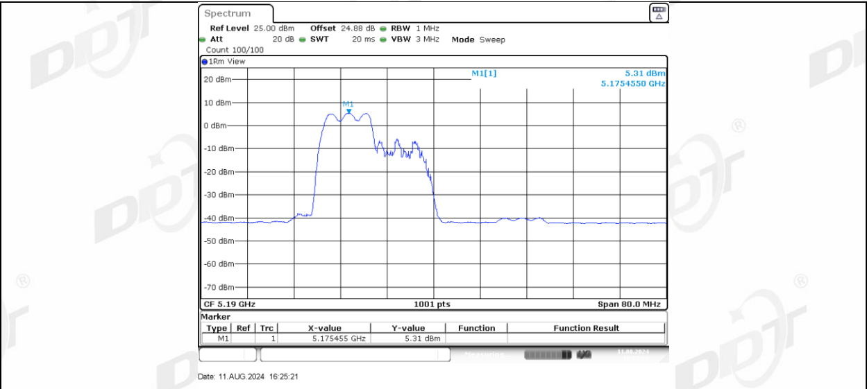
11AX40MIMO_Ant-3_5190_106Tone_RU56
