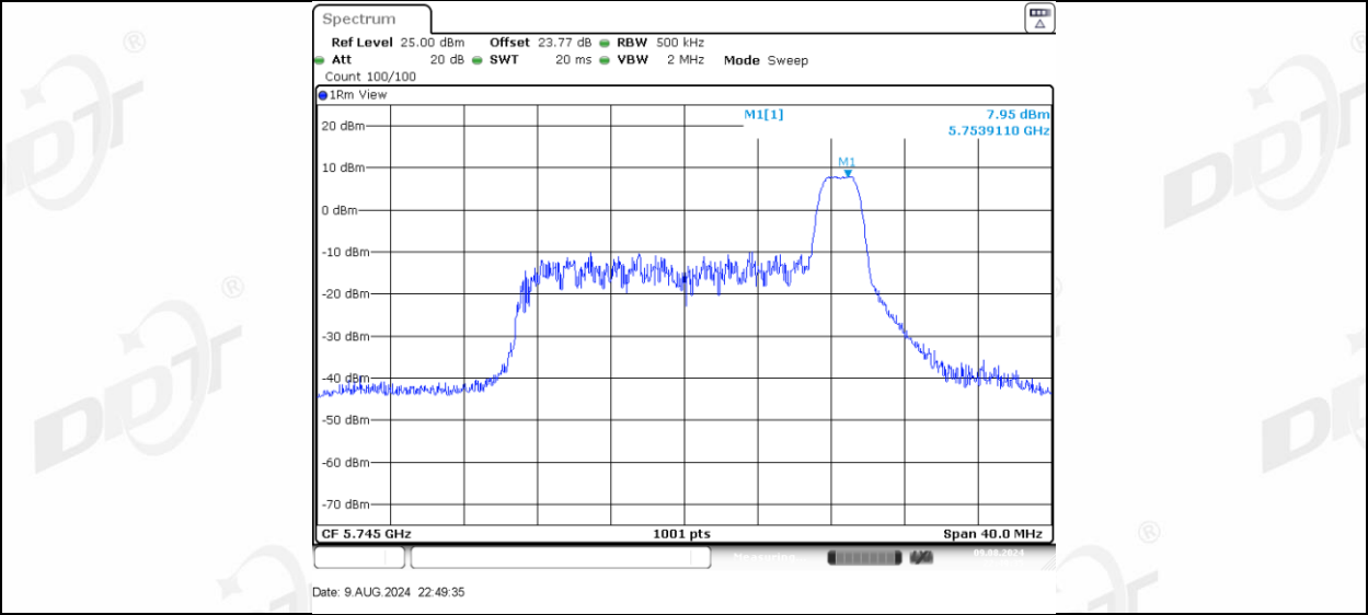
11AX20MIMO_Ant-1_5745_52Tone_RU37
