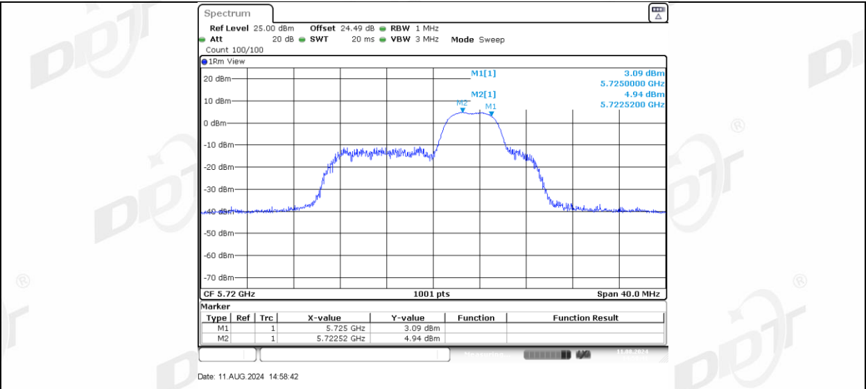
11AX20MIMO_Ant-3_5720_UNII-2C_52Tone_RU40
