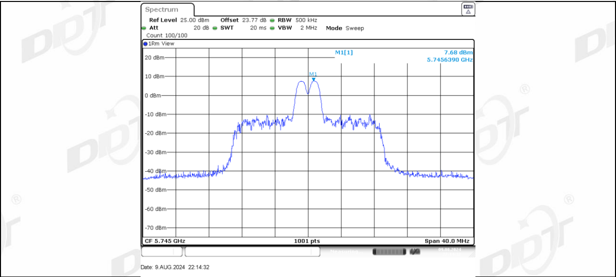
11AX20MIMO_Ant-1_5745_26Tone_RU8
