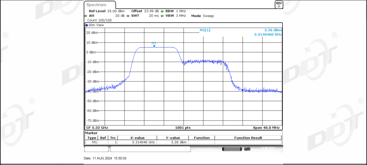
11AX20MIMO_Ant-1_5320_106Tone_RU54
