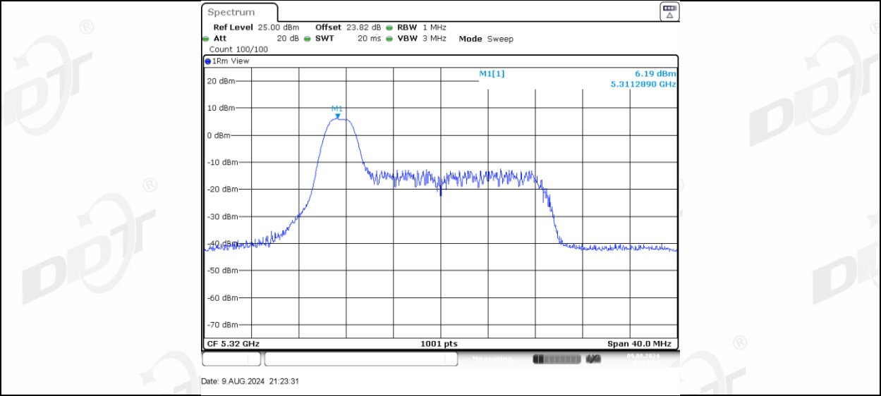
11AX20MIMO Ant-3 5320 26Tone_RU4
