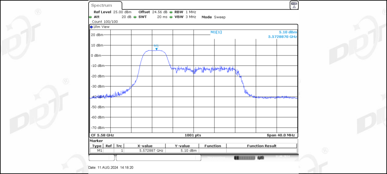
11AX20MIMO_Ant-1_5580_52Tone_RU39
