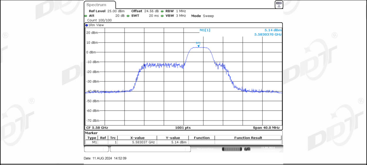
11AX20MIMO_Ant-1_5580_52Tone_RU40
