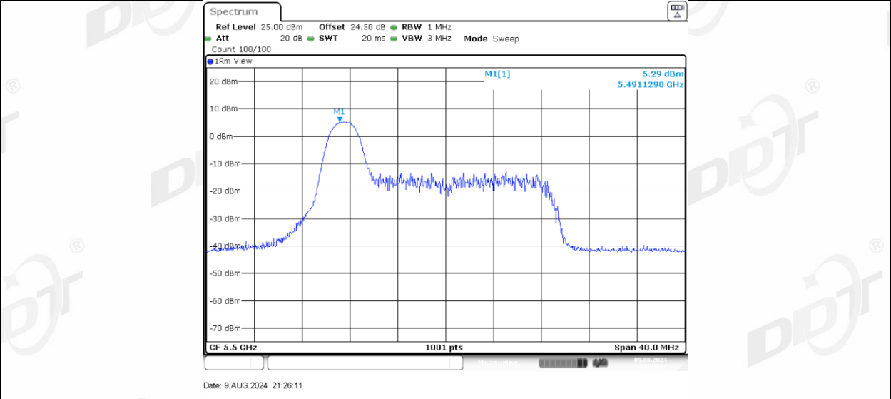
11AX20MIMO Ant-3 5500 26Tone RU4
