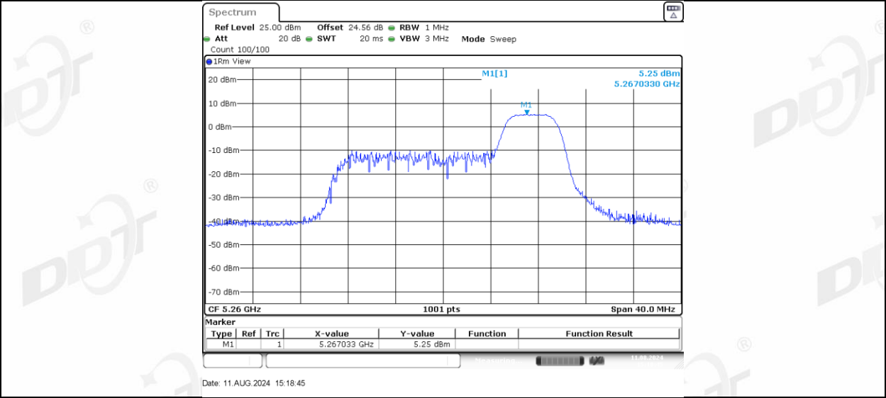
11AX20MIMO_Ant-3_5260_106Tone_RU53
