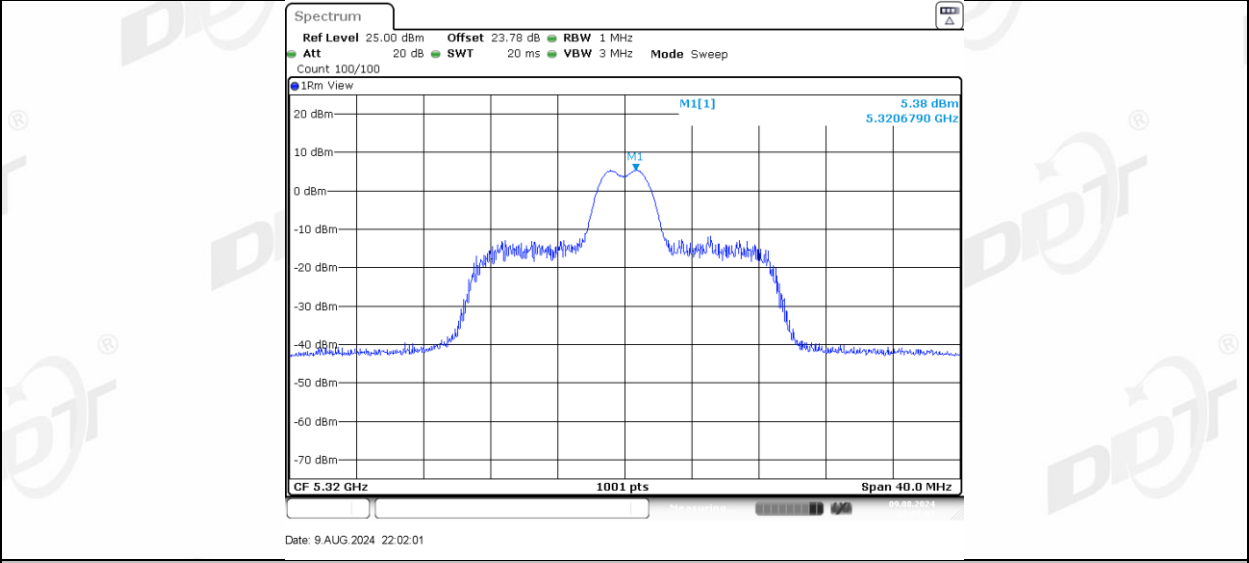
11AX20MIMO Ant-3 5320 26Tone_RU8
