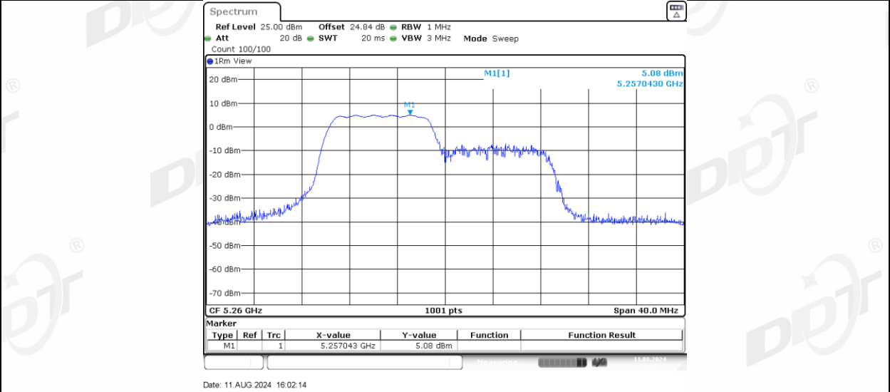
11AX20MIMO_Ant-3_5260_106Tone_RU54
