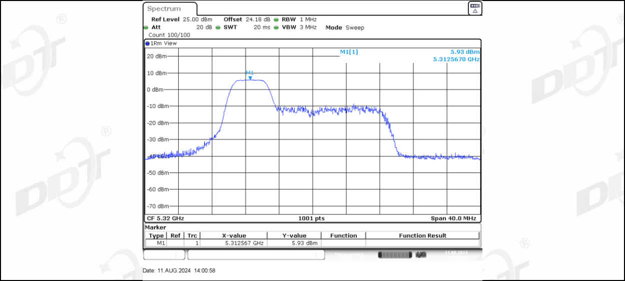
11AX20MIMO_Ant-3_5320_52Tone_RU39
