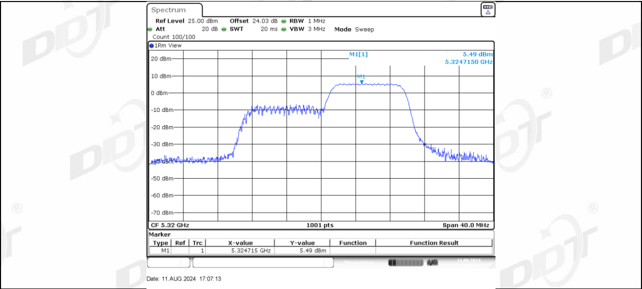
11AX20MIMO Ant-3 5320 26Tone_RU0
