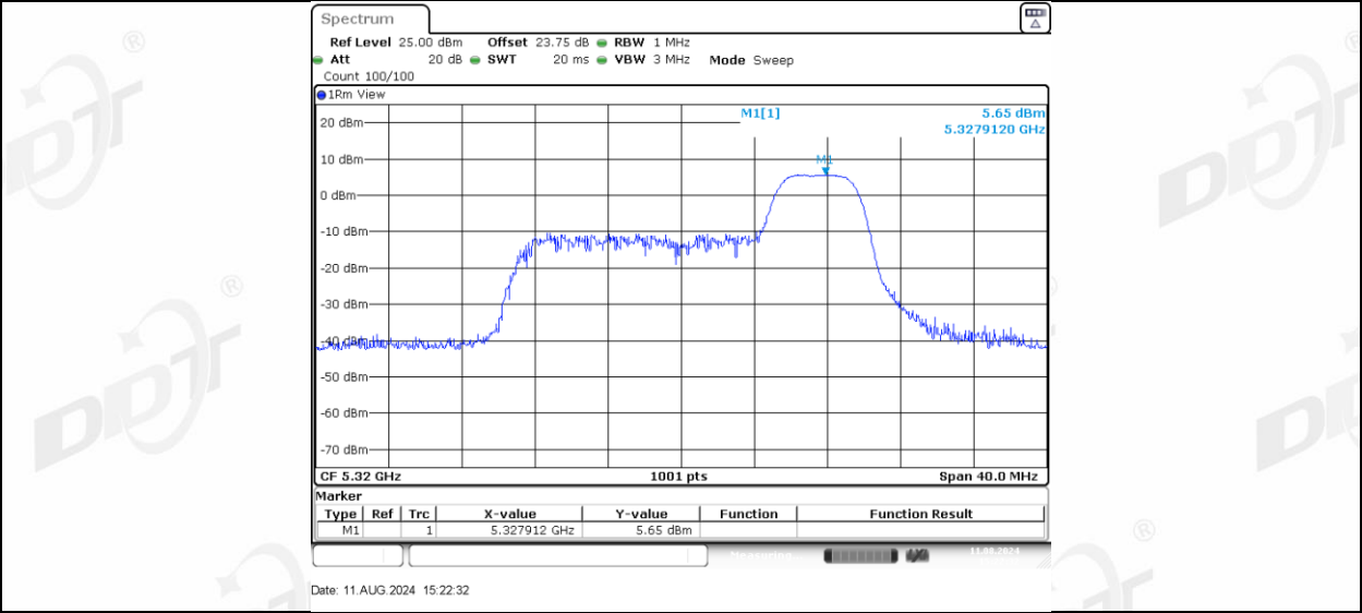
11AX20MIMO_Ant-1_5320_106Tone_RU53
