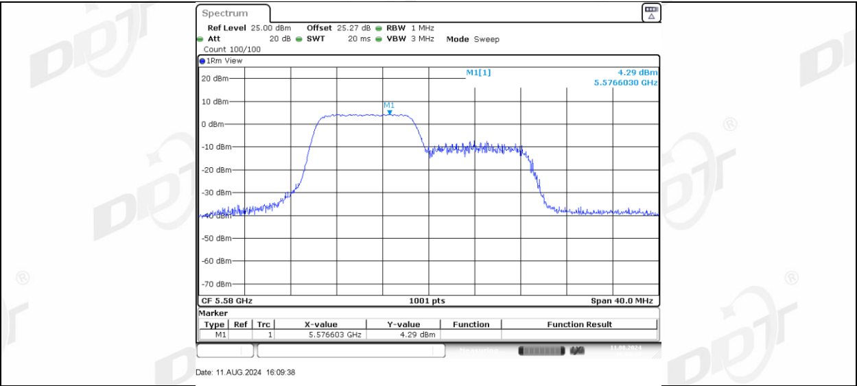
11AX20MIMO Ant-3 5580 106Tone RU54
