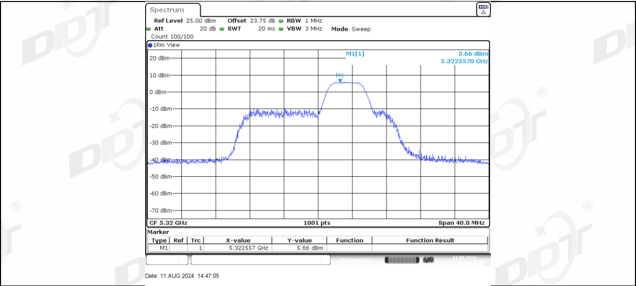
11AX20MIMO_Ant-1_5320_52Tone_RU40
