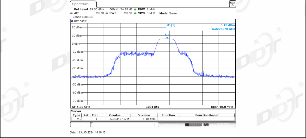
11AX20MIMO_Ant-3_5320_52Tone_RU40
