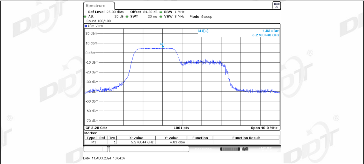
11AX20MIMO Ant-3 5280 106Tone RU54
