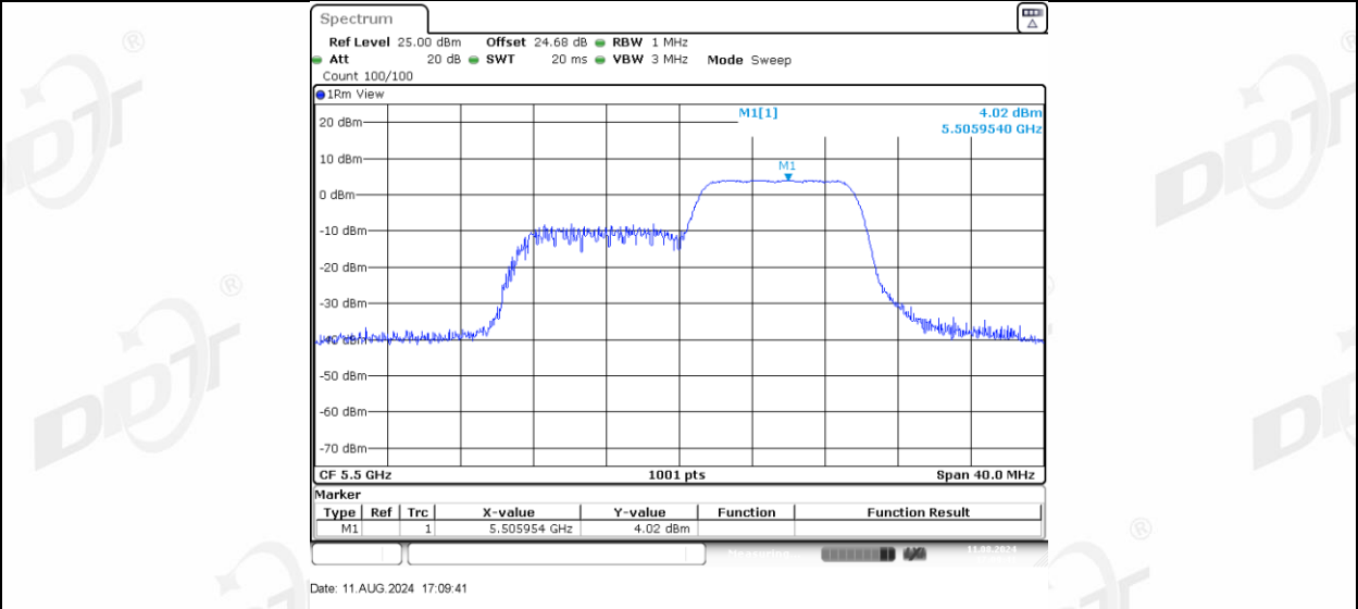
11AX20MIMO Ant-3 5500 26Tone RU0
