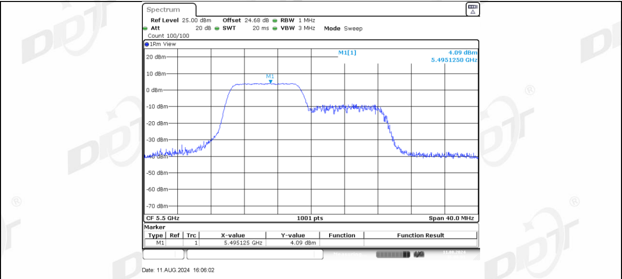
11AX20MIMO Ant-1 5500 106Tone RU54
