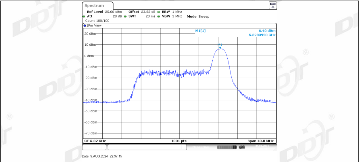
11AX20MIMO_Ant-3_5320_52Tone_RU37
