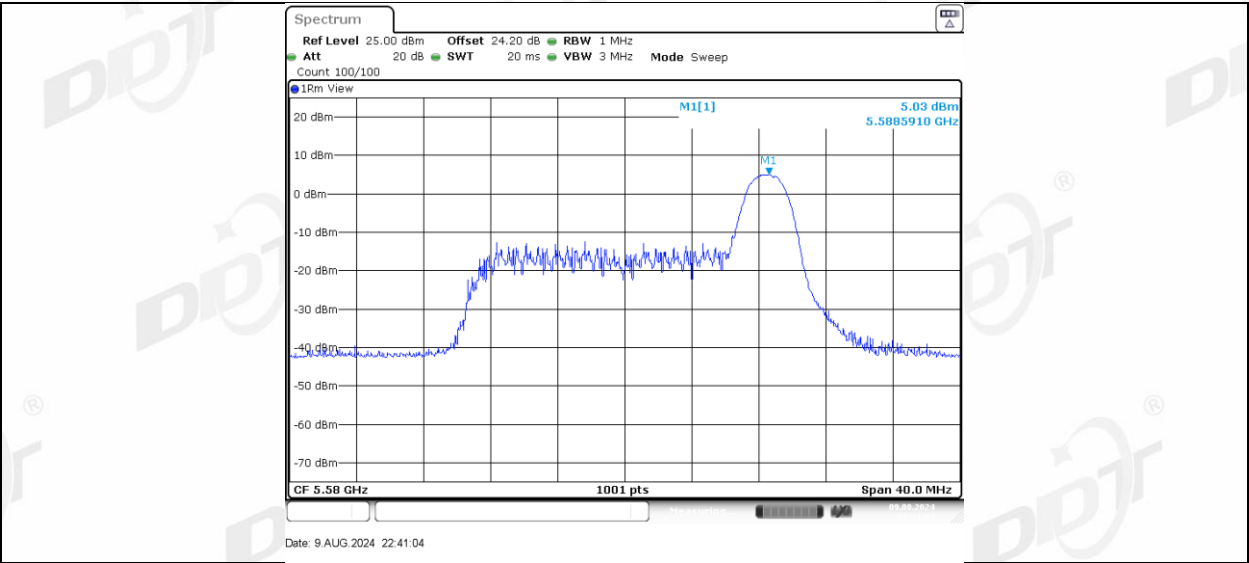
11AX20MIMO_Ant-1_5580_52Tone_RU37
