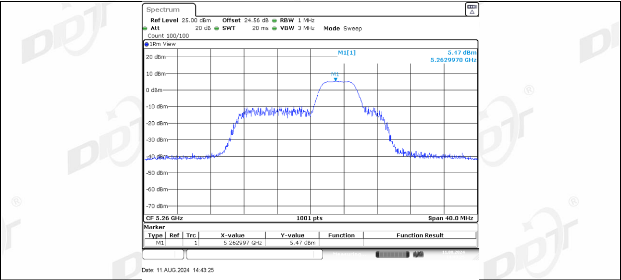
11AX20MIMO_Ant-3_5260_52Tone_RU40
