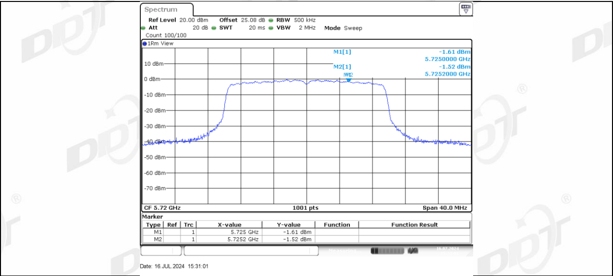
11AX20MIMO_Ant-3_5720_UNII-3
