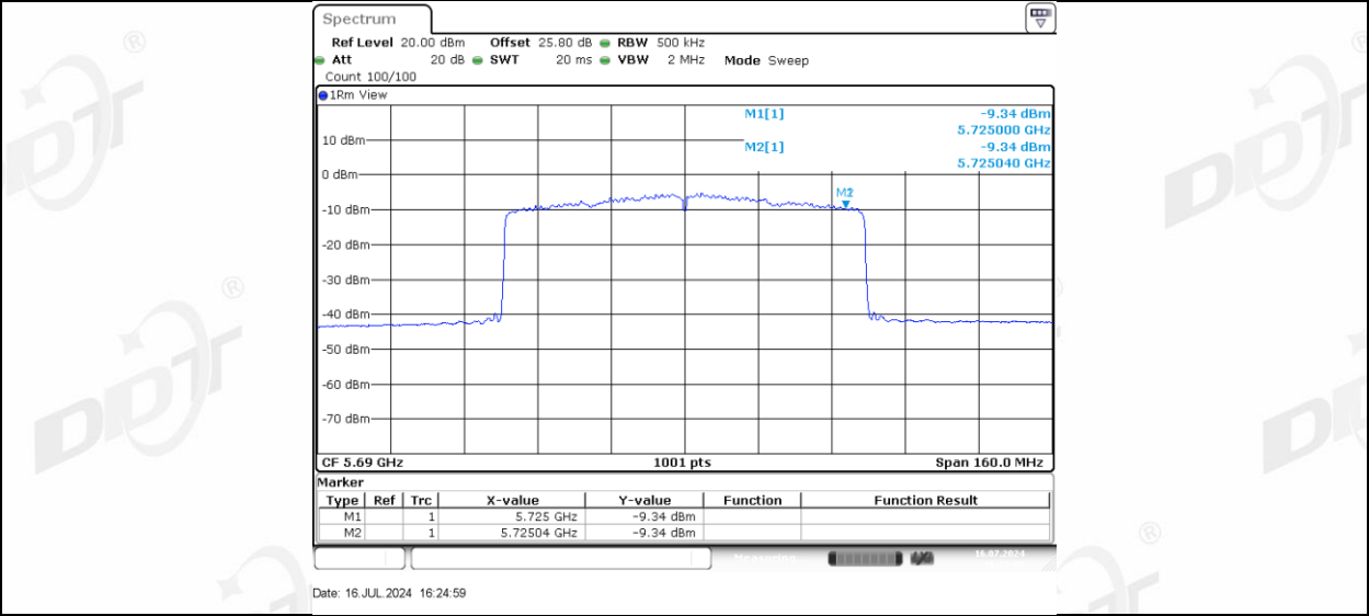
11AX80MIMO_Ant-3_5690_UNII-3
