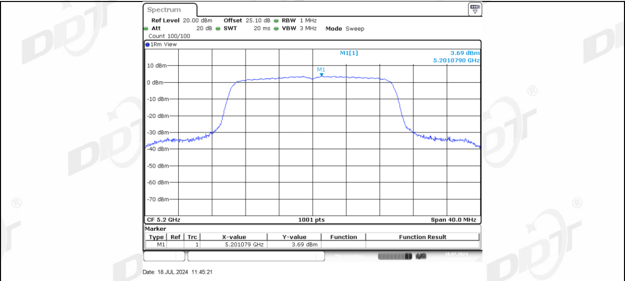
11AX20MIMO_Ant-3_5200
