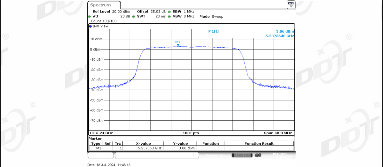
11AX20MIMO_Ant-3_5240
