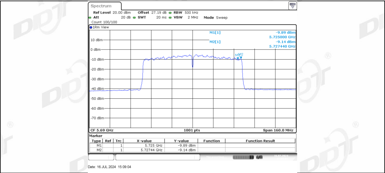
11AC80MIMO_Ant-3_5690_UNII-3
