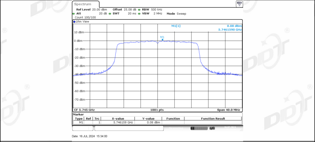
11AX20MIMO_Ant-3_5745
