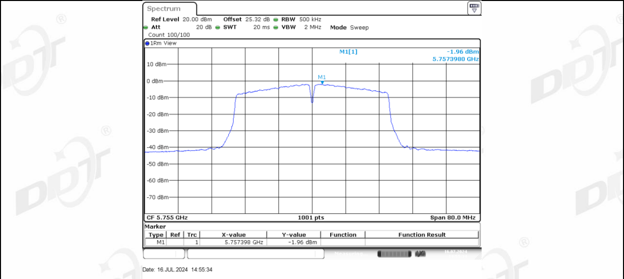
11AC40MIMO_Ant-3_5755
