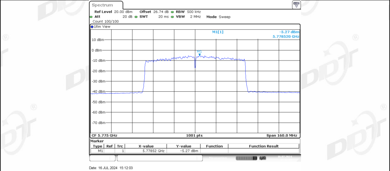
11AC80MIMO_Ant-3_5775
