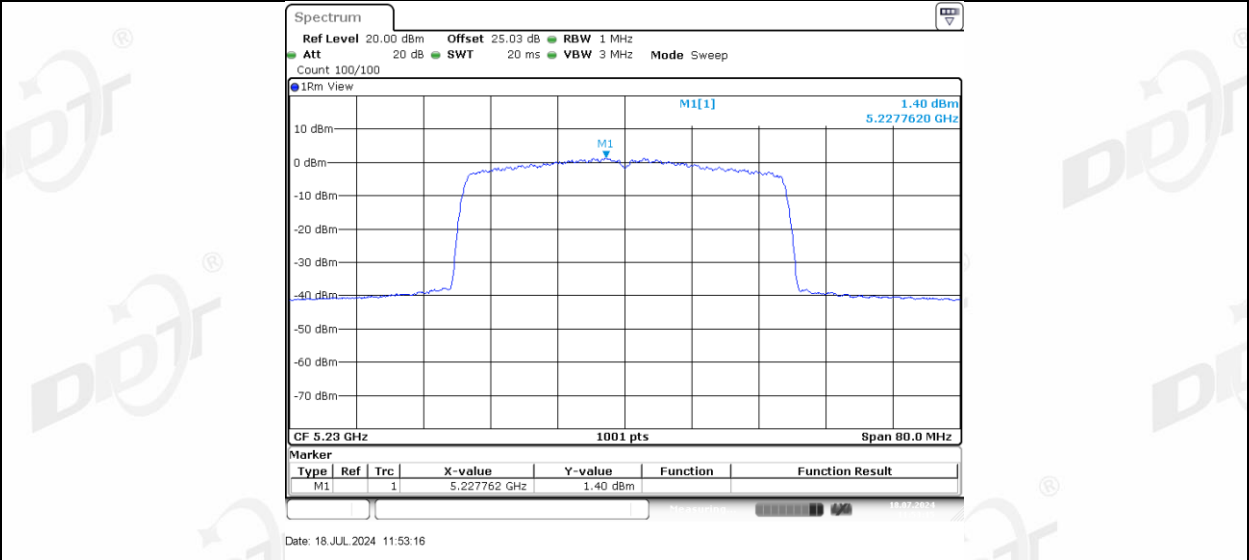
11AX40MIMO Ant-3_5230
