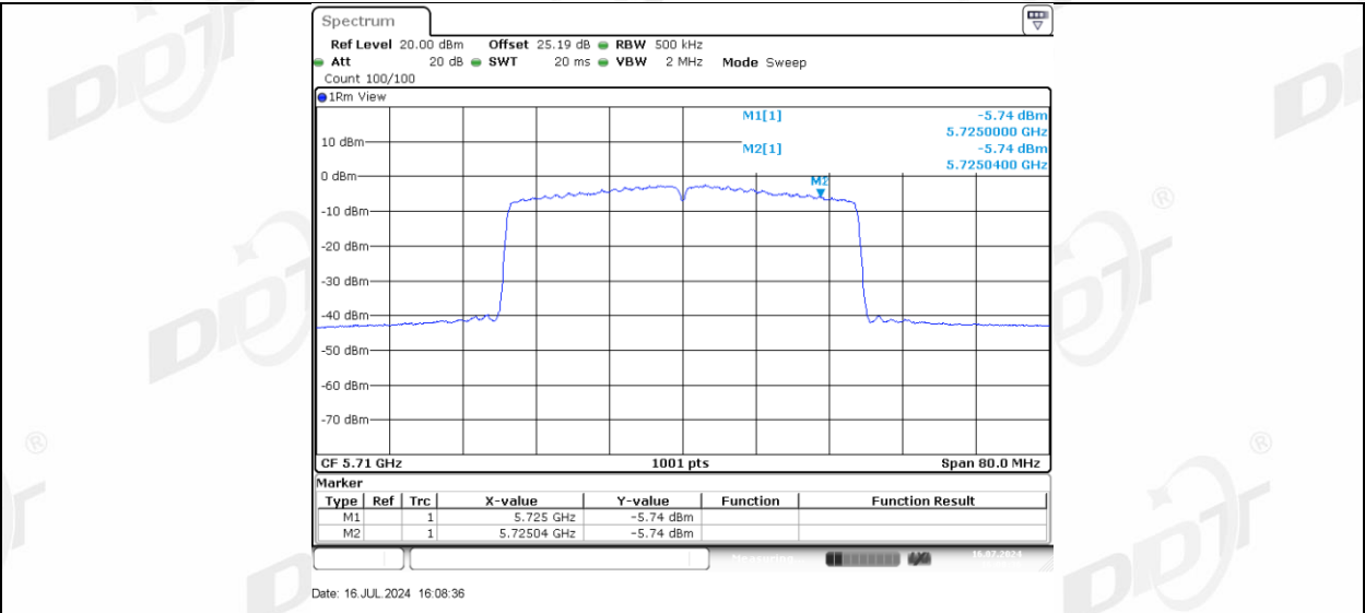
11AX40MIMO_Ant-3_5710_UNII-3
