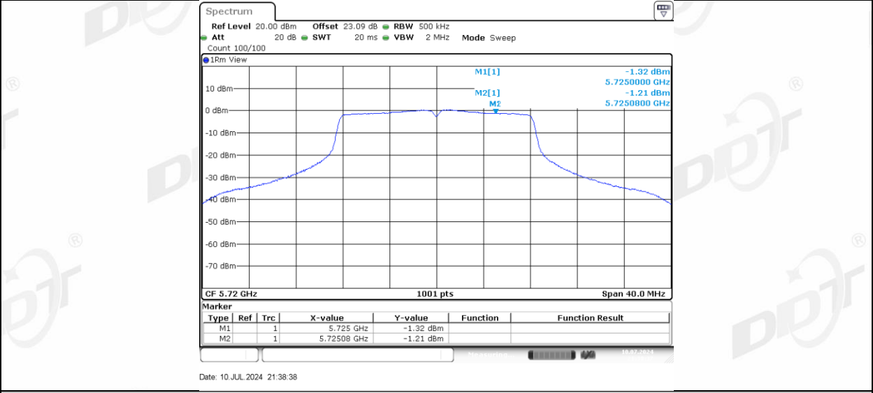
11A-CDD_Ant-3_5720_UNII-3
