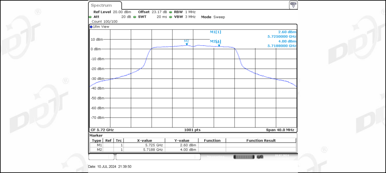
11A-CDD_Ant-1_5720_UNII-3
