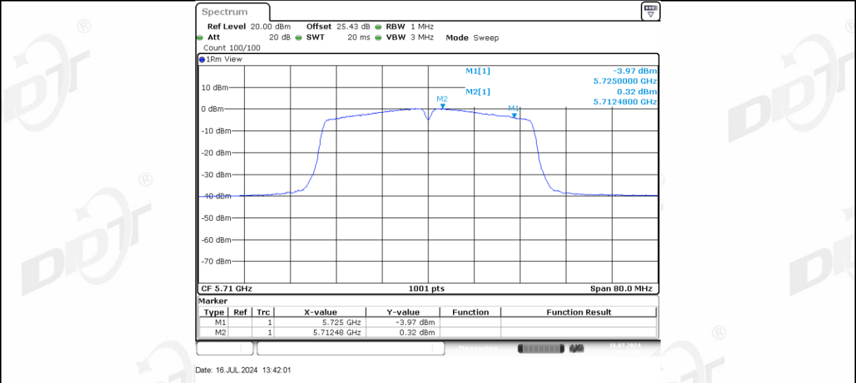
11N40MIMO_Ant-3_5710_UNII-2C
