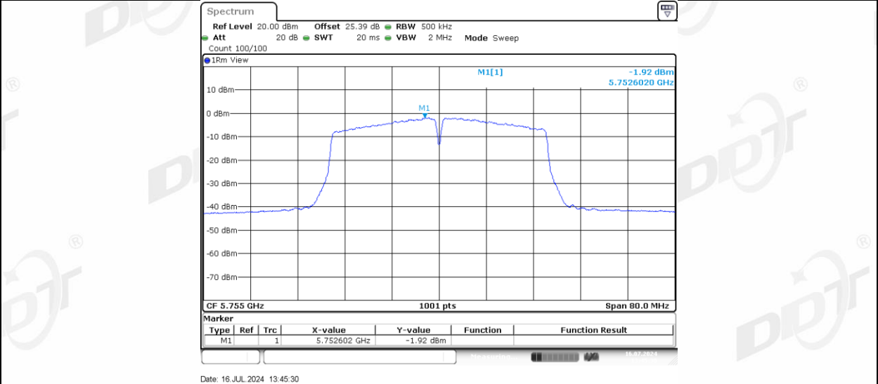
11N40MIMO_Ant-3_5755
