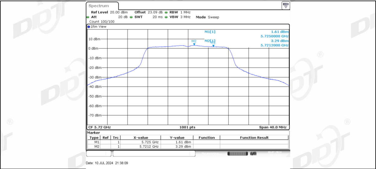
11A-CDD_Ant-3_5720_UNII-2C
