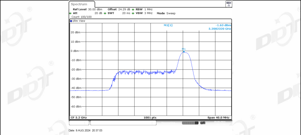
11AX20MIMO Ant-3 5200_52Tone_RU37
