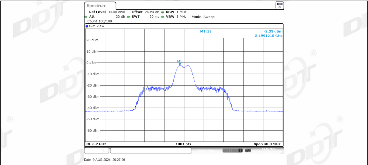
11AX20MIMO Ant-3 5200_26Tone_RU8
