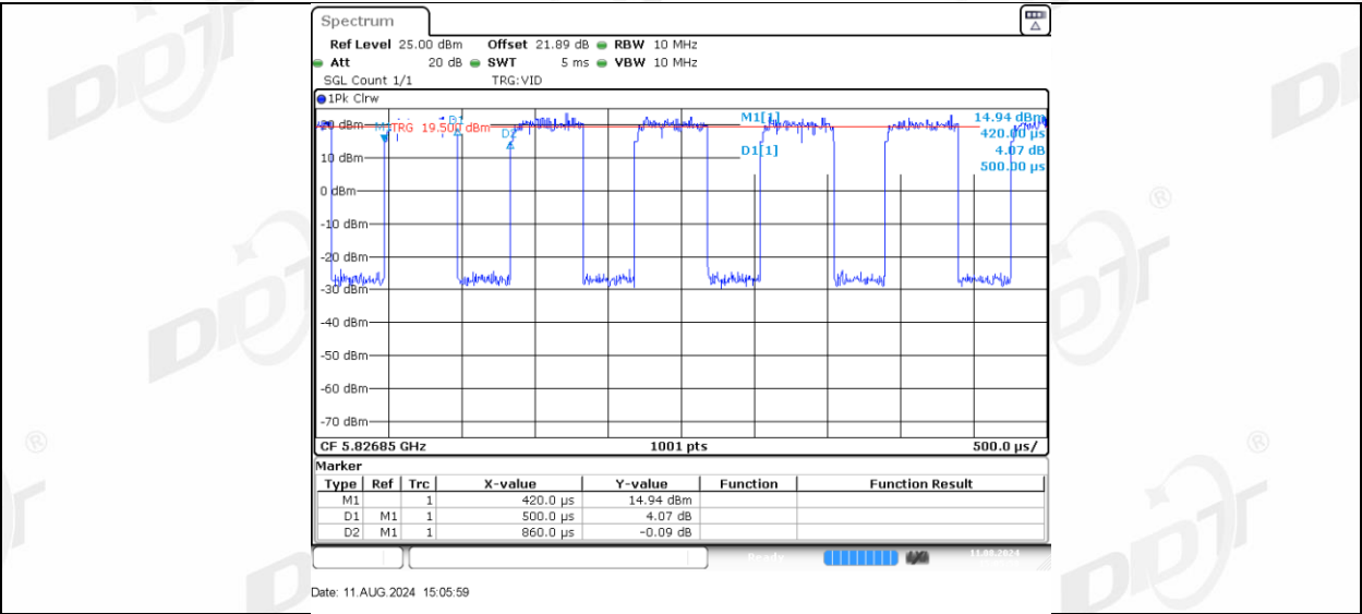
11AX20MIMO_Ant-3_5825_52Tone_RU40
