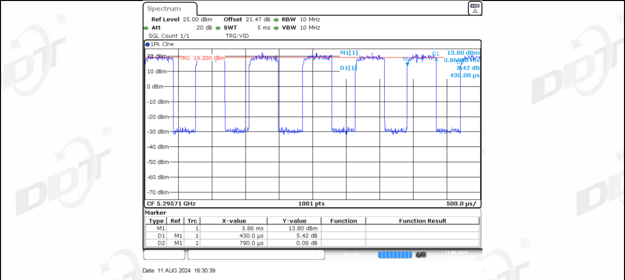
11AX40MIMO_Ant-1_5310_106Tone_RU56
