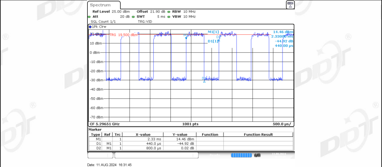
11AX40MIMO_Ant-3_5310_106Tone_RU56
