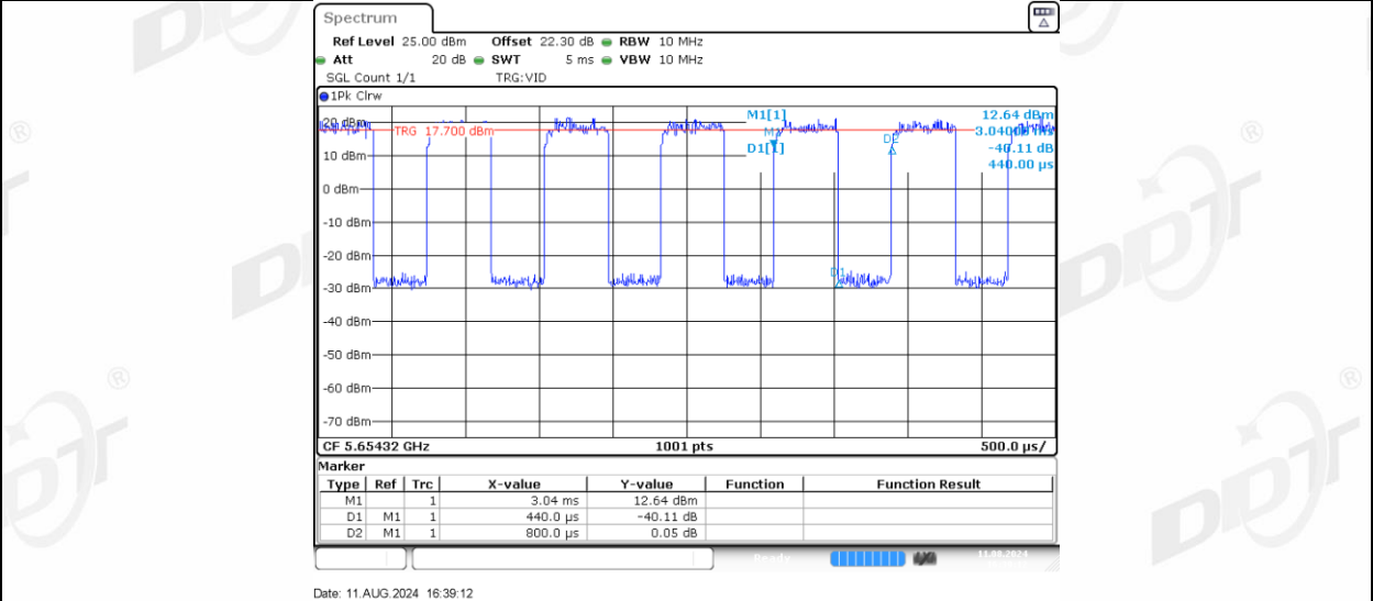
11AX40MIMO_Ant-3_5670_106Tone_RU56
