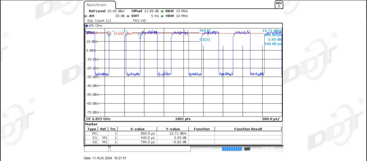
11AX20MIMO_Ant-3_5825_106Tone_RU54
