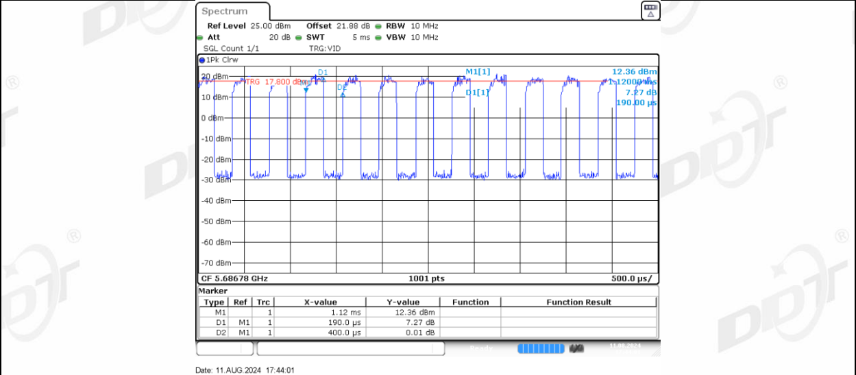
11AX40MIMO_Ant-1_5670_242Tone_RU61
