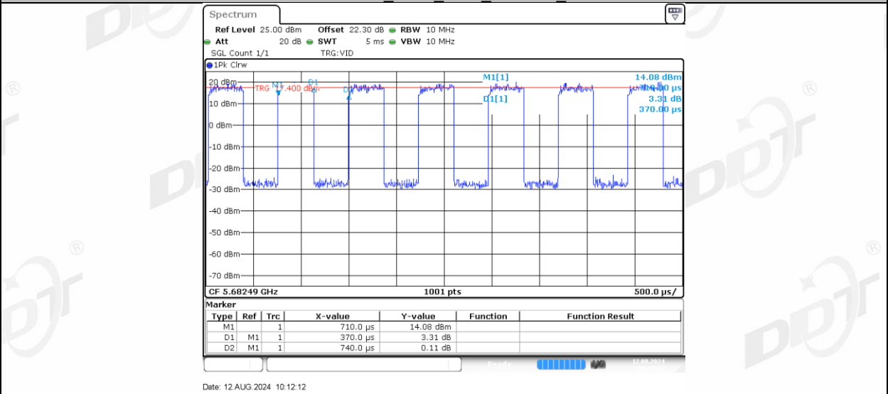
11AX40MIMO_Ant-1_5710_106Tone_RU53
