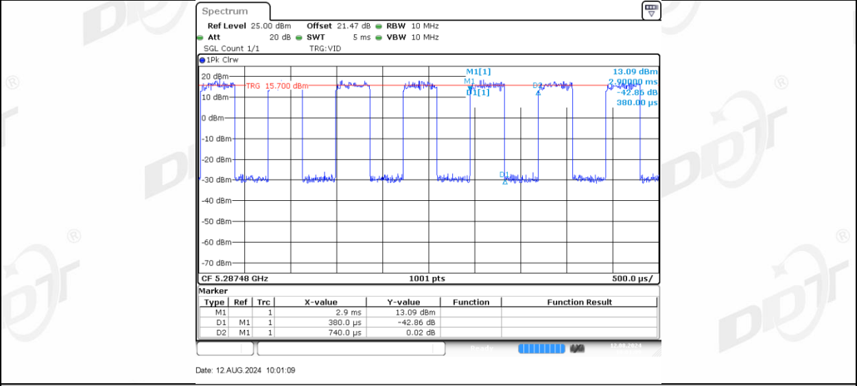
11AX40MIMO_Ant-3_5270_106Tone_RU53
