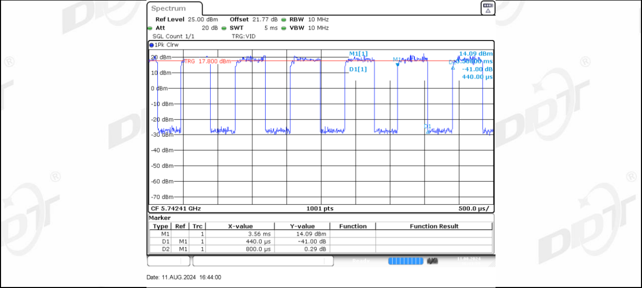
11AX40MIMO_Ant-1_5755_106Tone_RU56
