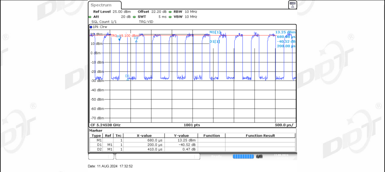
11AX40MIMO_Ant-3_5230_242Tone_RU61
