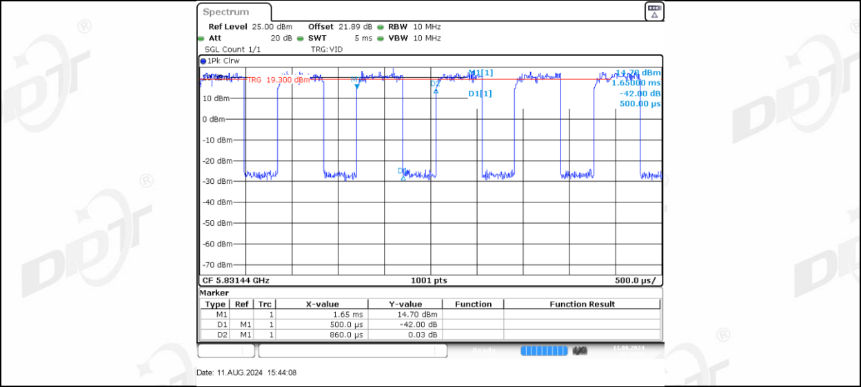
11AX20MIMO_Ant-3_5825_106Tone_RU53
