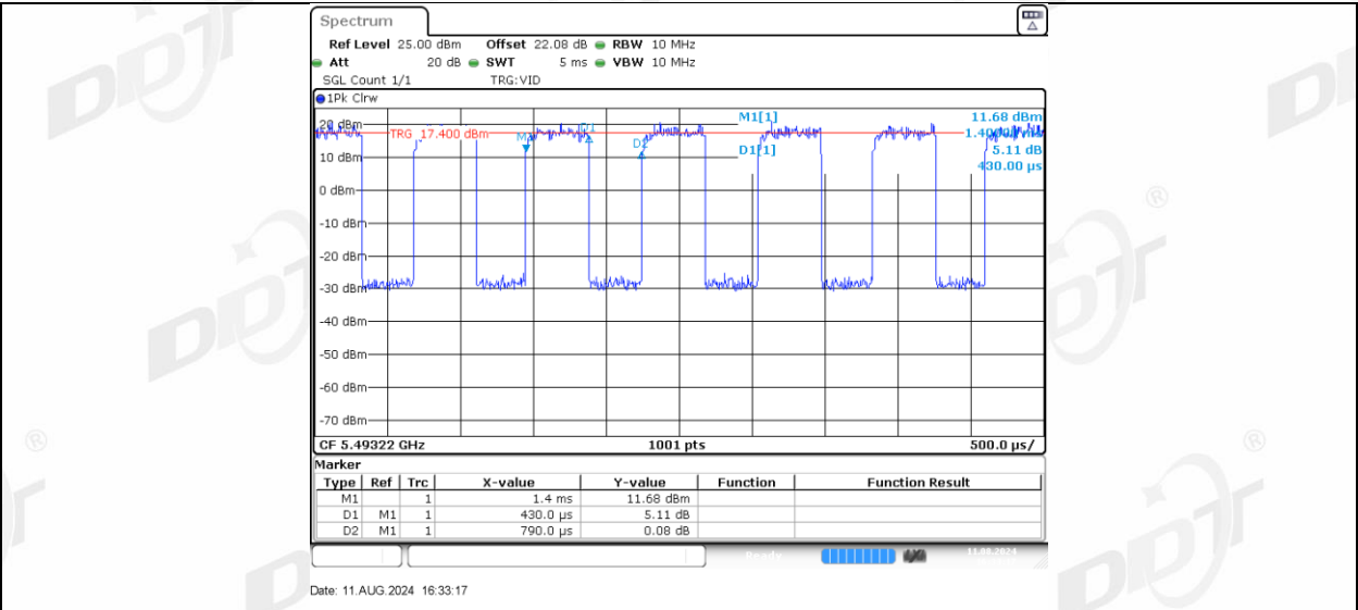
11AX40MIMO_Ant-1_5510_106Tone_RU56
