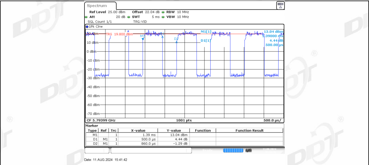
11AX20MIMO_Ant-3_5785_106Tone_RU53
