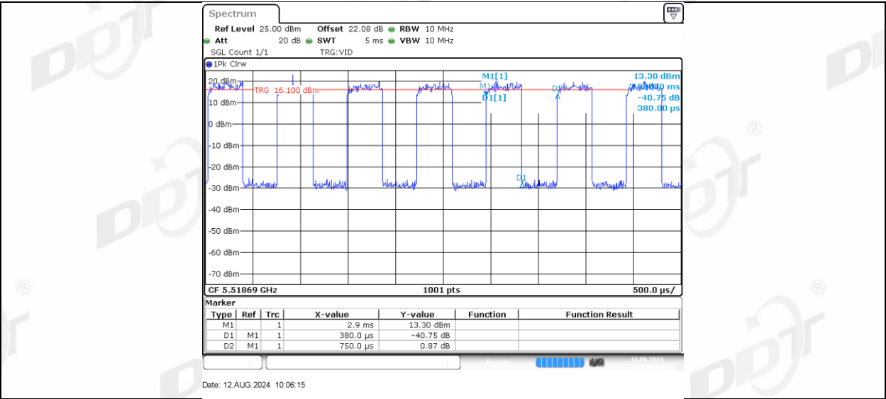
11AX40MIMO_Ant-3_5510_106Tone_RU53
