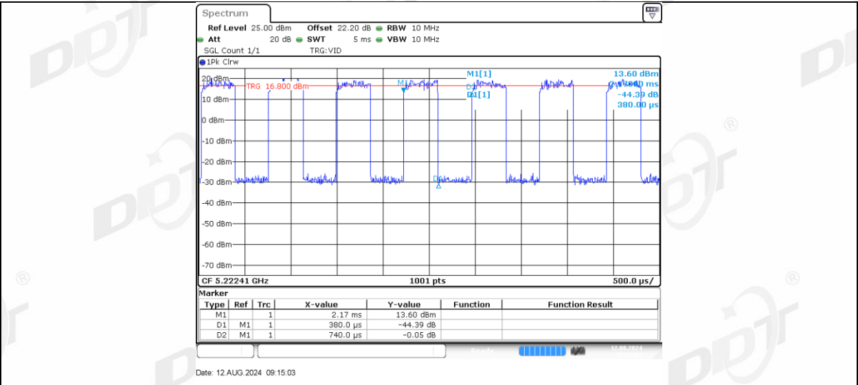
11AX40MIMO_Ant-3_5230_242Tone_RU62
