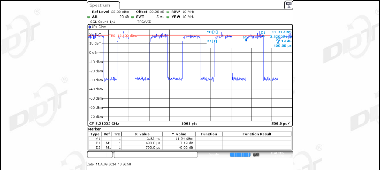
11AX40MIMO_Ant-3_5230_106Tone_RU56
