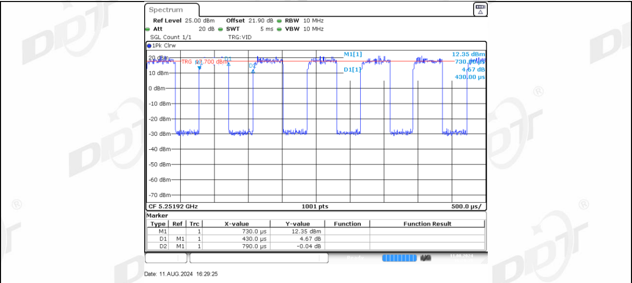
11AX40MIMO_Ant-3_5270_106Tone_RU56
