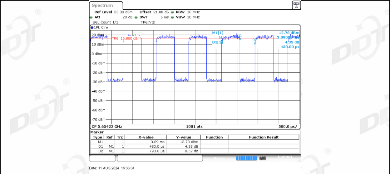
11AX40MIMO_Ant-1_5670_106Tone_RU56
