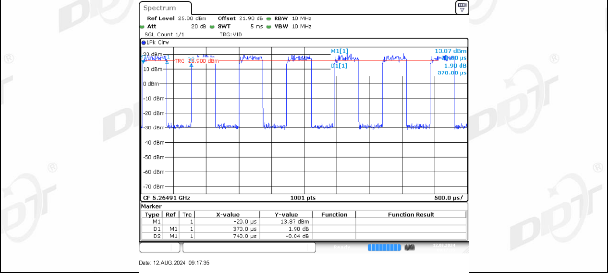
11AX40MIMO_Ant-3_5270_242Tone_RU62
