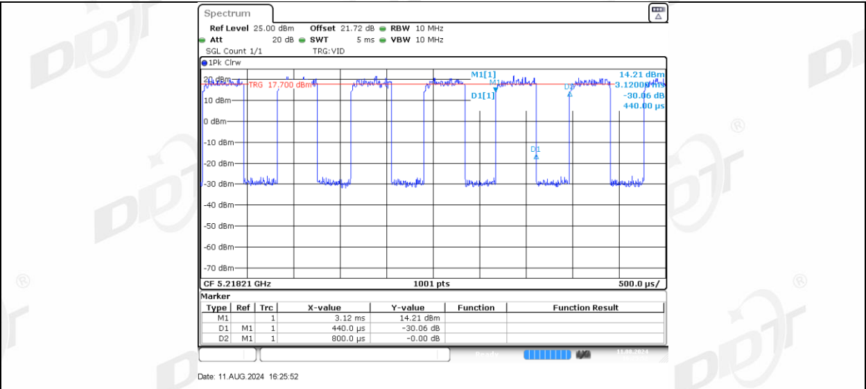
11AX40MIMO_Ant-1_5230_106Tone_RU56
