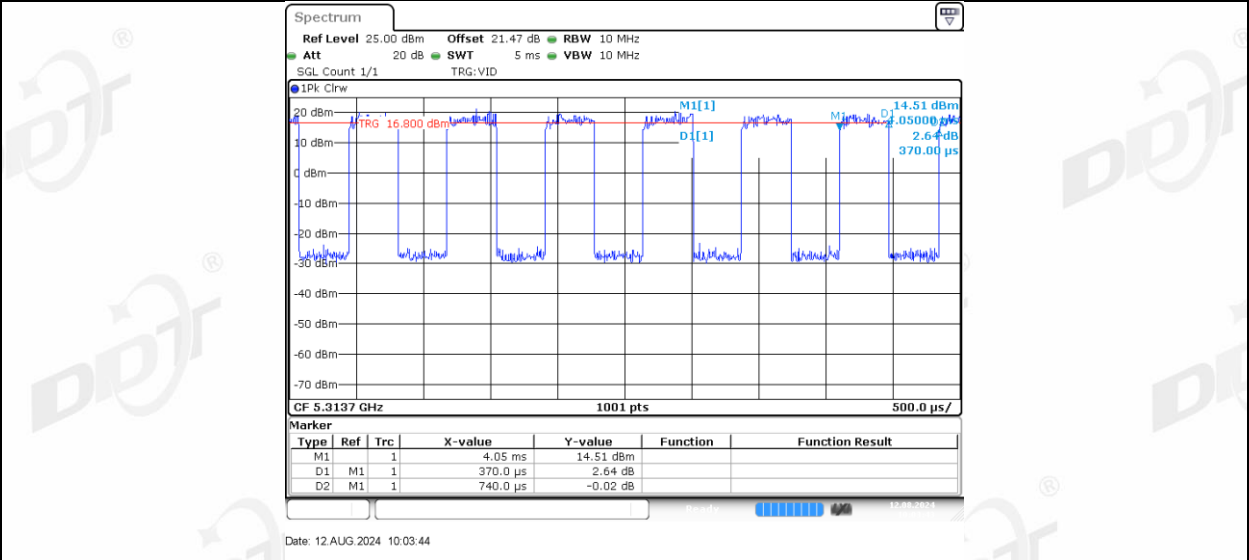
11AX40MIMO_Ant-3_5310_106Tone_RU53
