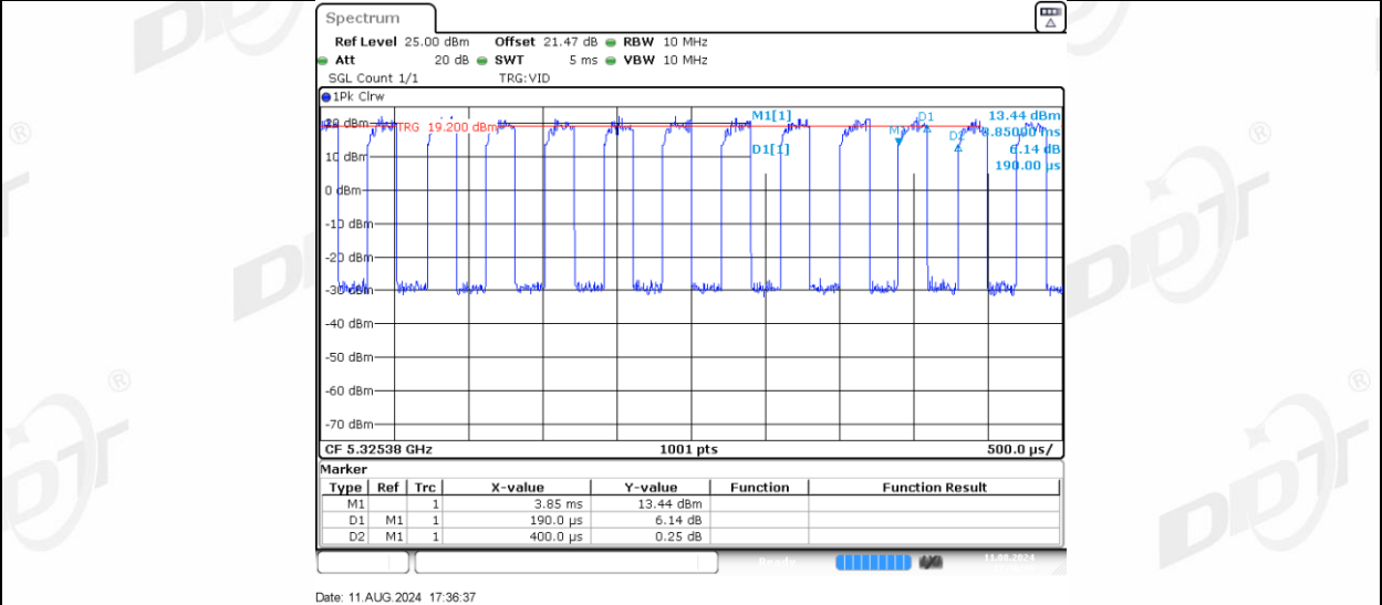
11AX40MIMO_Ant-1_5310_242Tone_RU61
