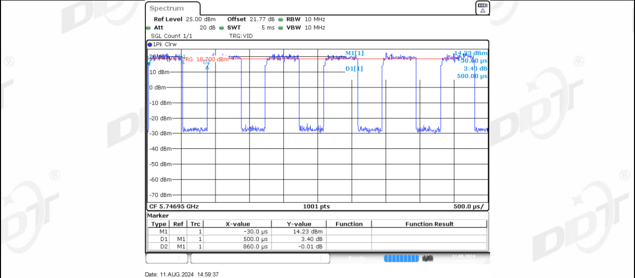
11AX20MIMO_Ant-1_5745_52Tone_RU40
