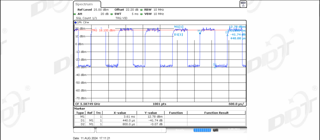
11AX20MIMO_Ant-3_5580_26Tone_RU0
