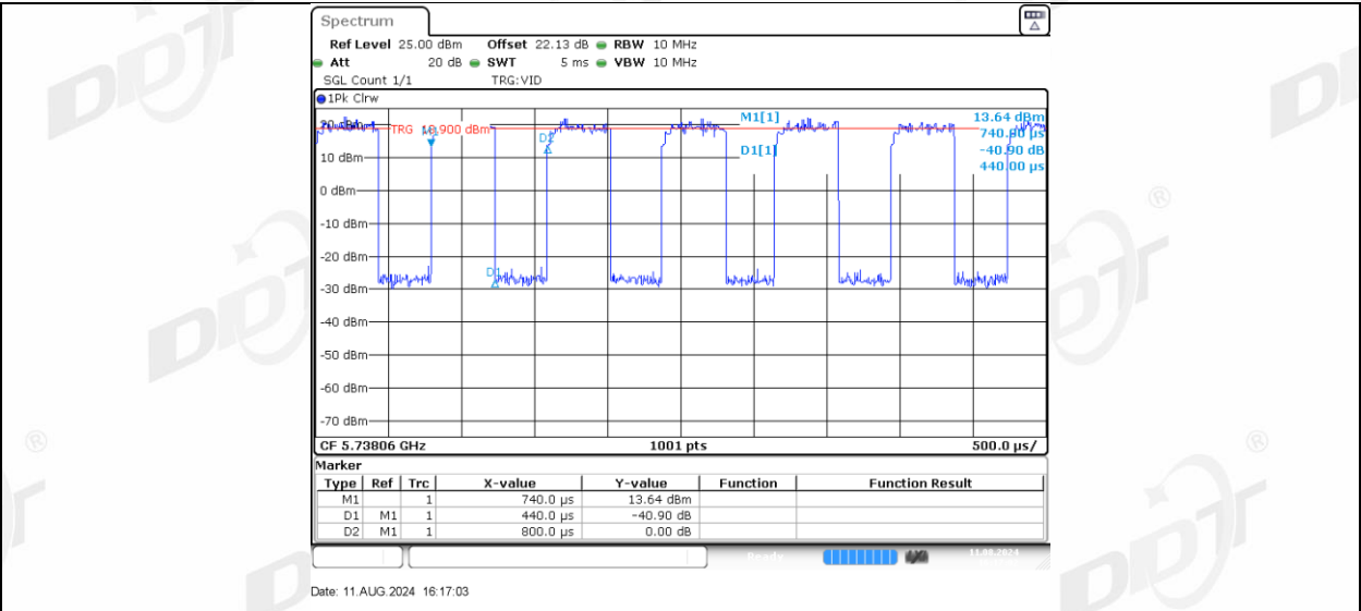
11AX20MIMO Ant-3 5745 106Tone_RU54
