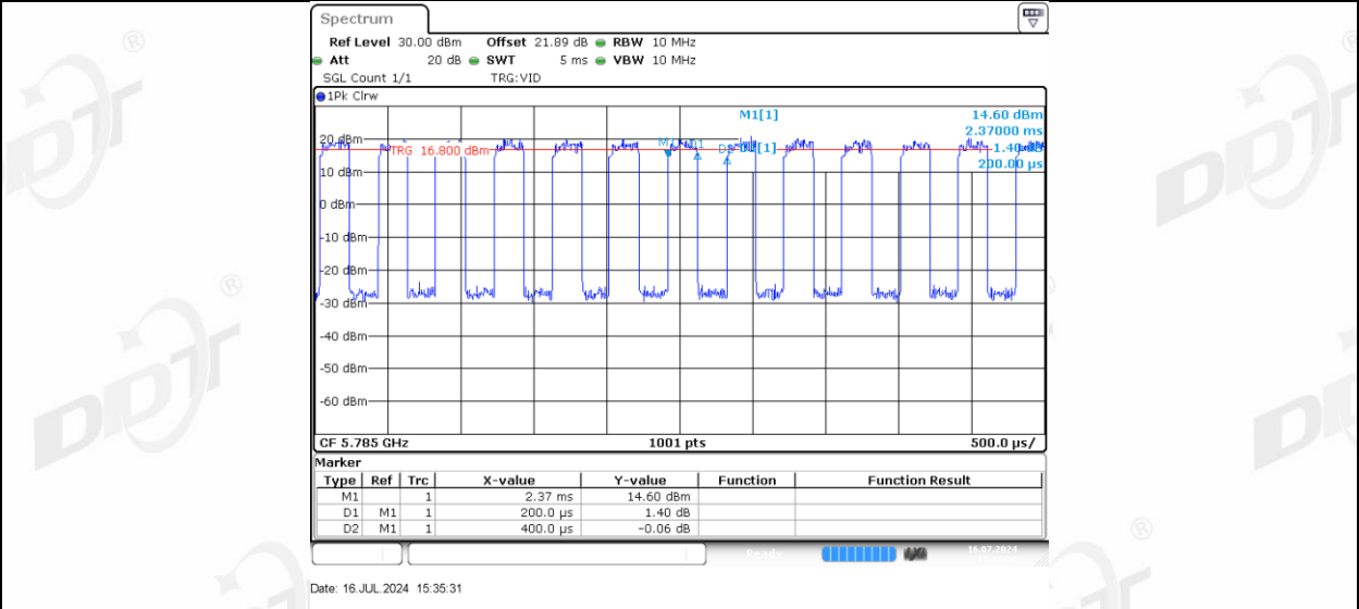
11AX20MIMO_Ant-3_5785
