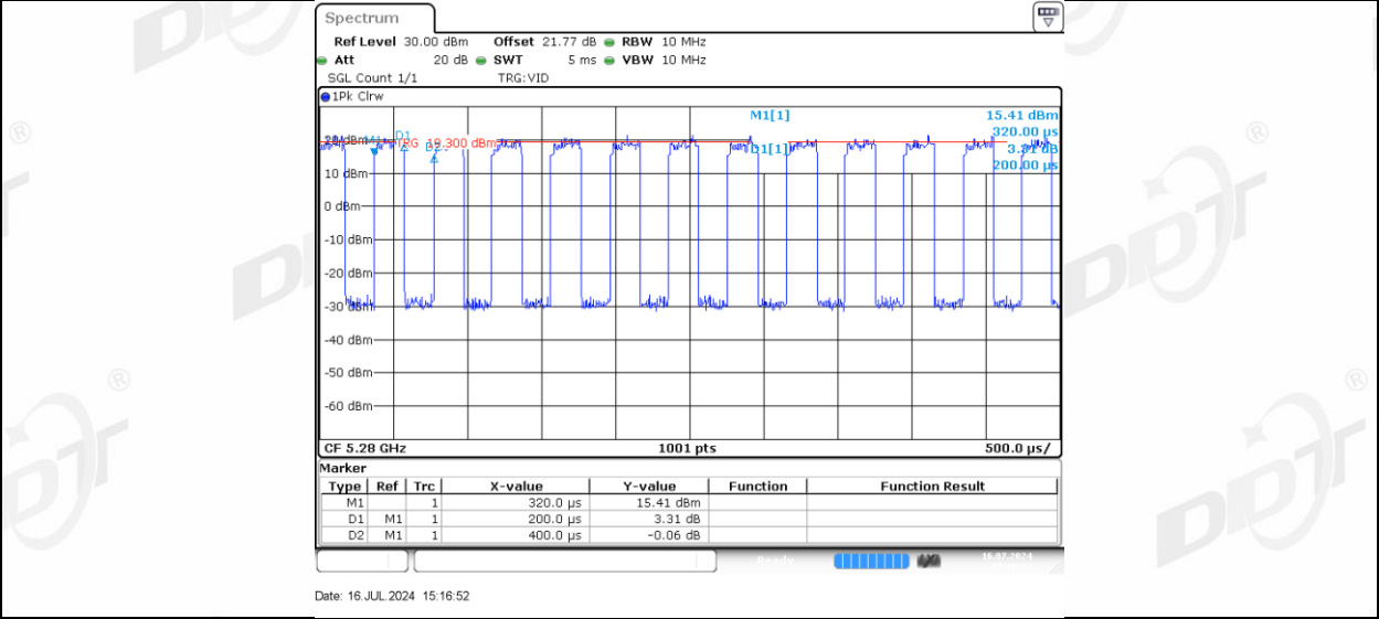
11AX20MIMO_Ant-3_5280
