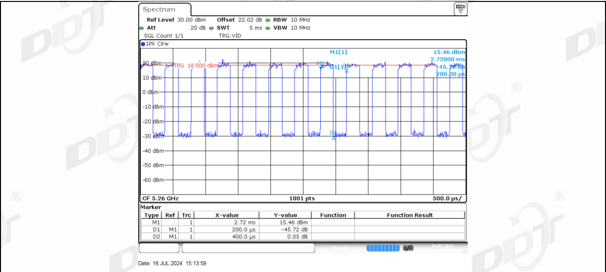
11AX20MIMO_Ant-3_5260
