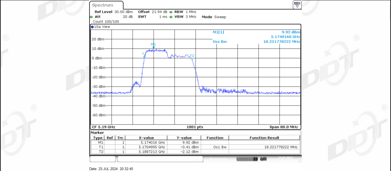
11AX40MIMO_Ant-3_5190_106Tone_RU56
