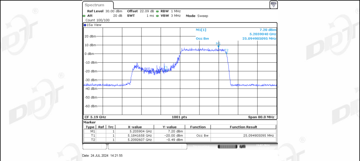
11AX40MIMO_Ant-3_5190_106Tone_RU53
