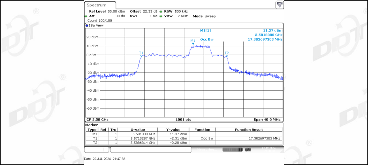
11AX20MIMO_Ant-3_5580_52Tone_RU40
