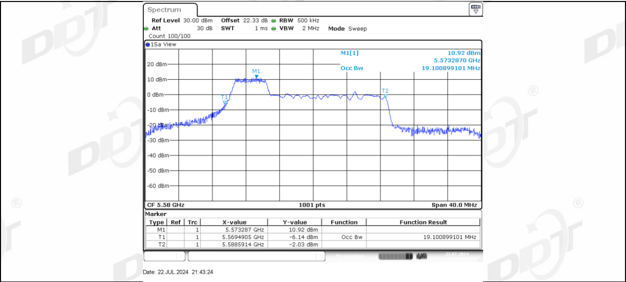
11AX20MIMO_Ant-3_5580_52Tone_RU39
