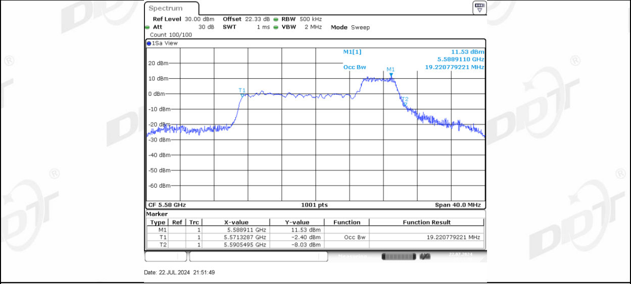
11AX20MIMO_Ant-3_5580_106Tone_RU53
