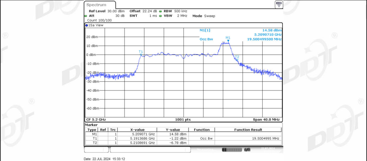
11AX20MIMO Ant-3 5200_52Tone_RU37
