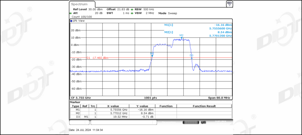
11AX40MIMO_Ant-3_5755_242Tone_RU61
