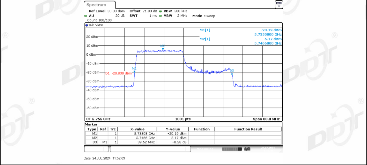
11AX40MIMO_Ant-3_5755_242Tone_RU62
