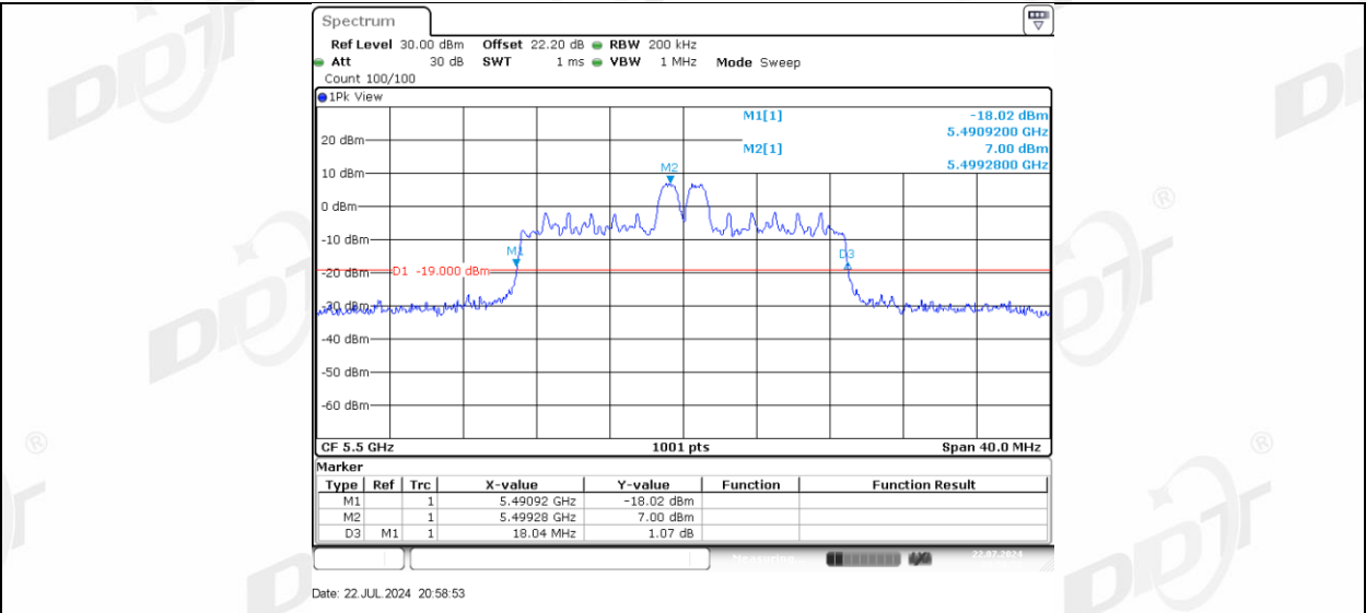
11AX20MIMO Ant-3 5500_26Tone_RU8
