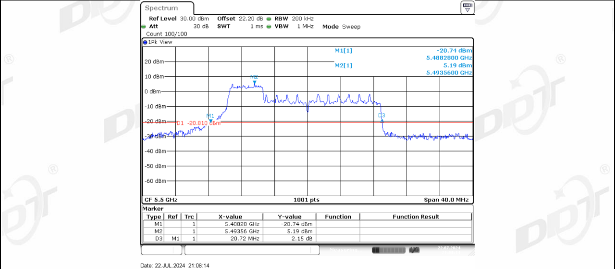
11AX20MIMO Ant-3 5500_52Tone_RU39
