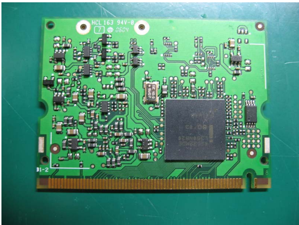
Wireless LAN Module back side
