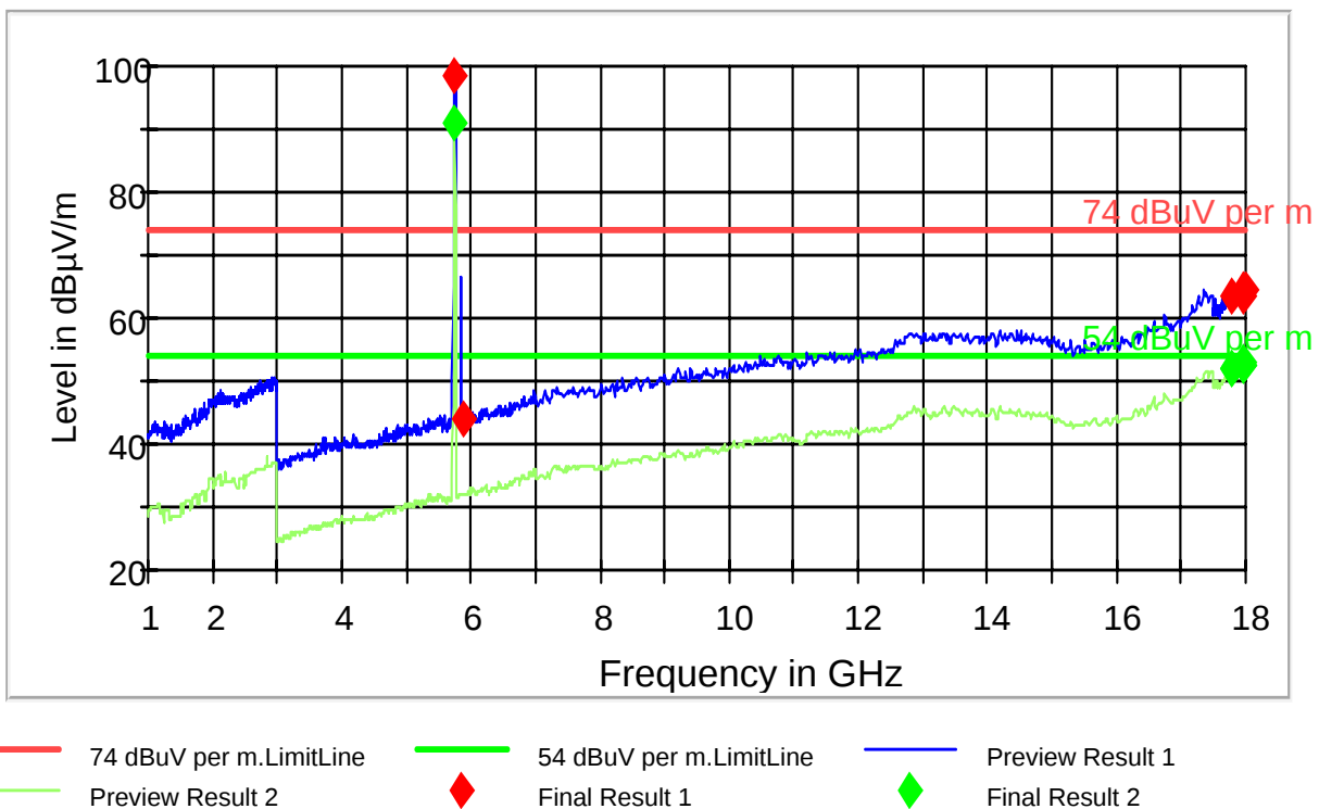
FCC 15 1-18GHz
