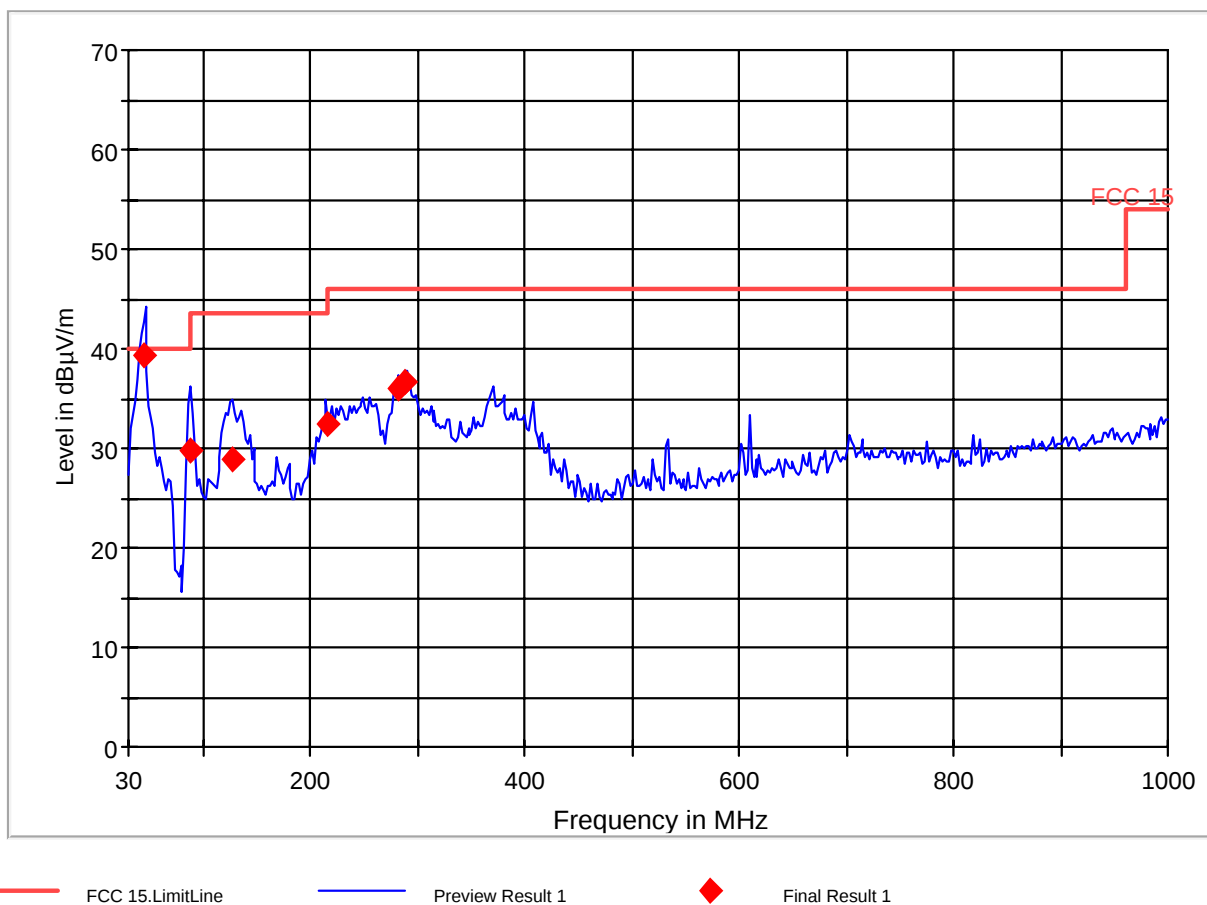
FCC 15 30-1000MHz
