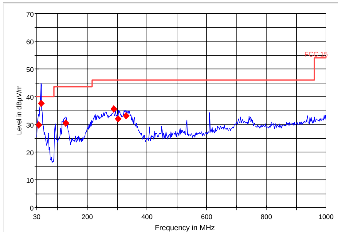
FCC 15 30-1000MHz
