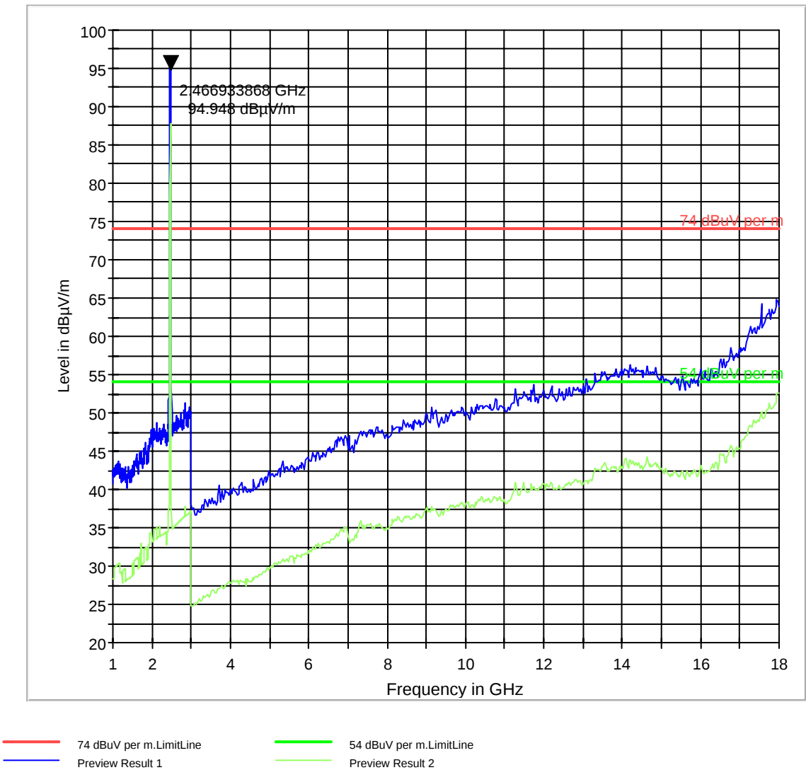
FCC 15 1-18GHz
