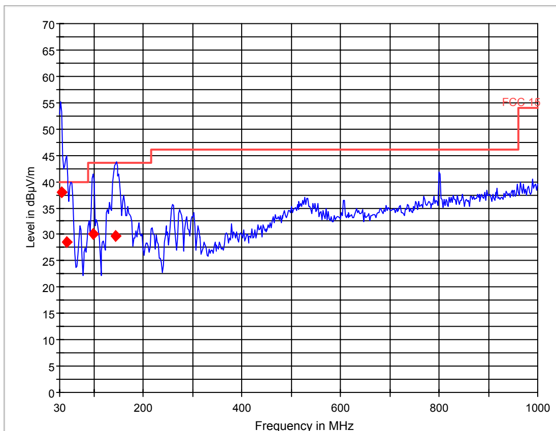
FCC 15 30-1000MHz
