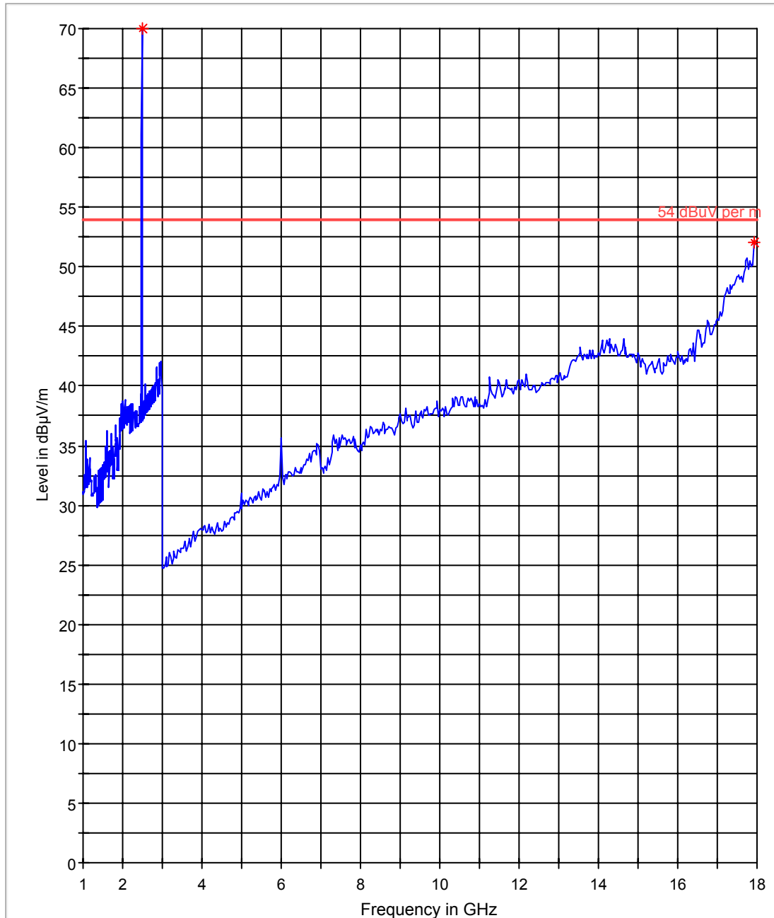
FCC 15 1-18GHz
