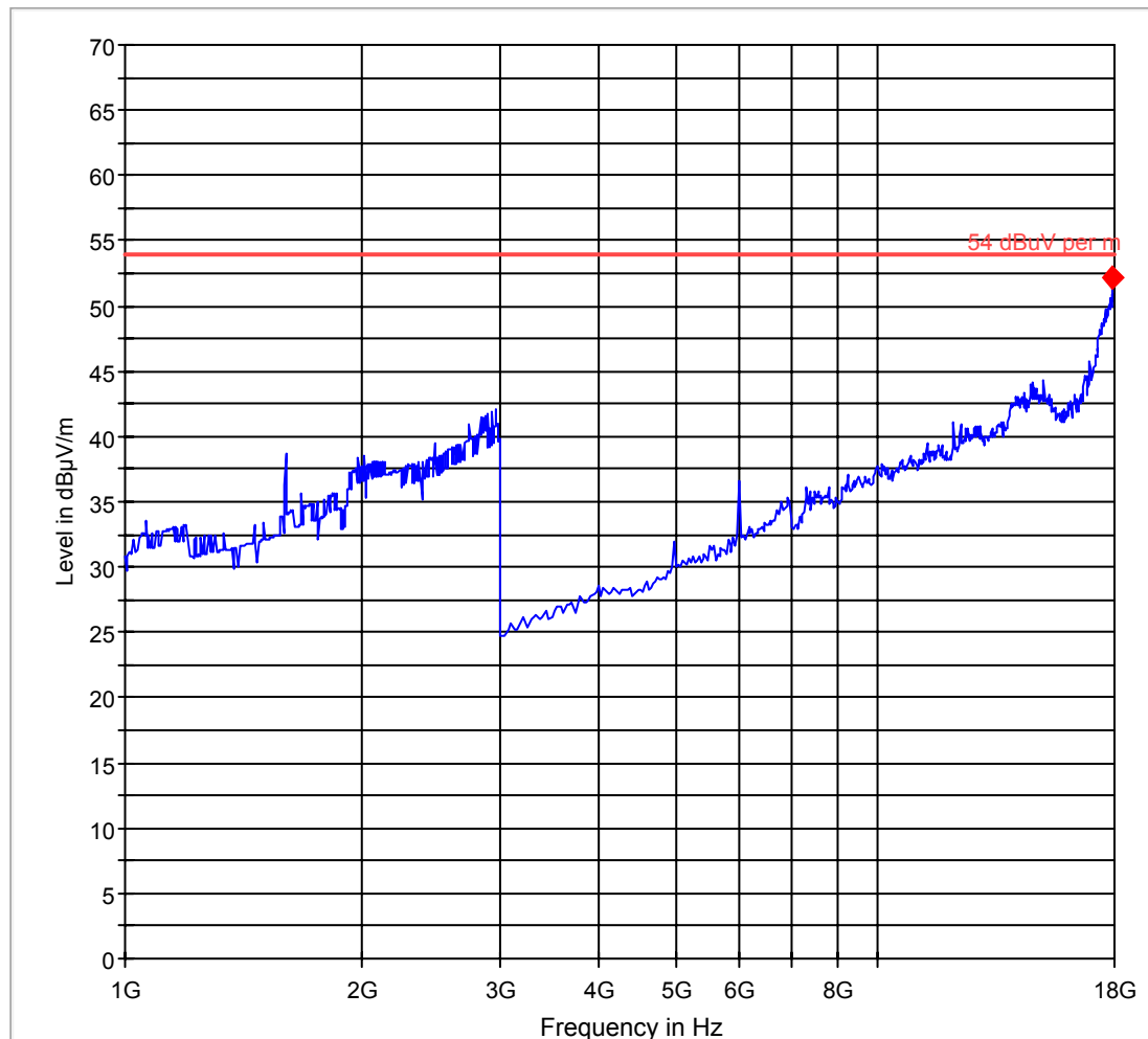
FCC 15 1-18GHz
