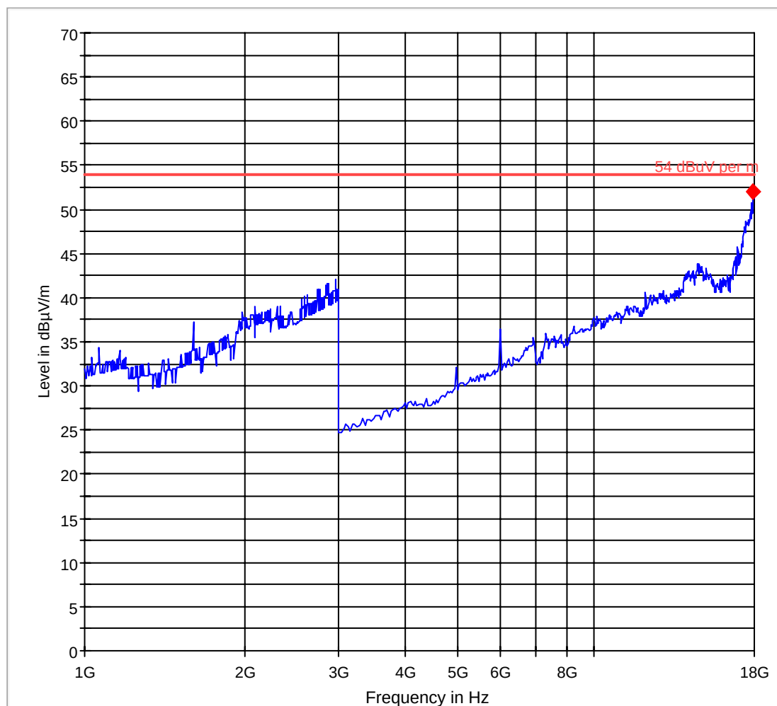
FCC 15 1-18GHz
