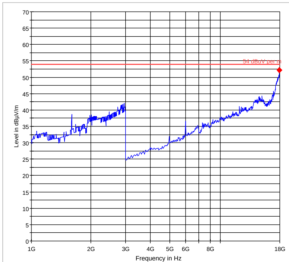
FCC 15 1-18GHz
