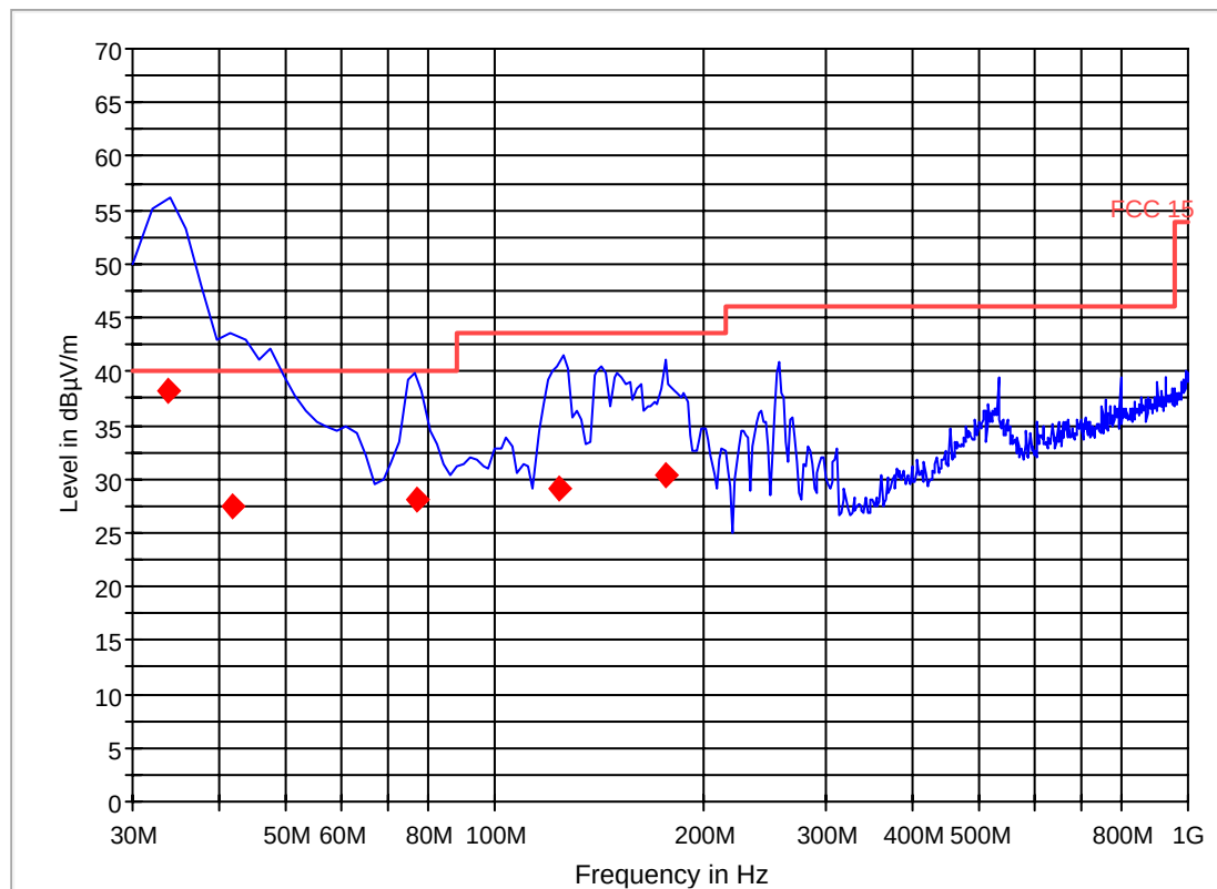
FCC 15 30-1000MHz
