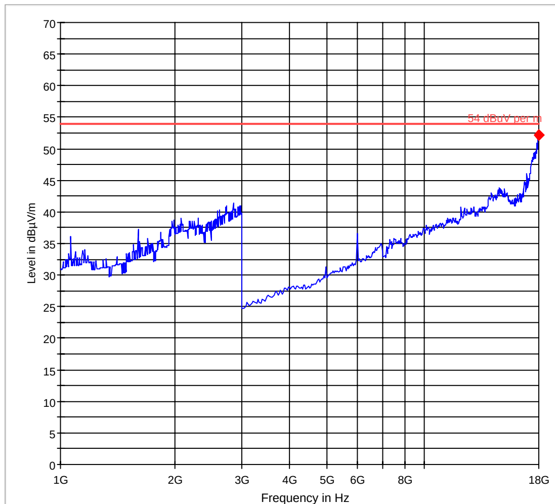
FCC 15 1-18GHz
