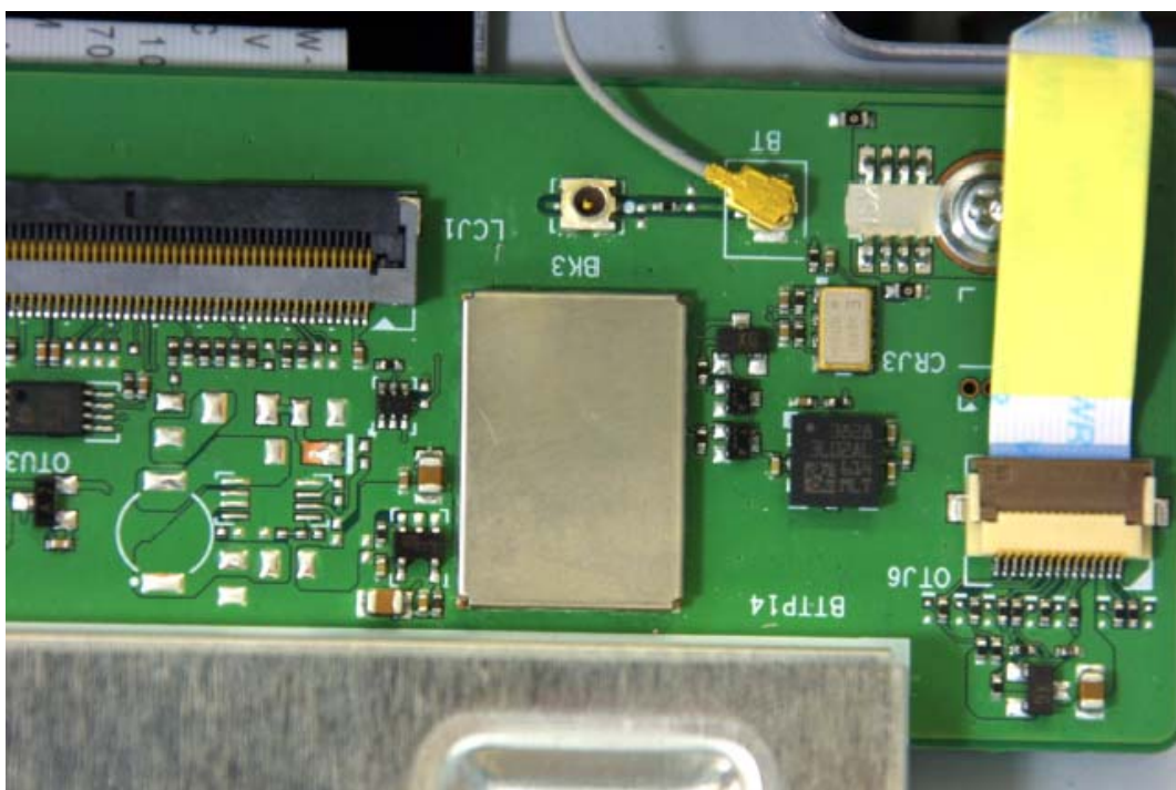
BT Module Close up
