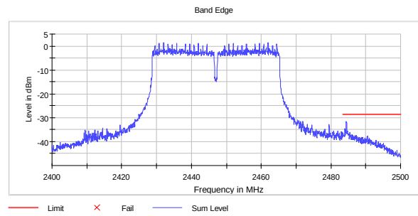
Band Edge Ch08 802.11n HT40 MCS15 MIMO
