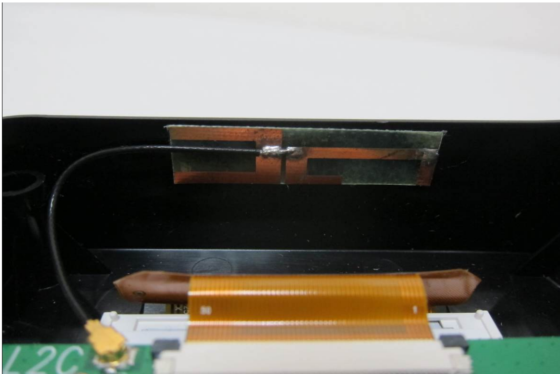
EUT-6. WLAN Antenna B
