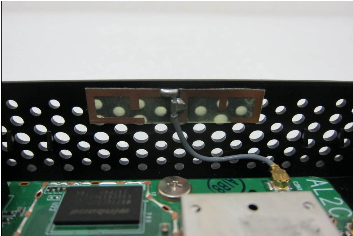
EUT-5. WLAN Antenna A
