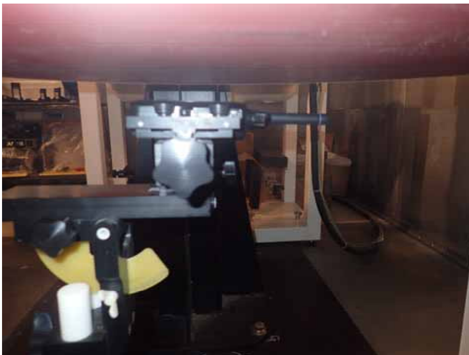
< FA-SC27VS Antenna >
