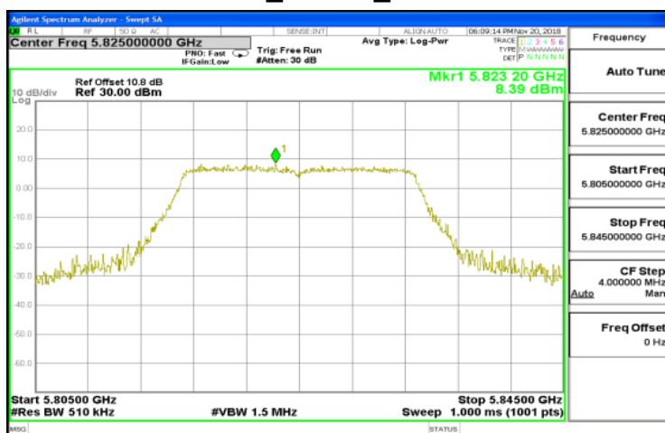
802.11n_20MHz_5825MHz
